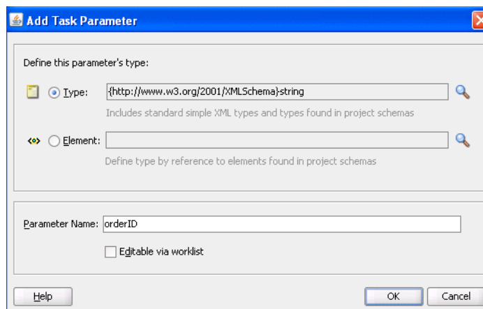
Figure 29–14 Add Task Parameter Dialog
