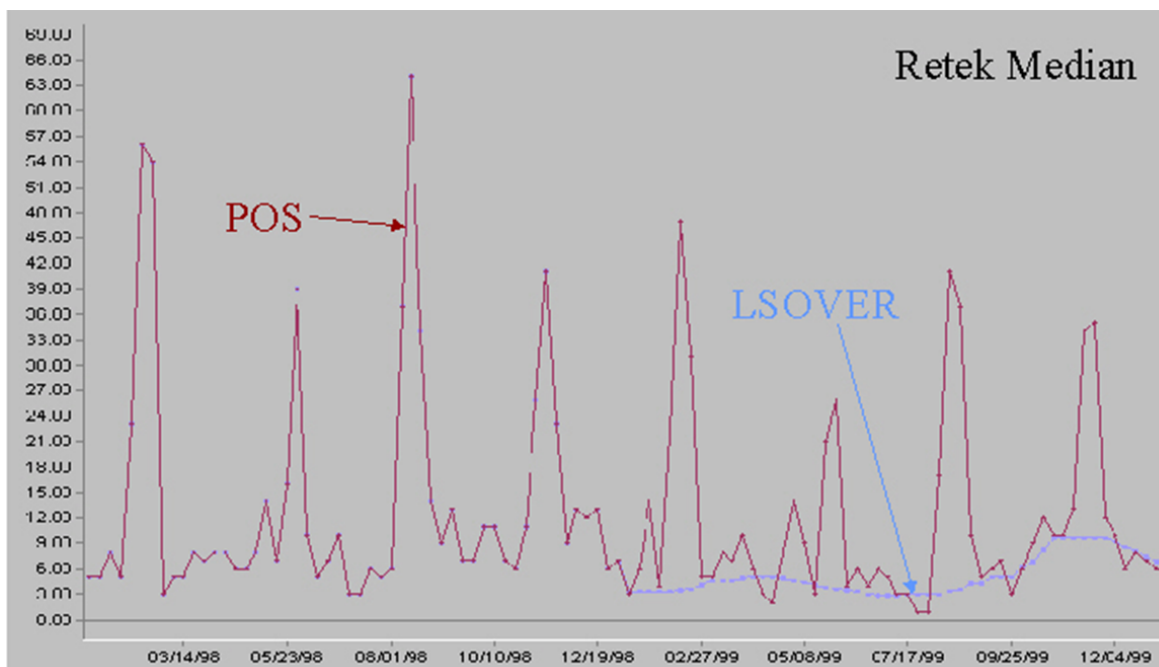
Example C–6 Retek Median with Default Parameters
