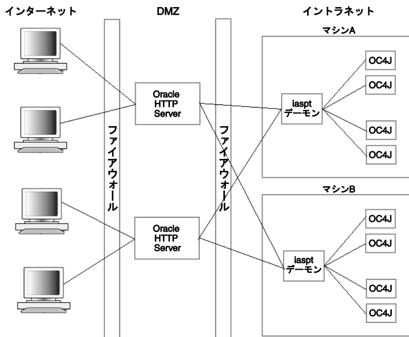
図 9-2 ポート・トンネリング
