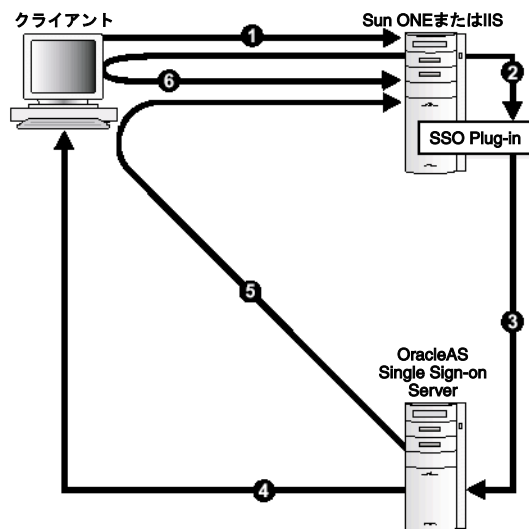
図 B-1 OracleAS SSO Plug-in
