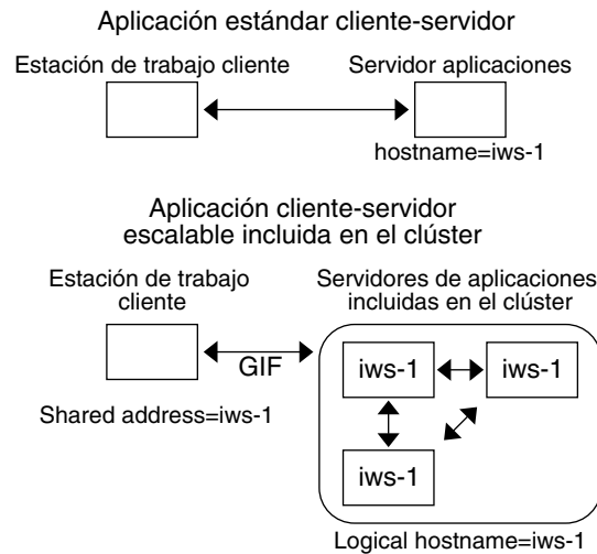
FIGURA 3-5 Comparación entre los nombres de sistema fijos y las direcciones compartidas
