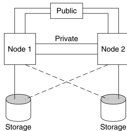
FIGURA 2-6 x86: Topología de par en clúster
