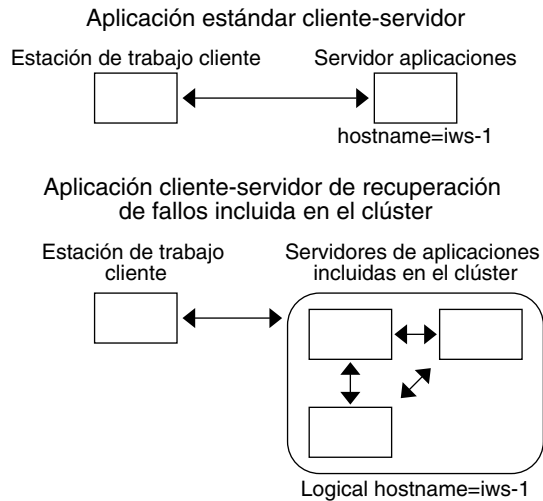
FIGURA 3-4 Comparación entre los nombres de sistema fijo y lógico
