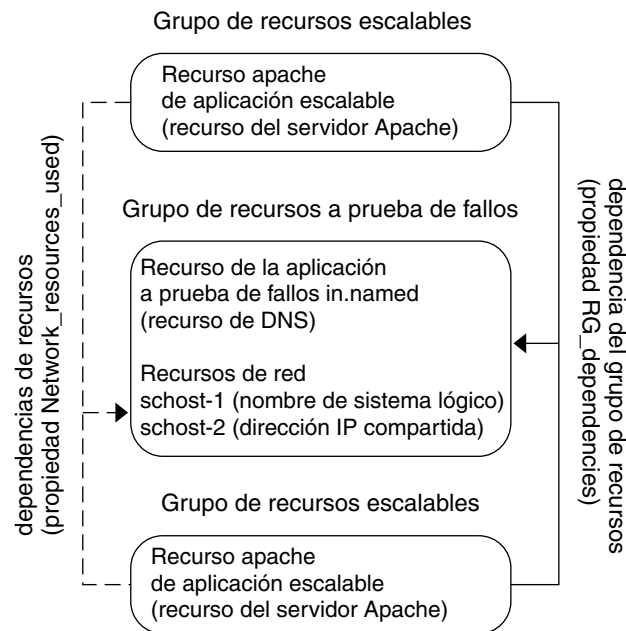
FIGURA 3-6 SPARC: Ejemplo de los grupos de recursos a prueba de fallos y escalables
