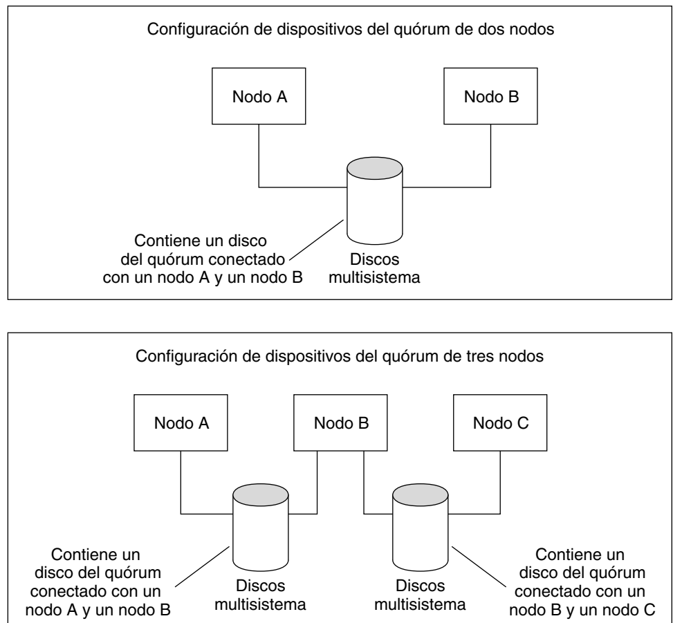
FIGURA 3-2 Ejemplos de configuraciones de los dispositivos del quórum
