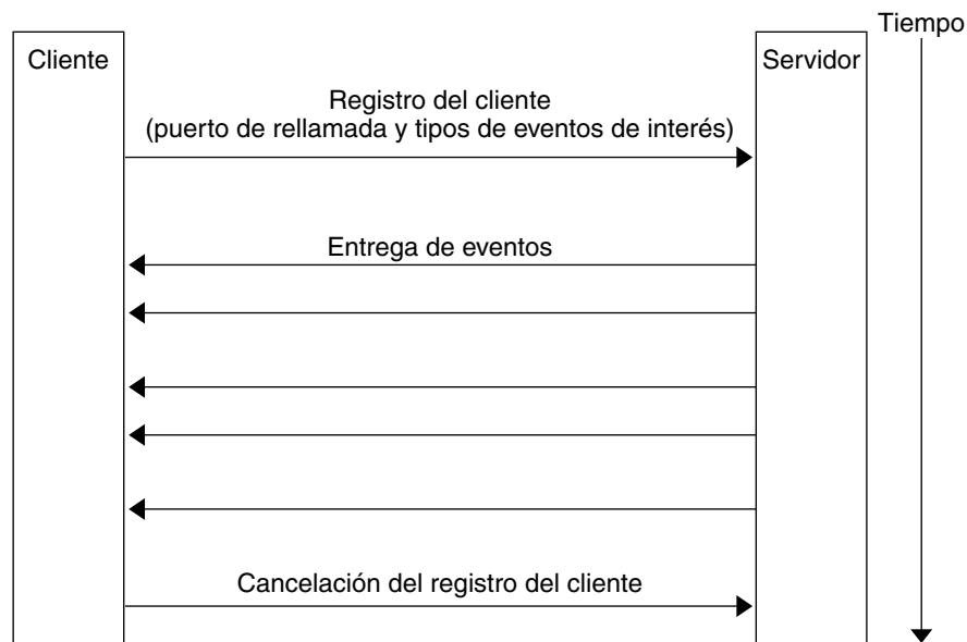
FIGURA 12–2 Flujo de comunicación entre un cliente y un servidor
