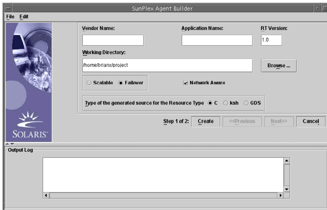
FIGURA 9-1 Pantalla de creación
