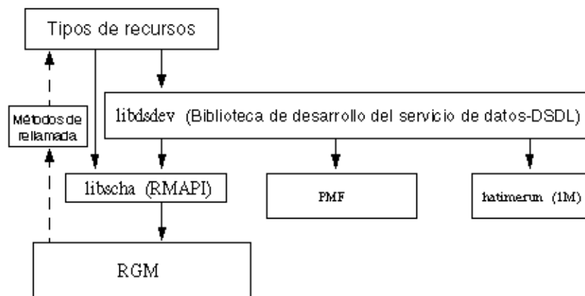
FIGURA 1-1 Arquitectura de programación
