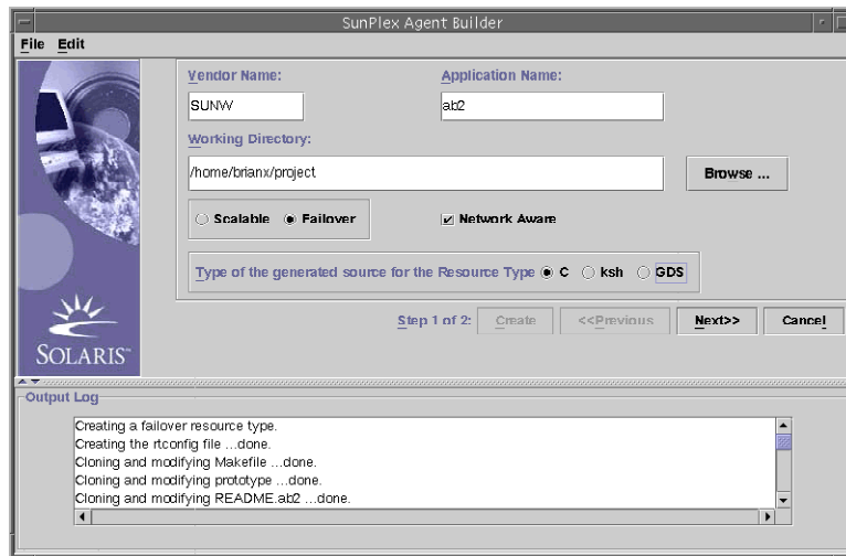
FIGURA 9-4 Pantalla de creación del software Agent Builder
