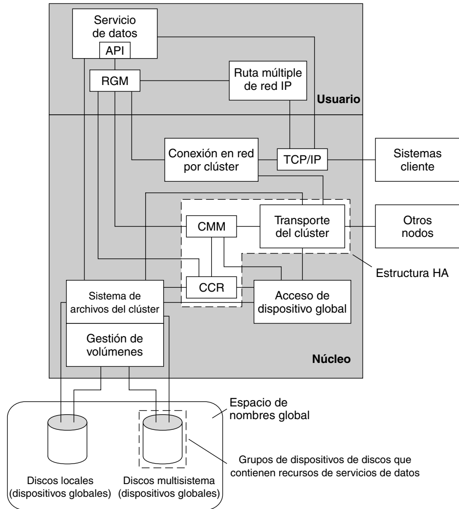
FIGURA 3-2 Arquitectura del software de Sun Cluster
