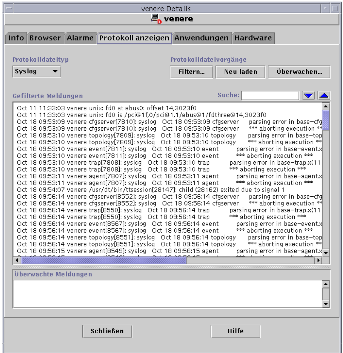
ABBILDUNG 14-3 Das Register "Protokoll anzeigen"
