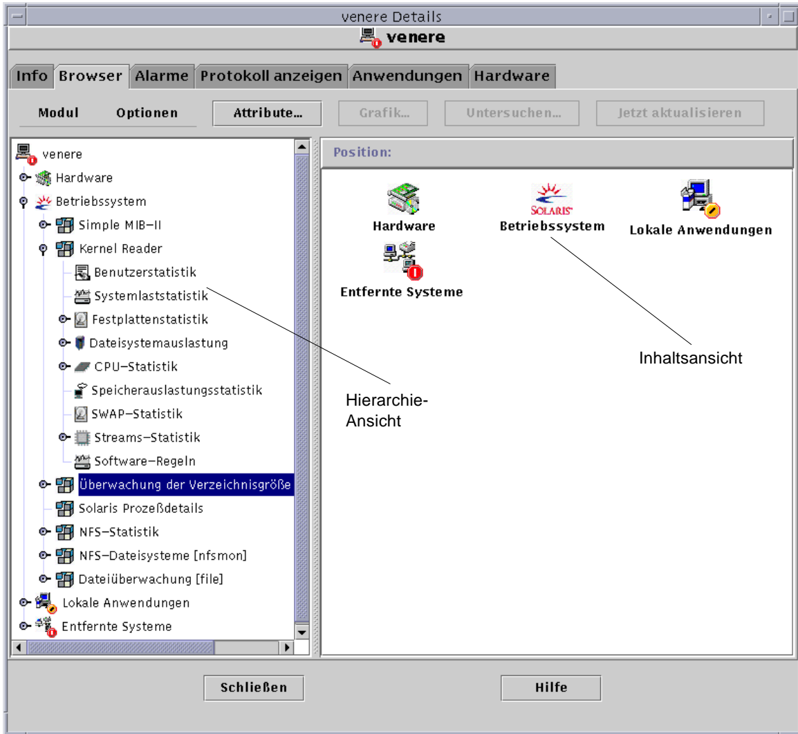
ABBILDUNG 8-3 Das Detailangabenfenster des Suchdienstes
