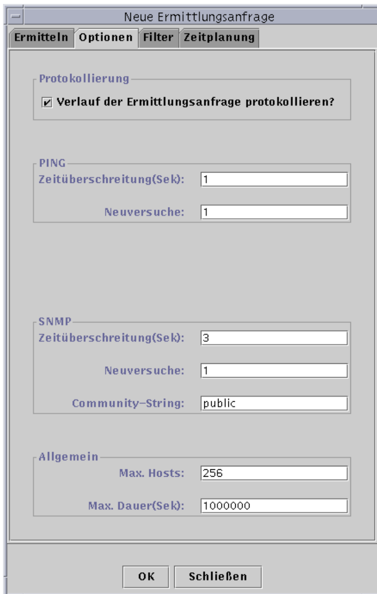
ABBILDUNG 6-4 Das Register "Optionen" im Fenster "Neue Ermittlungsanfrage"
