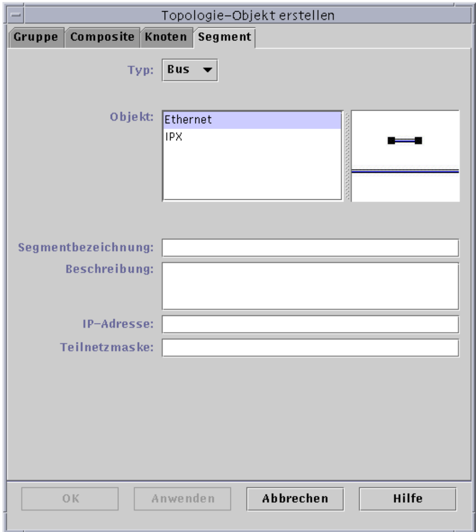
ABBILDUNG 5-7 Das Register "Segment" im Fenster "Topologie-Objekt erstellen"
