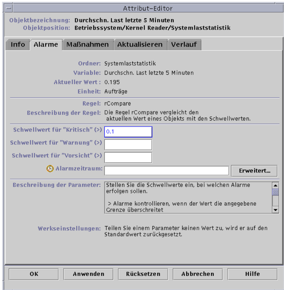
ABBILDUNG 10-3 Das Register “Alarmer” im Attribut-Editor für eine überwachte Eigenschaft
