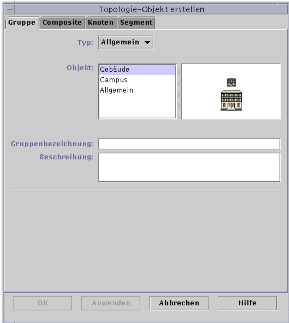
ABBILDUNG 5-5 Erstellen einer Gruppe im Fenster “Topologie-Objekt erstellen”
