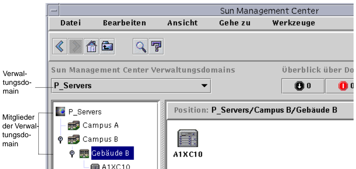
ABBILDUNG 1-4 Darstellung einer Verwaltungsdomain und deren Mitglieder im Sun Management Center Hauptkonsolenfenster
