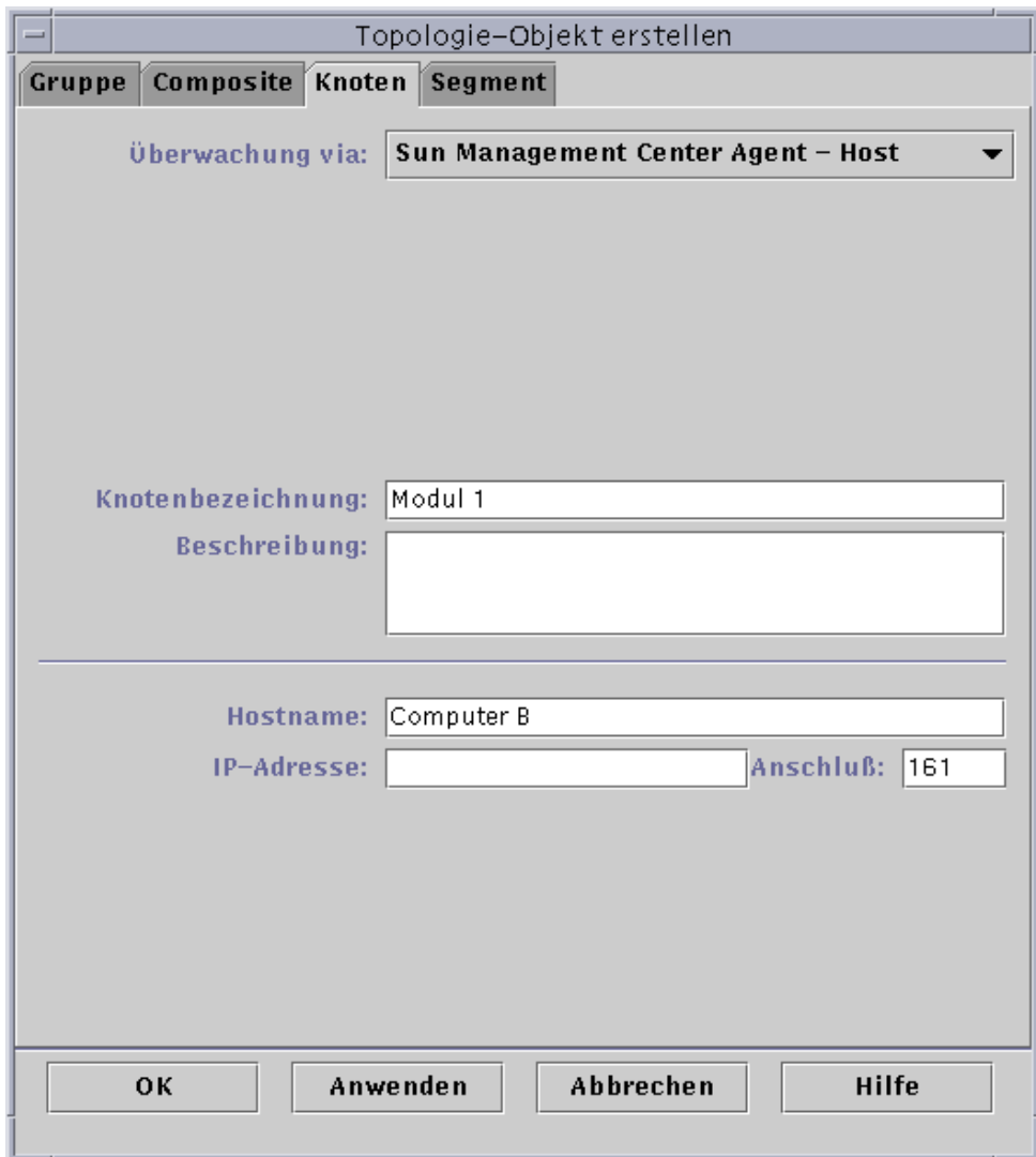
ABBILDUNG 5-2 Das Fenster “Topologie-Objekt erstellen” für “Sun Management Center Agent - Modul”
