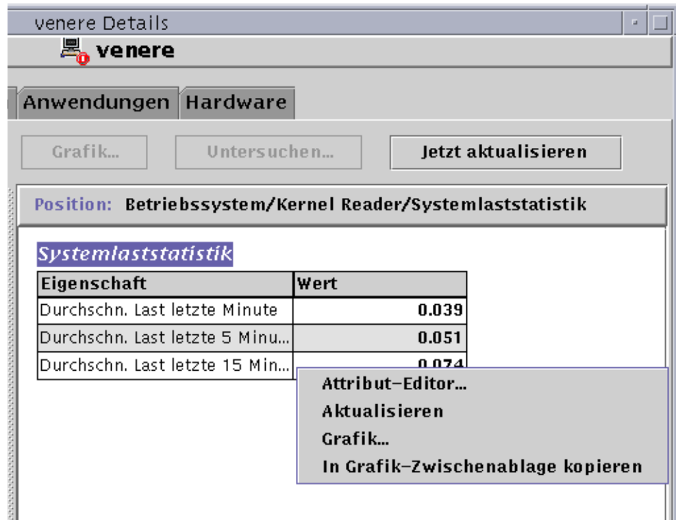
ABBILDUNG 9-10 Das Popup-Menü für überwachte Dateneigenschaften
