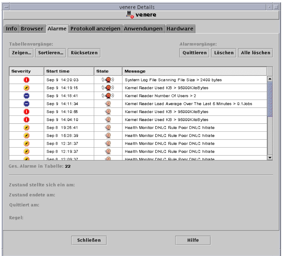
ABBILDUNG 13-10 Daten im Register “Alarme” des Detailfensters
