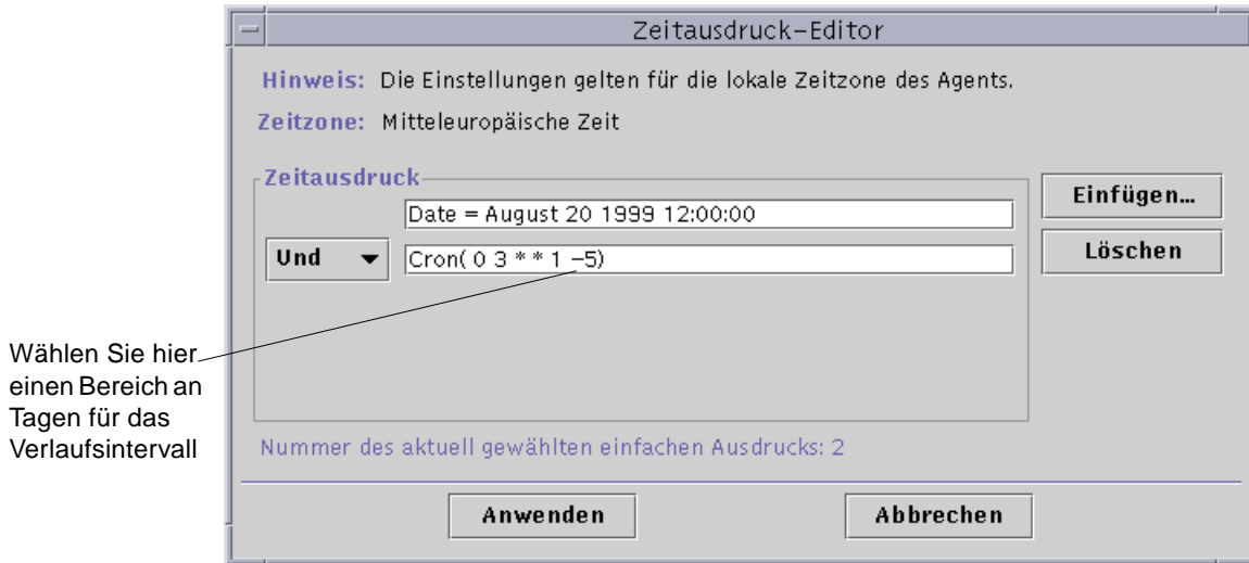
ABBILDUNG 11-13 Der Zeitausdruck-Editor zeigt das Anfangsdatum/die Anfangsuhrzeit 12:00:00 nachm., 20. August 1999 und das Verlaufsintervall 3:00 vorm. jeden Montag bis Freitag
