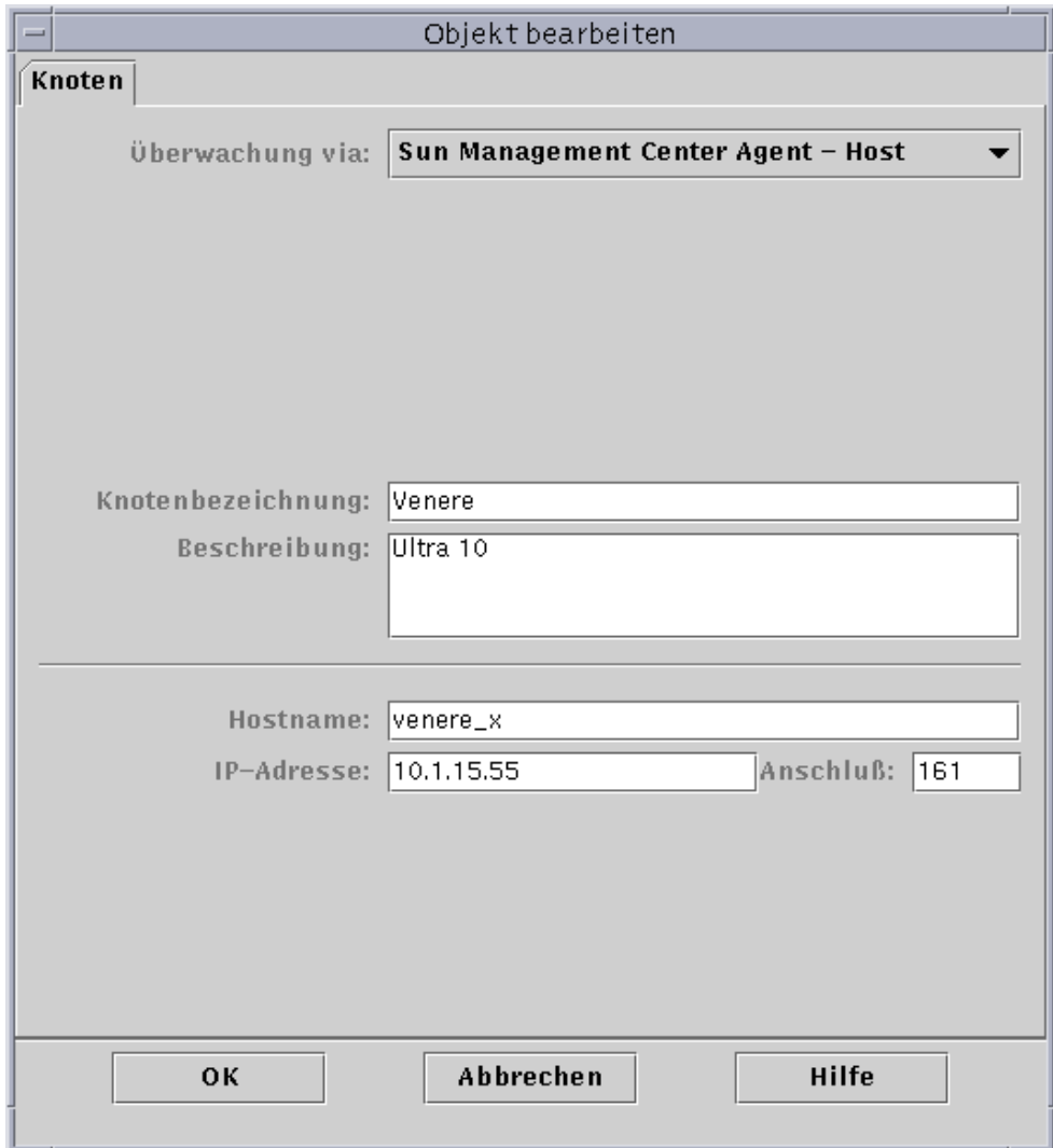
ABBILDUNG 5-8 Das Fenster "Objekt bearbeiten"—Beispiel für Knoten
