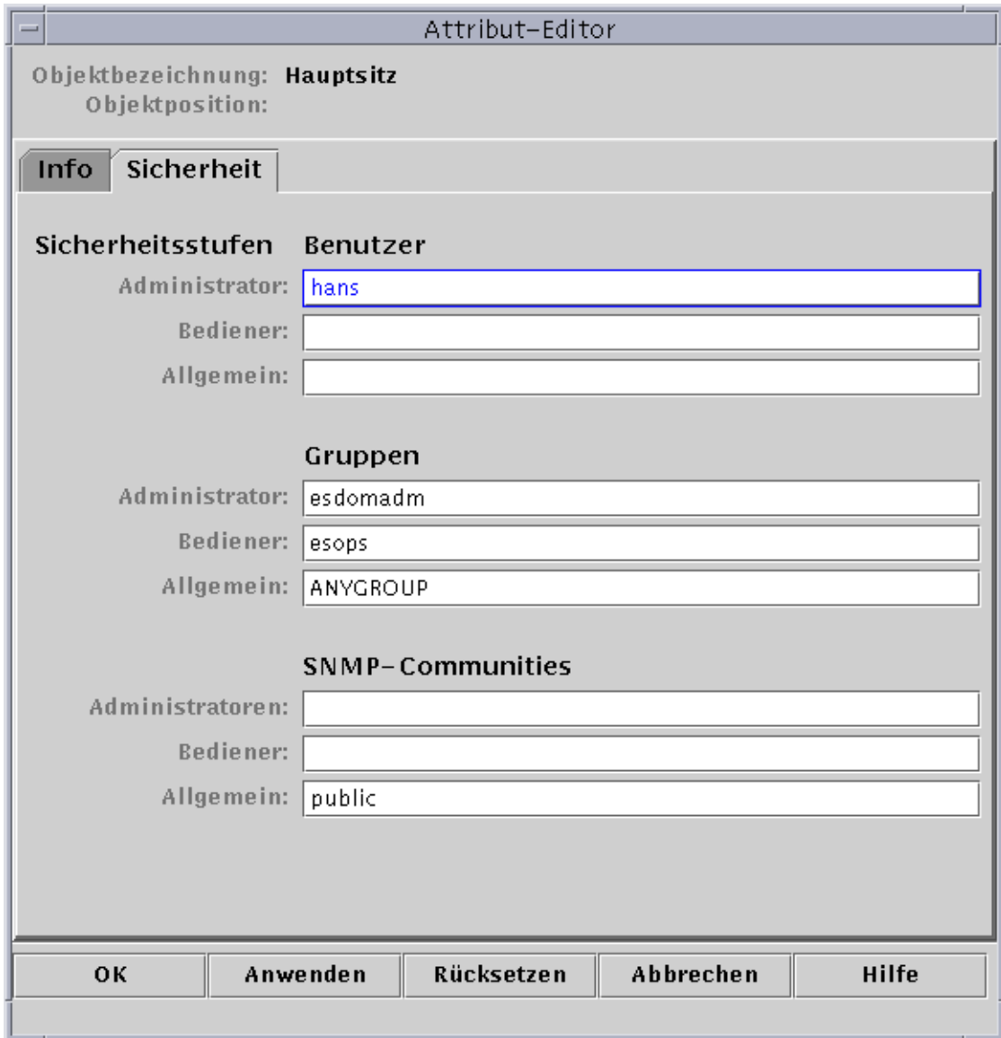
ABBILDUNG 4-16 Attribut-Editor für eine Verwaltungsdomain
