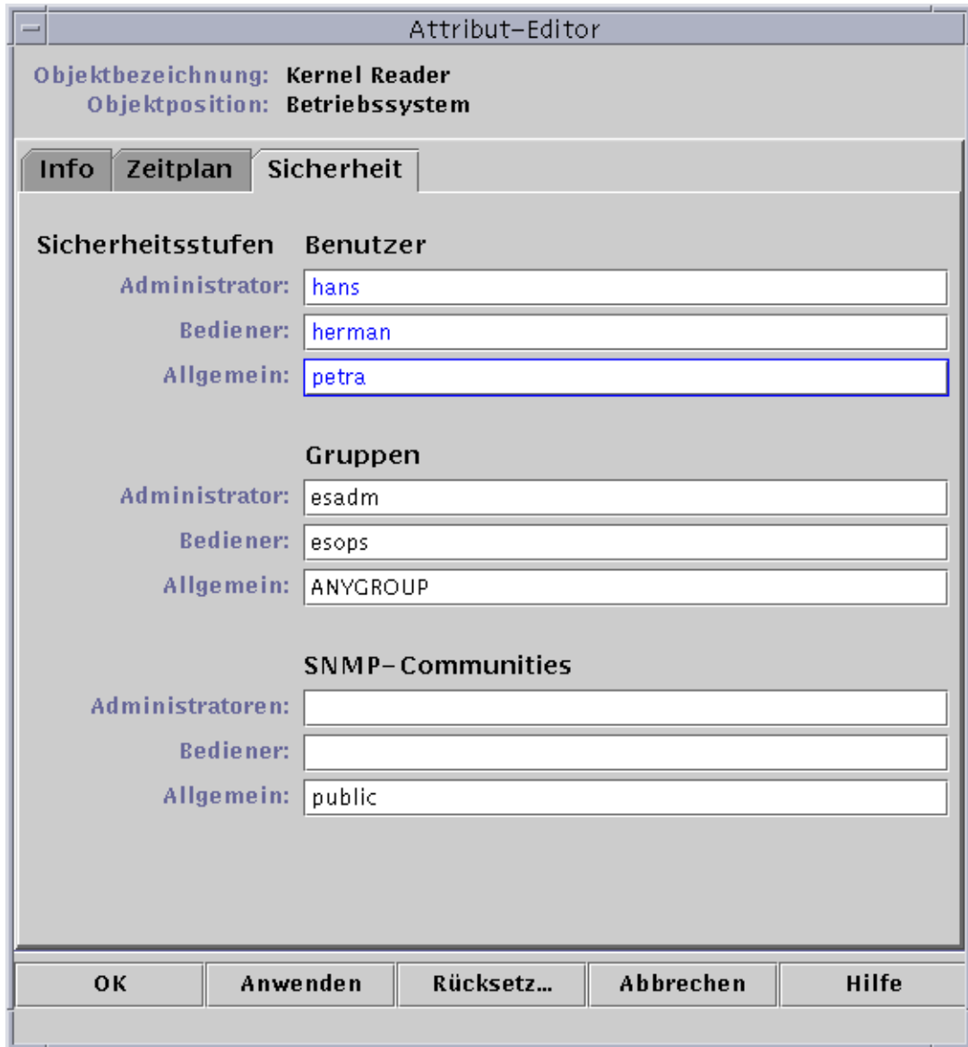
ABBILDUNG 12-15 Einstellen der Modulsicherheit im Attribut-Editor
