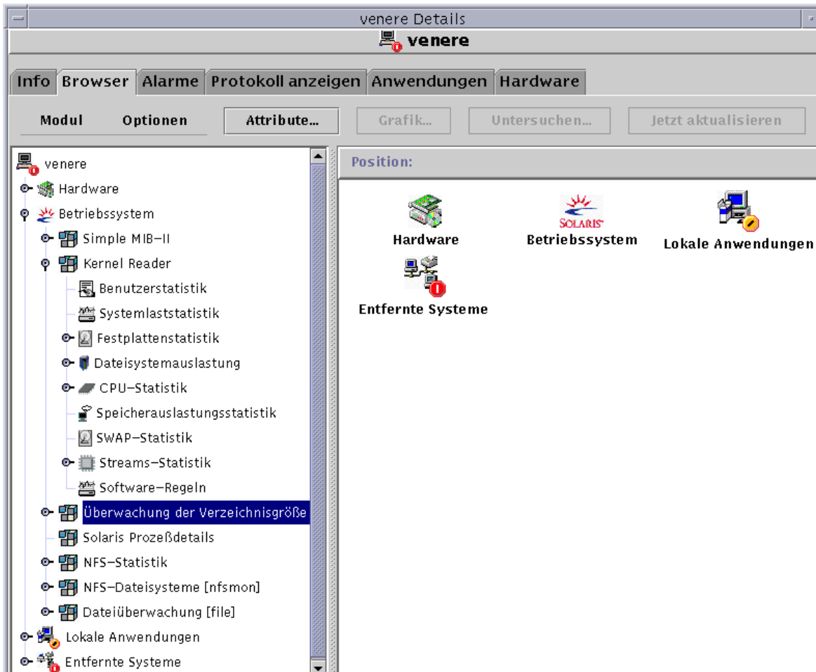
ABBILDUNG 14-1 Detailfenster für ein gewähltes Objekt
