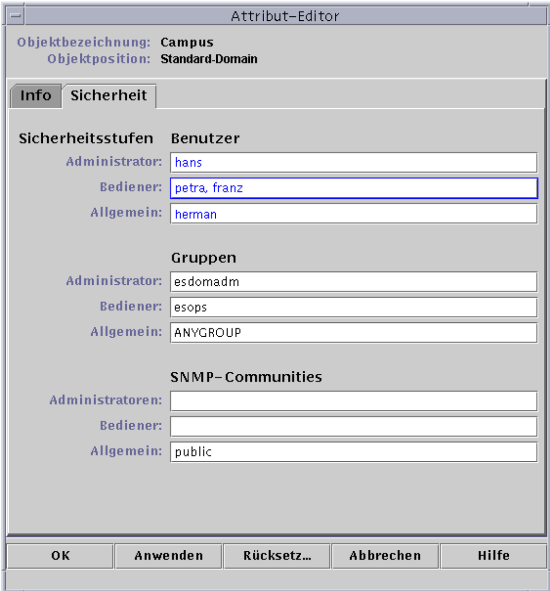
ABBILDUNG 15-2 Beispiel für Sicherheitsfelder im Attribut-Editor
