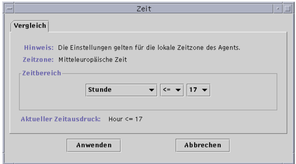
ABBILDUNG 11-17 Das Register "Vergleich" mit der Einstellung kleiner als oder gleich 5 Uhr nachm.
