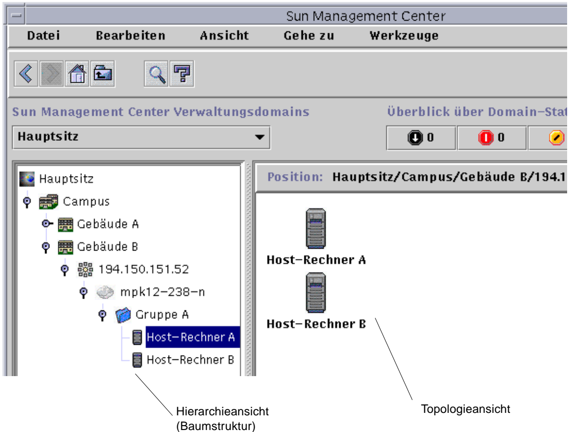
ABBILDUNG 7-2 Hauptkonsolenfenster mit Hierarchie- und Topologieansicht
