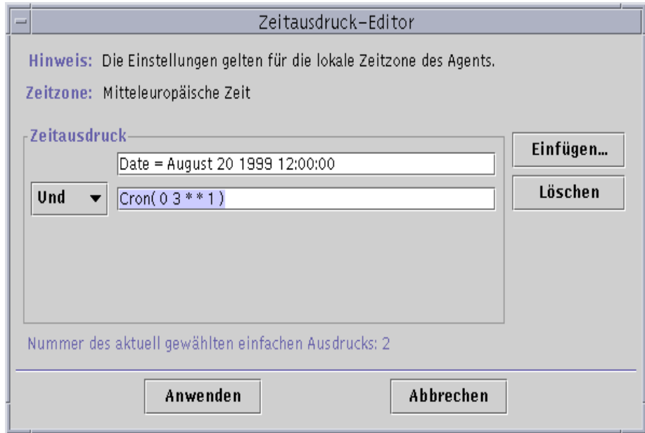
ABBILDUNG 11-12 Der Zeitausdruck-Editor zeigt das Anfangsdatum und die Anfangszeit 12:00:00 nachm., 20. August 1999 und für das Verlaufsintervall die Anfangszeit 3:00 vorm. jeden Montag
