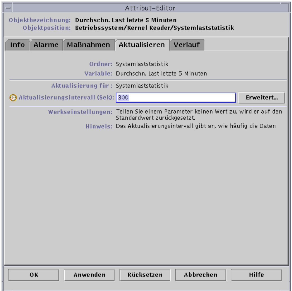
ABBILDUNG 10-6 Das Register “Aktualisieren” im Attribut-Editor für eine überwachte Eigenschaft
