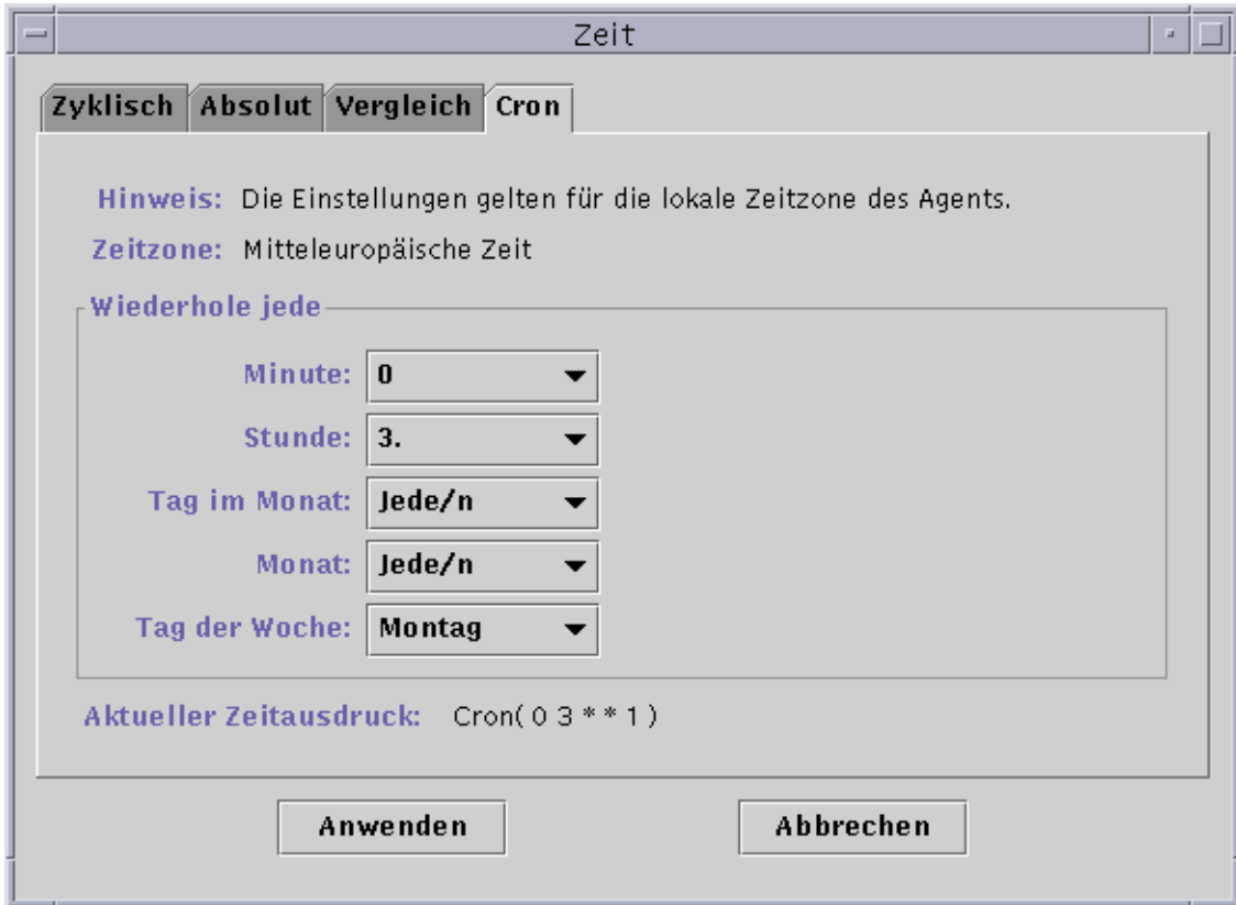
ABBILDUNG 11-11 Das Register "Cron" mit der Auswahl 03.00 Uhr jeden Montag
