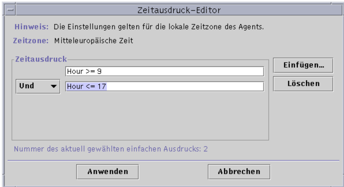
ABBILDUNG 11-18 Der Zeitausdruck-Editor zeigt das Intervall 09.00 bis 17.00 Uhr
