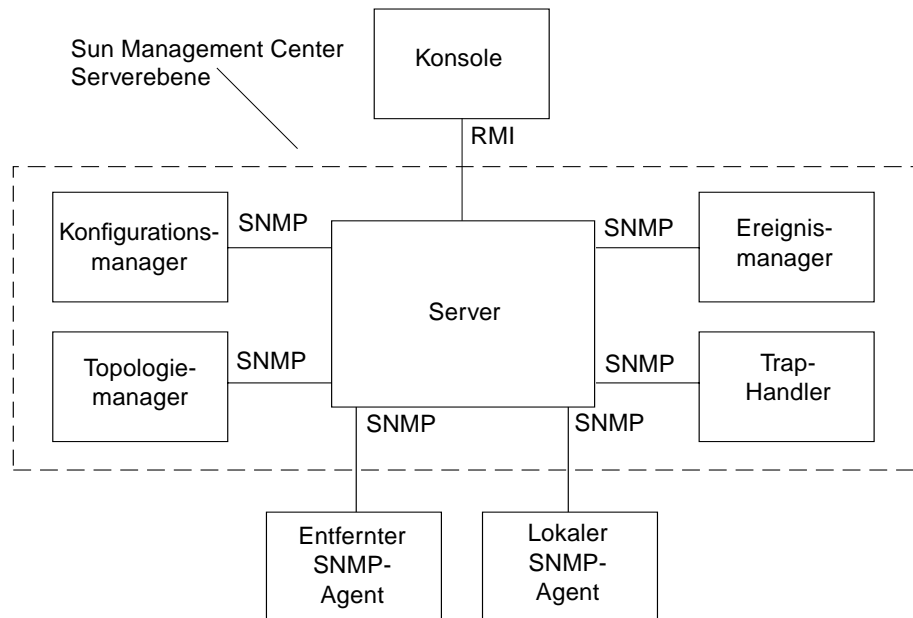
ABBILDUNG 1-2 Sun Management Center Serverebene
