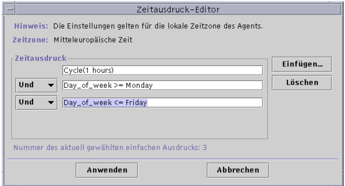
ABBILDUNG 11-7 Zeitausdruck-Editor mit einem einstündigen Zyklus im Bereich Montag bis Freitag
