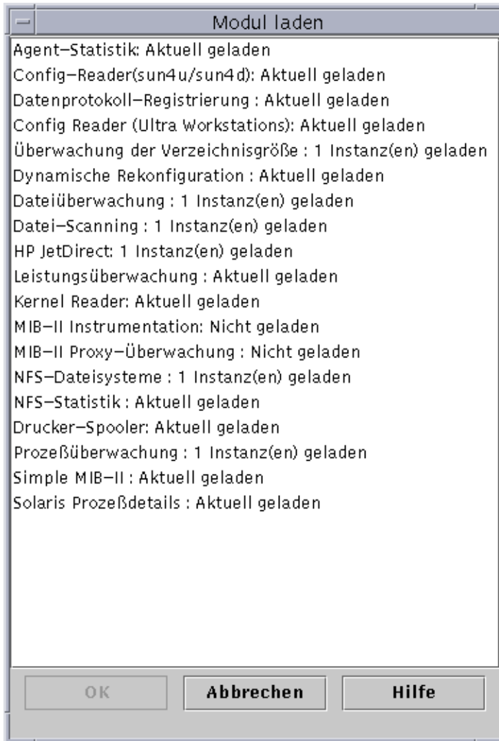
ABBILDUNG 12-5 Das Dialogfeld "Modul laden"
