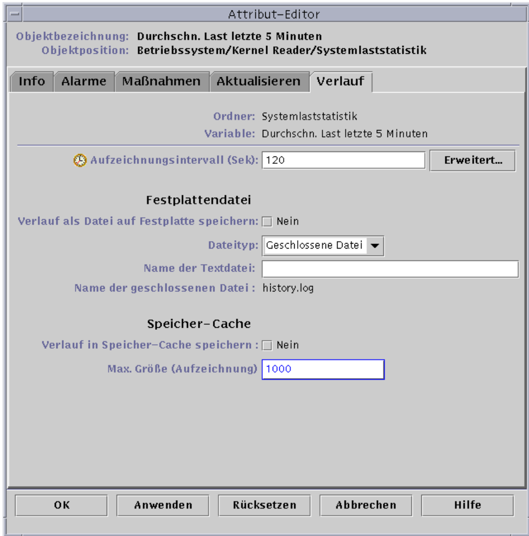
ABBILDUNG 10-7 Das Register "Verlauf" im Attribut-Editor für eine überwachte Eigenschaft
