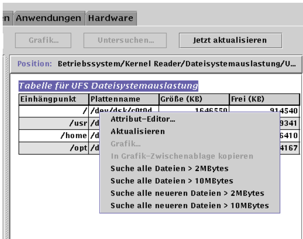
ABBILDUNG C-1 Untersuchungsbefehle für Dateisystemsyntax
