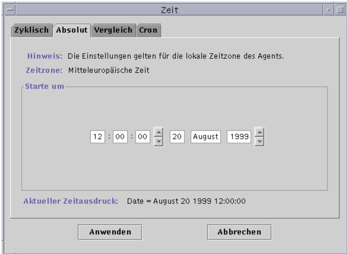
ABBILDUNG 11-9 Start um 12:00:00 vorm. am 20. August 1999
