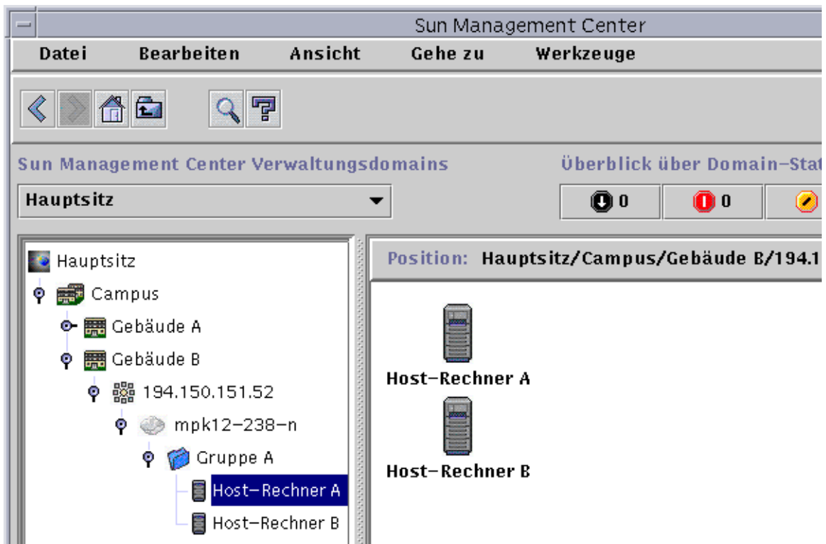
ABBILDUNG 4-1 Beispiel-Verwaltungsdomain
