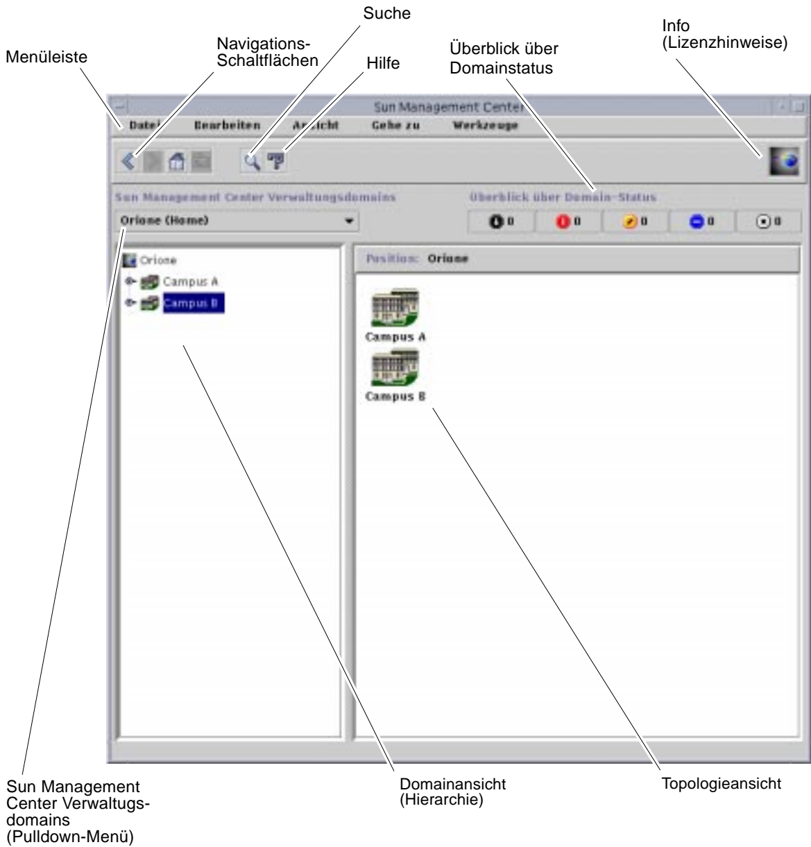
ABBILDUNG 7-1 Hauptkonsolenfenster
