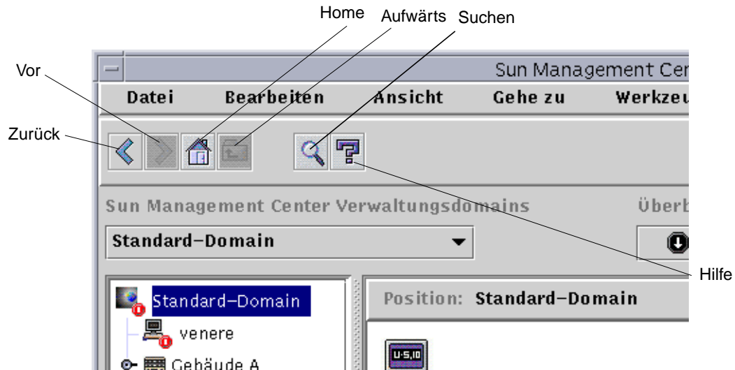
ABBILDUNG 7-5 Navigationsschaltflächen
