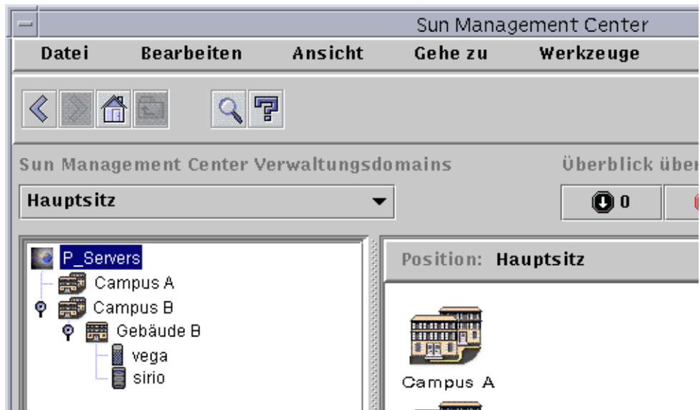
ABBILDUNG 4-5 Stammdomain
