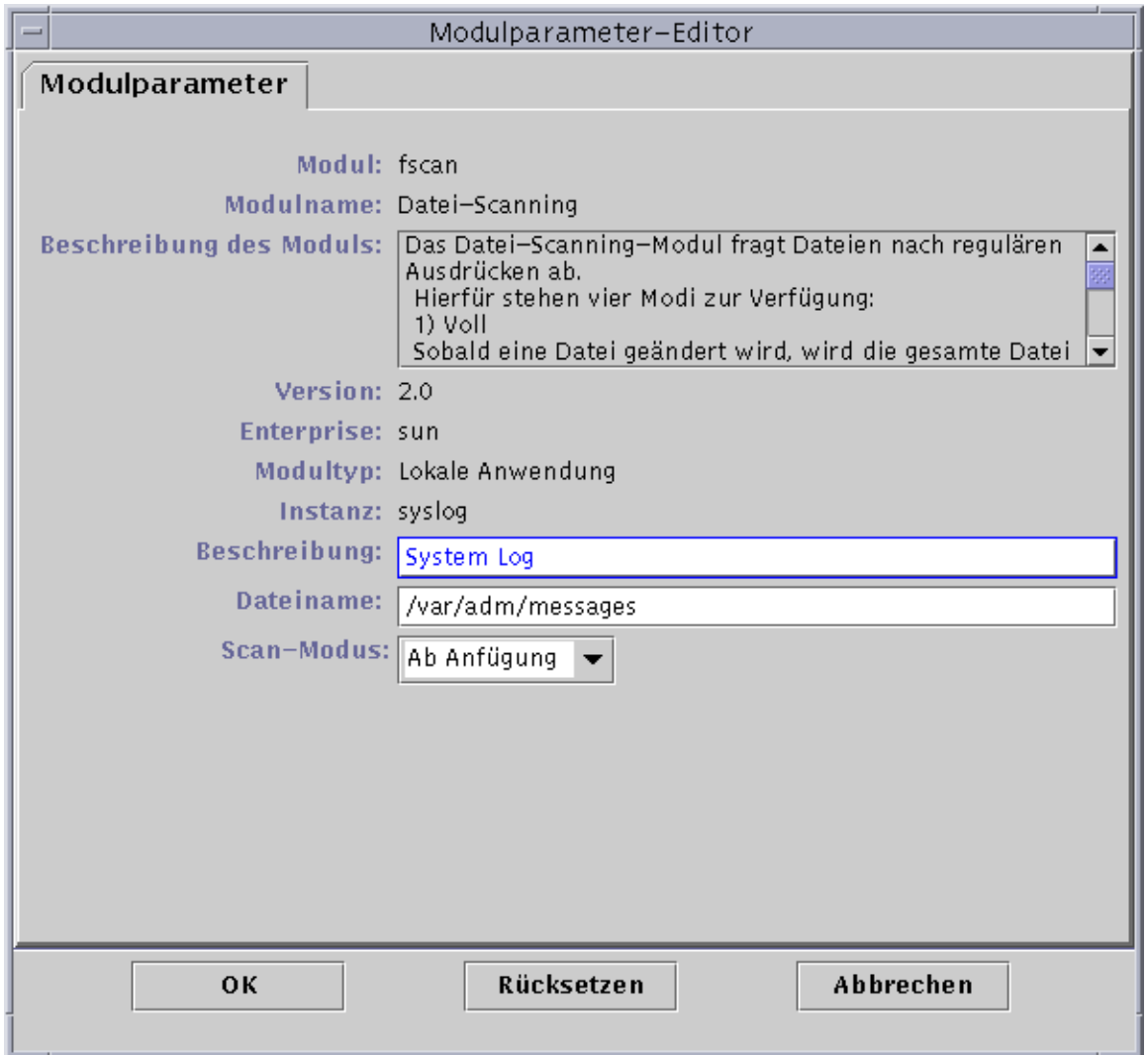
ABBILDUNG 12-11 Modulparameter-Editor
