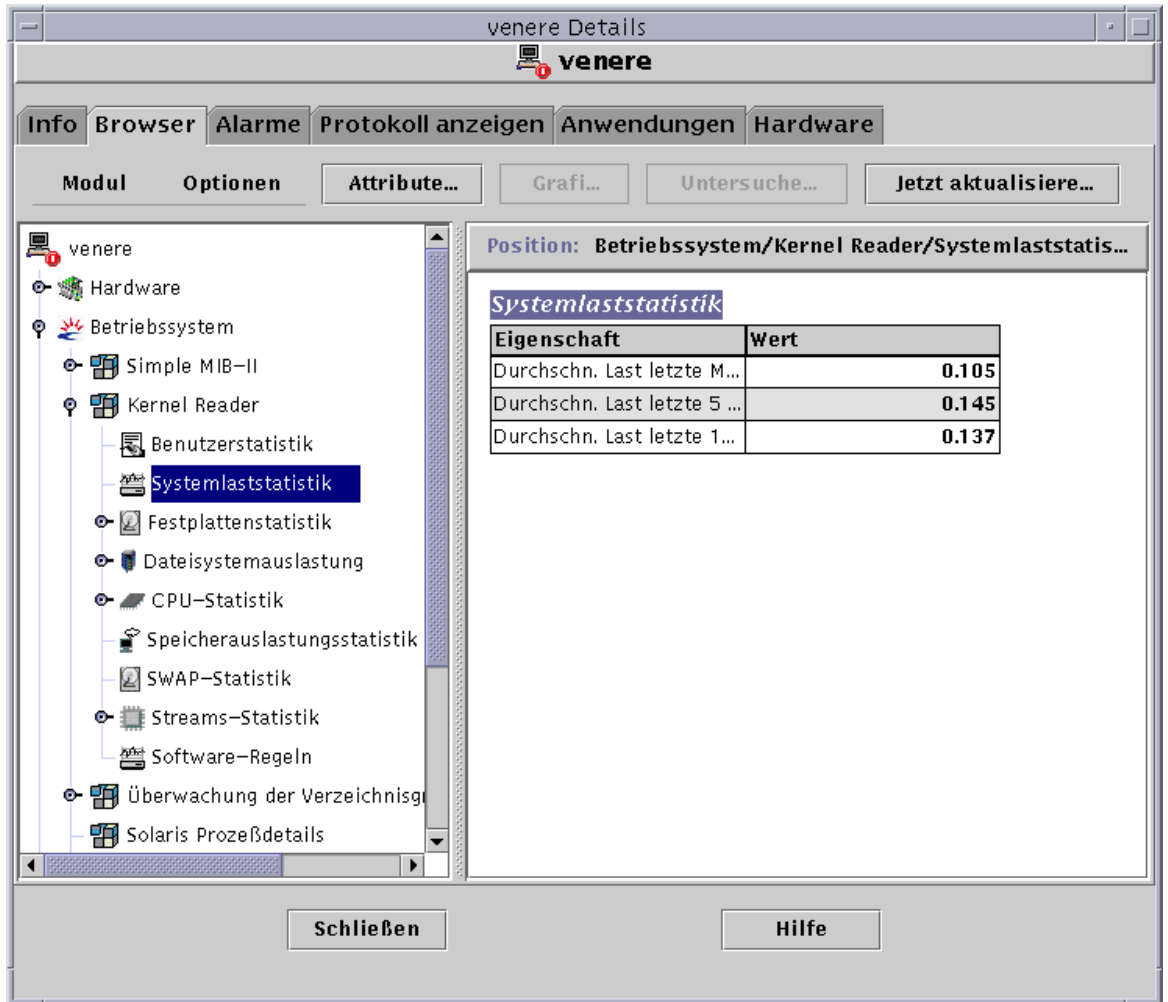
ABBILDUNG 9-1 Systemlaststatistik
