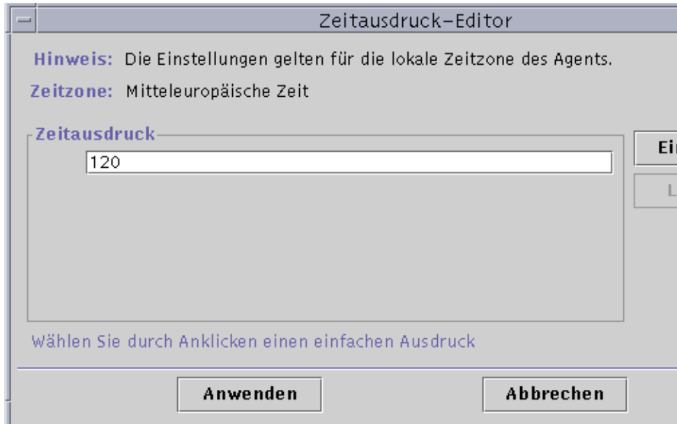
ABBILDUNG 11-1 Zeitausdruck-Editor
