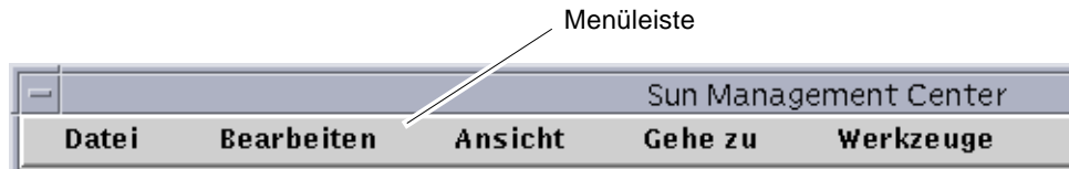
ABBILDUNG 7-4 Menüleiste
