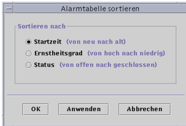
ABBILDUNG 13-13 Alarmtabelle sortieren
