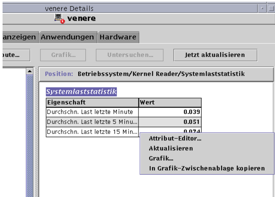
ABBILDUNG 10-1 Gewählte Dateneigenschaft
