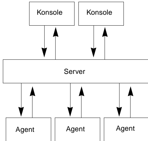
ABBILDUNG 1-1 Sun Management Center Komponentenebenen
