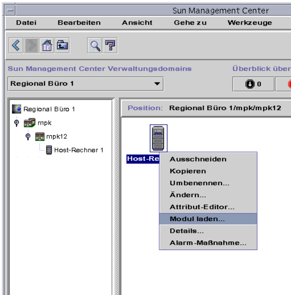
ABBILDUNG 12-2 Das Popup-Menü "Modul laden" in der Topologieansicht
