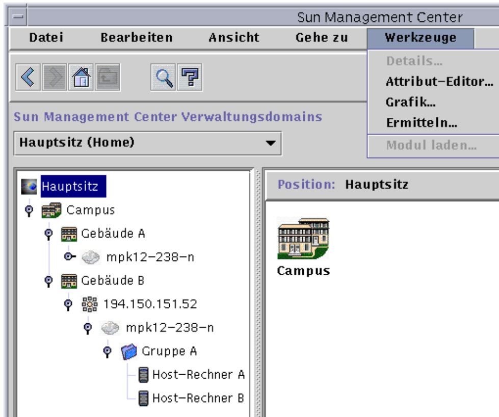
ABBILDUNG 8-2 Öffnen des Detailfensters über das Menü "Werkzeuge"
