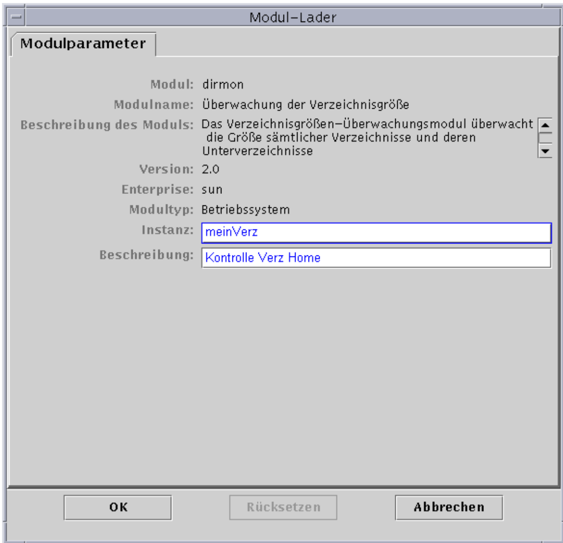
ABBILDUNG 12-6 Das Dialogfeld "Modul-Lader" für die Verzeichnisgrößenüberwachung
