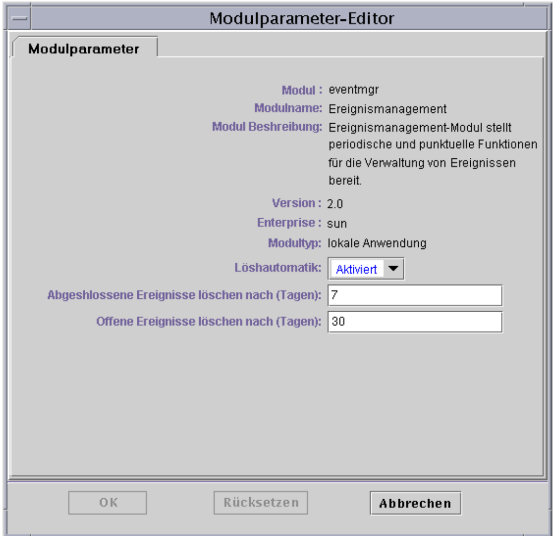
ABBILDUNG B-5 Modulparameter-Editor für das Ereignismanagement-Modul
