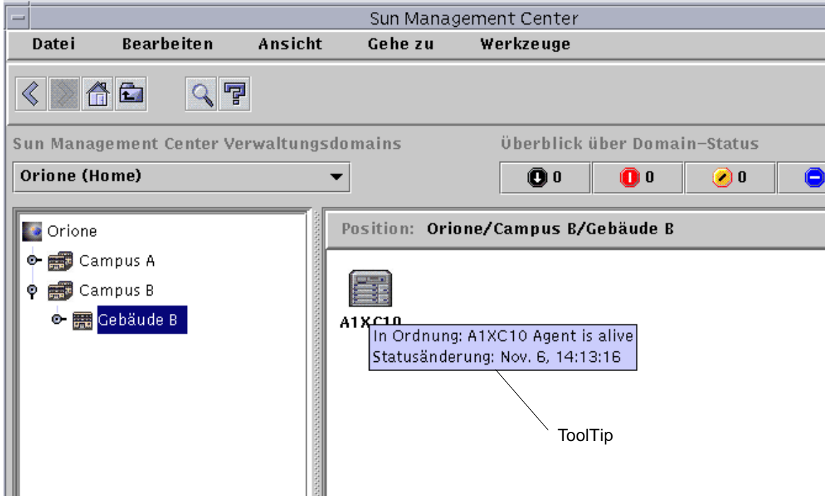
ABBILDUNG 7-3 ToolTip
