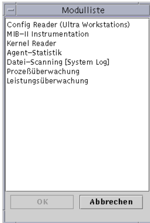
ABBILDUNG 5-3 Modulliste
