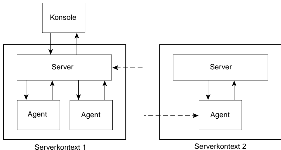
ABBILDUNG 15-1 Entfernter Serverkontext
