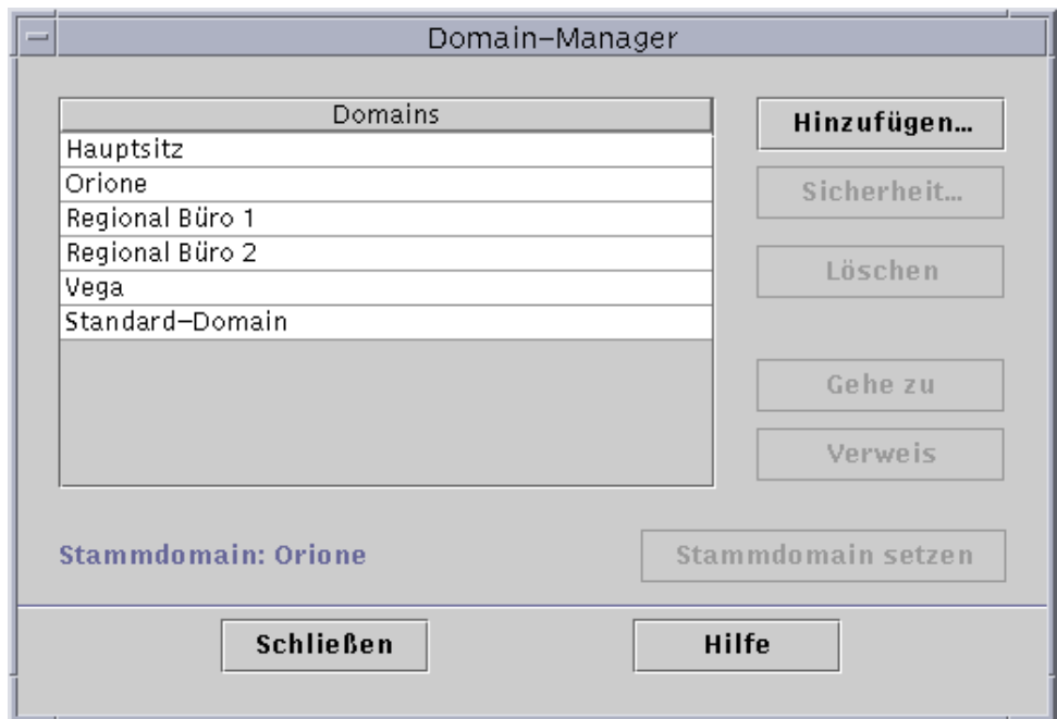
ABBILDUNG 4-6 Domain-Manager
