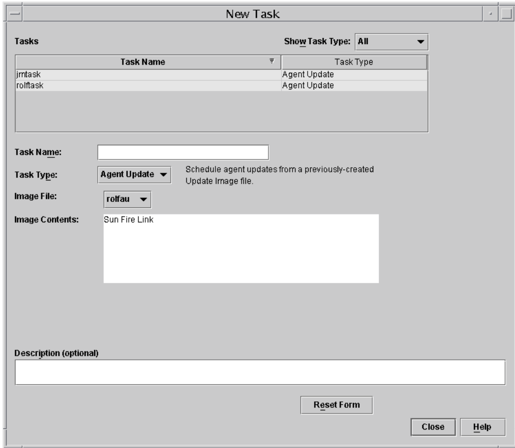
图 2-10 “New Task（新任务）”面板
