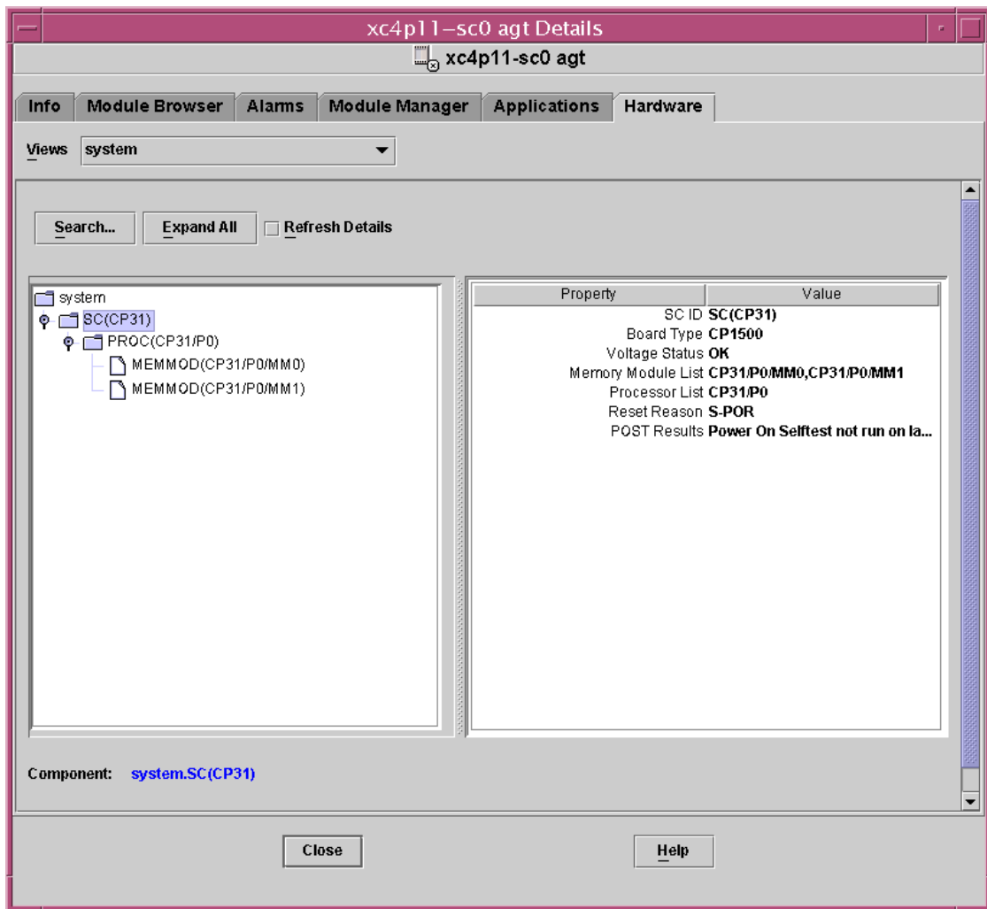
图 5-13 Sun Fire 15K/12K 系统控制器 (CP1500) 逻辑视图
