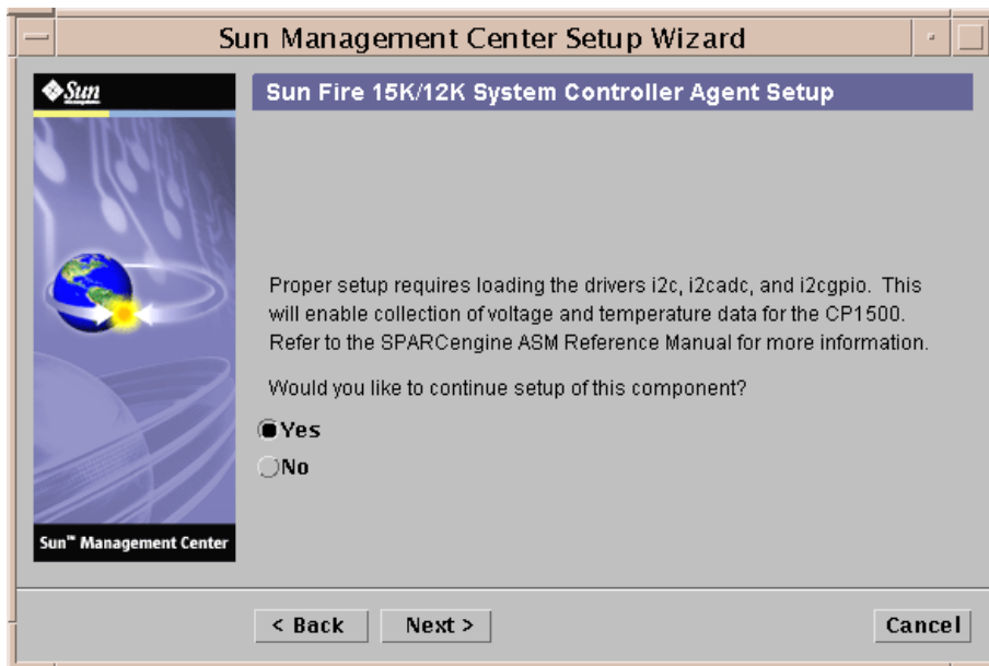
图 2-5 CP1500 系统控制器代理设置
