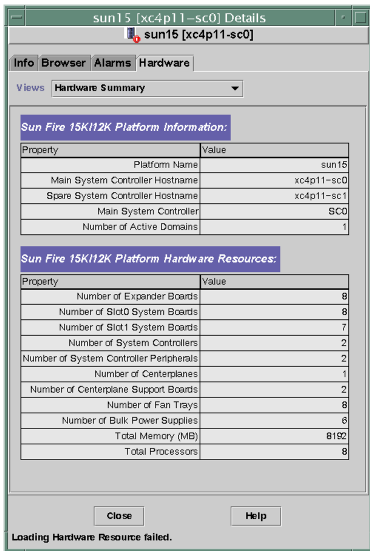
图 5-1 Sun Fire 15K/12K 平台的硬件摘要
