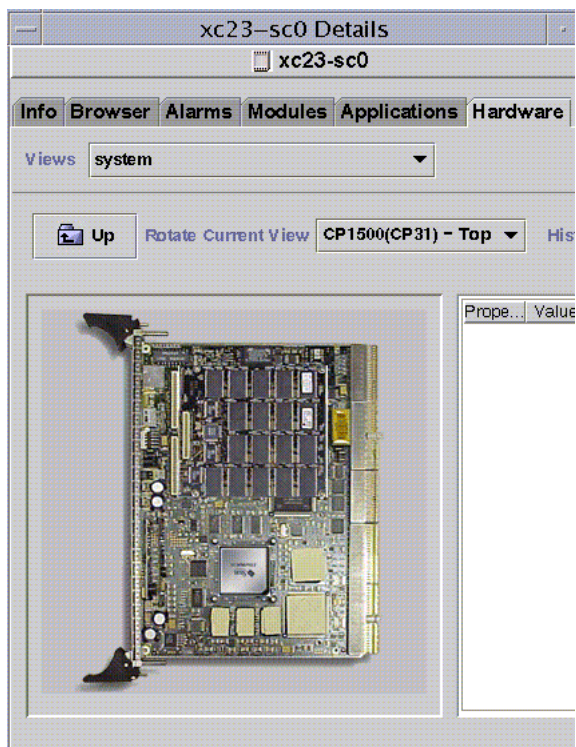
图 5-11 CP1500 系统控制器物理视图的顶端
