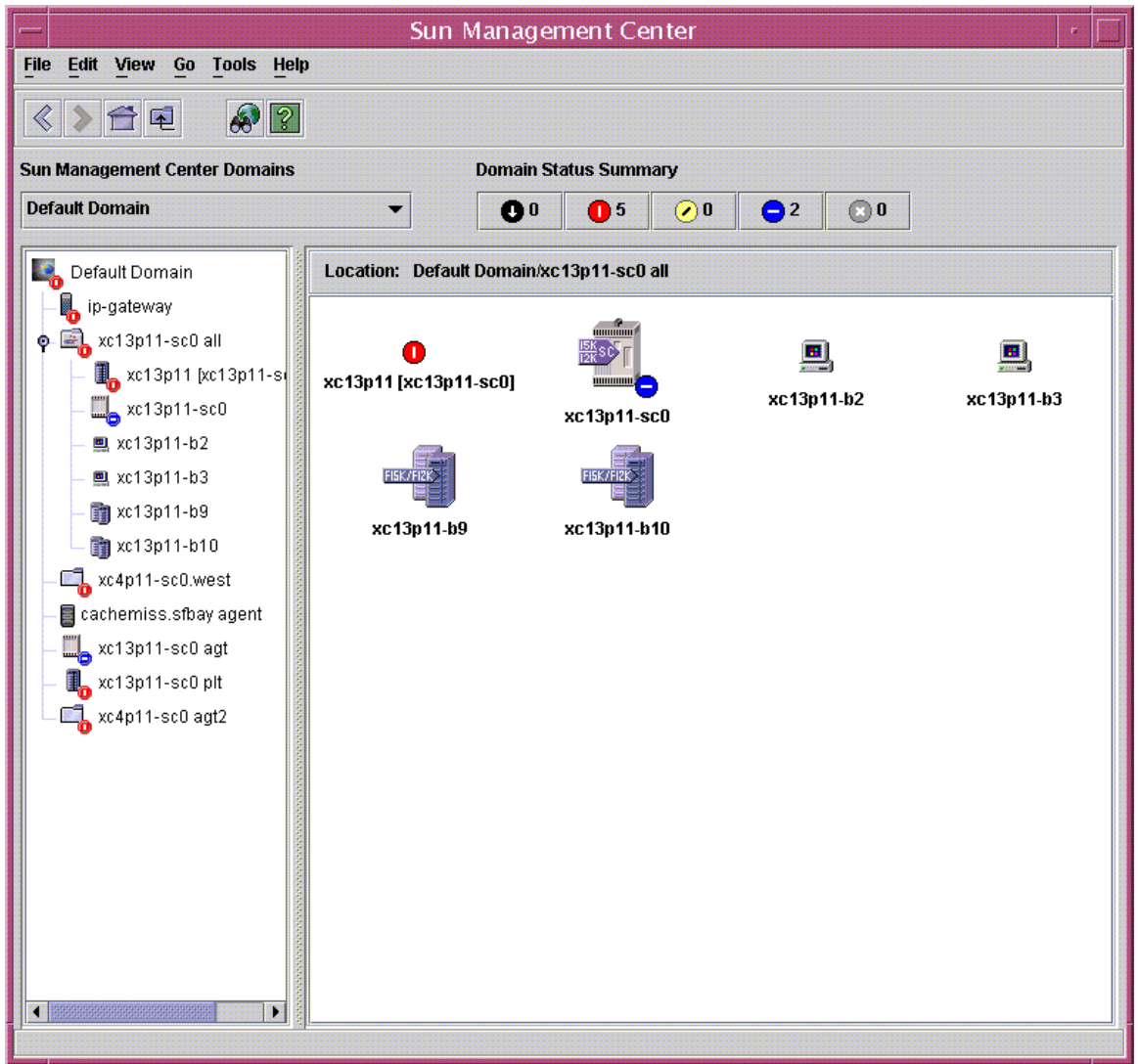
图 4-1 Sun Fire 15K/12K 组合对象示例
