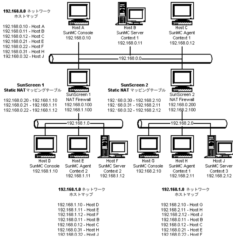
図 D-3 複雑な NAT ネットワーク 構成例
