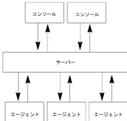
図 2-1 Sun Management Center の基本アーキテクチャー
