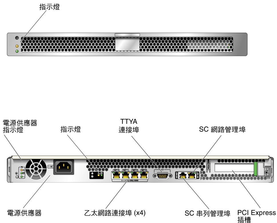
圖 3 Sun SPARC Enterprise T1000 伺服器前方與後方面板
