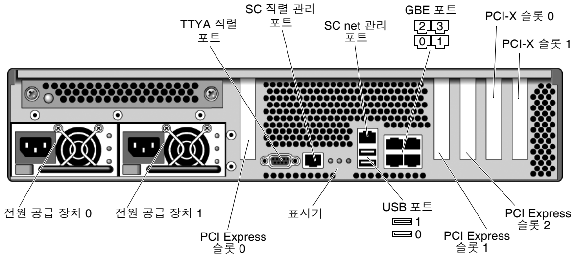
그림 4 Sun SPARC Enterprise T2000 서버 후면 패널
