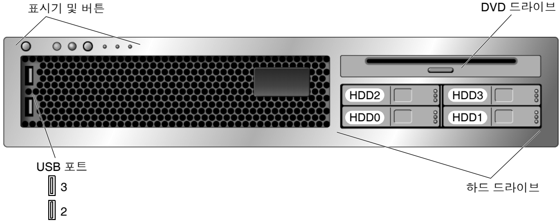
그림 3 Sun SPARC Enterprise T2000 서버 전면 패널
