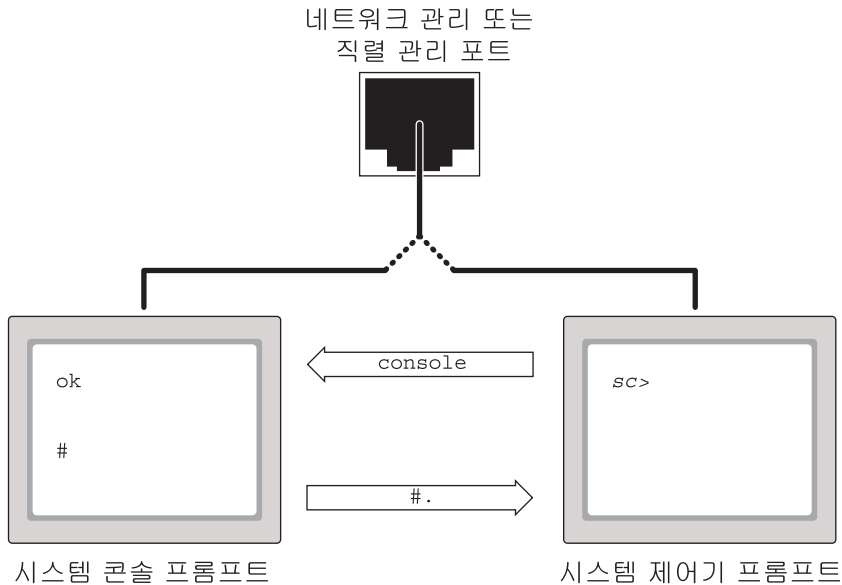
그림 1-5 시스템 콘솔과 시스템 제어기 채널 분리
