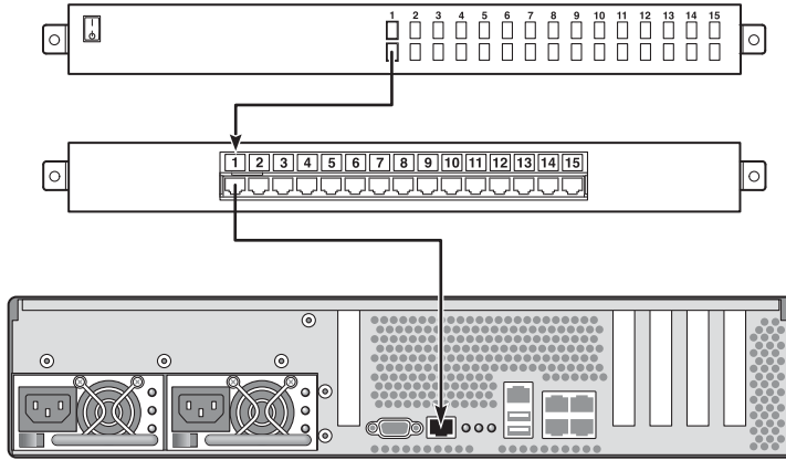
그림 1-3 단말기 서버와 SPARC Enterprise T2000 서버 간의 패치 패널 연결
