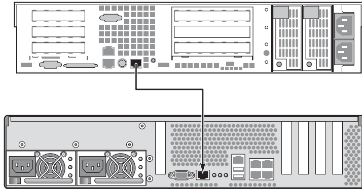
그림 1-4 SPARC Enterprise T2000 서버와 다른 시스템 간 TIP 연결
