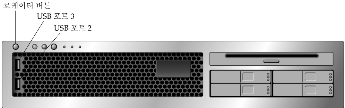
그림 2-1 SPARC Enterprise T2000 새시의 로케이터 버튼
