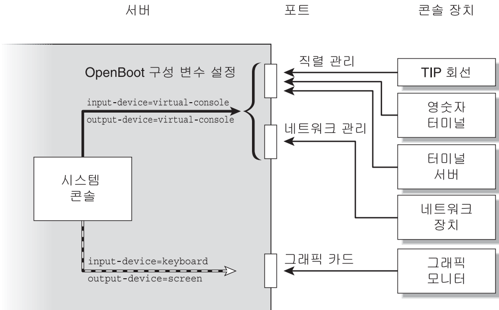
그림 1-1 시스템 콘솔 지정
