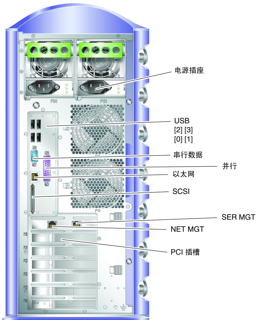
图 1-4 I/O 端口位置
