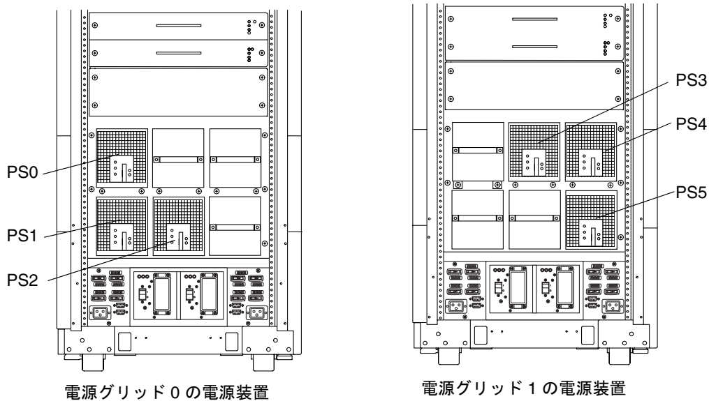
図 4-2 電源グリッド 0 および電源グリッド 1 の電源装置 — Sun Fire E6900 システム
