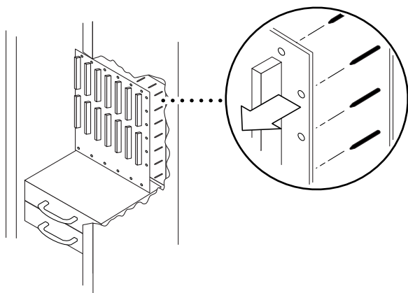
図 11-7 センタープレーンを手前に引くことによるガイドピンの取り外し — Sun Fire E6900 システム
