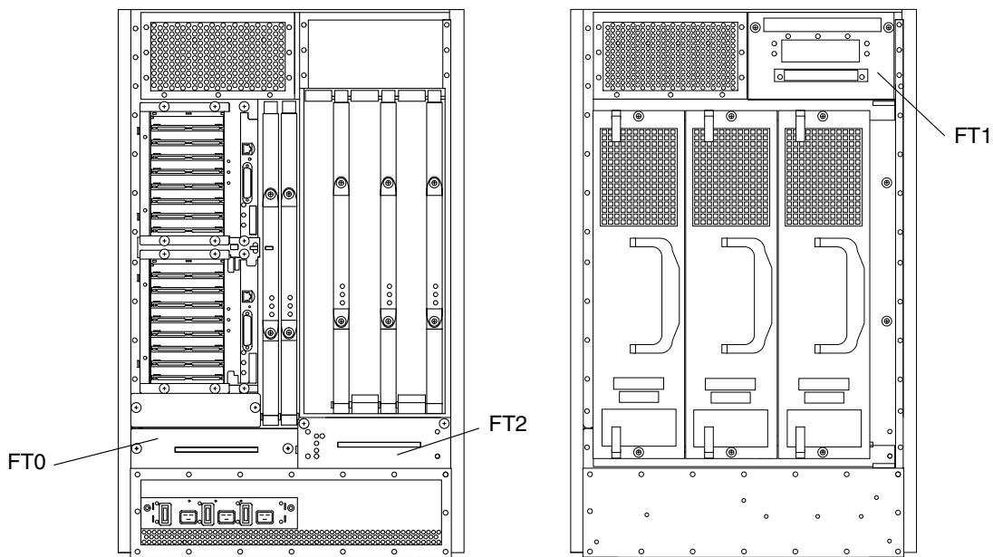
図 6-2 背面および正面のファントレー — Sun Fire E4900 システム
