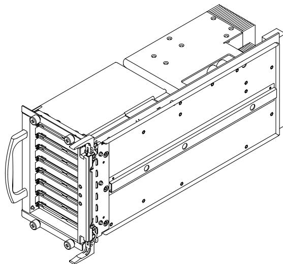
図 C-6 PCI/PCI+/PCI-X I/O アセンブリ
