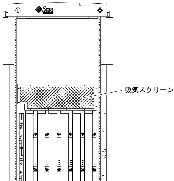
図 12-1 Sun Fire E6900 システムの吸気スクリーンの場所 (正面図)
