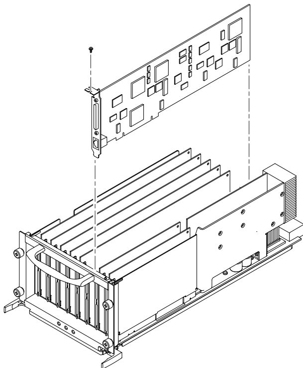
図 9-4 I/O アセンブリからの PCI カードの取り外し
