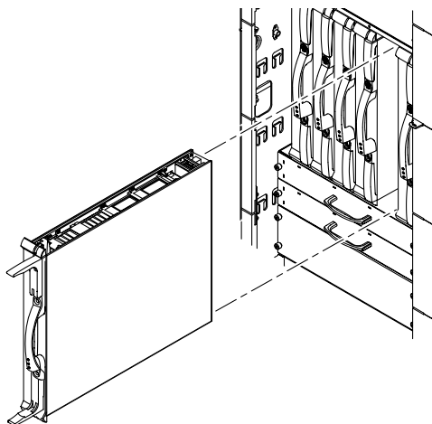
図 8-5 CPU/メモリーボードの取り外しまたは取り付け — Sun Fire E6900 システム
