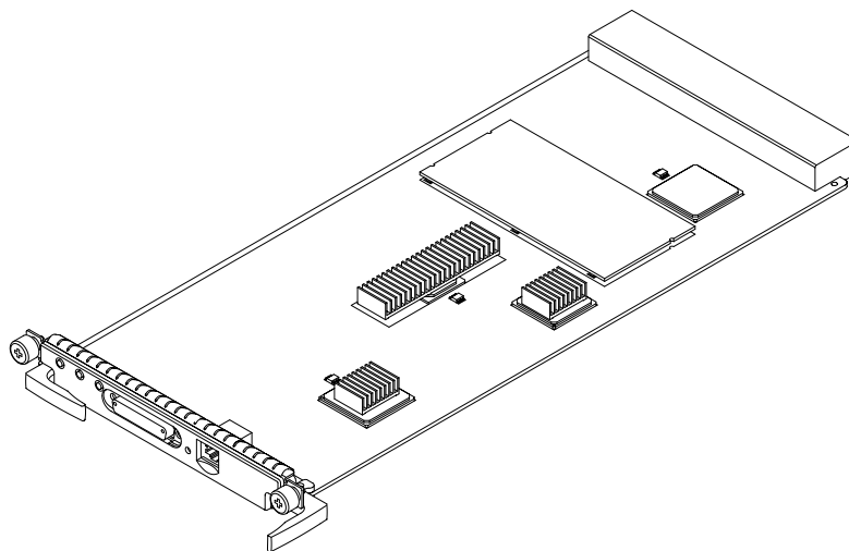
図 C-8 システムコントローラボード — Sun Fire E6900/E4900 システム
