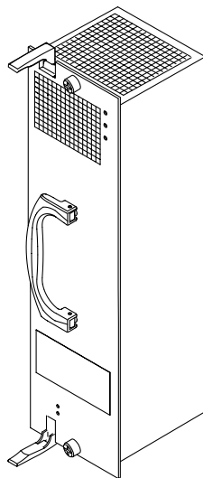
図 C-10 Sun Fire E4900 システムの電源装置
