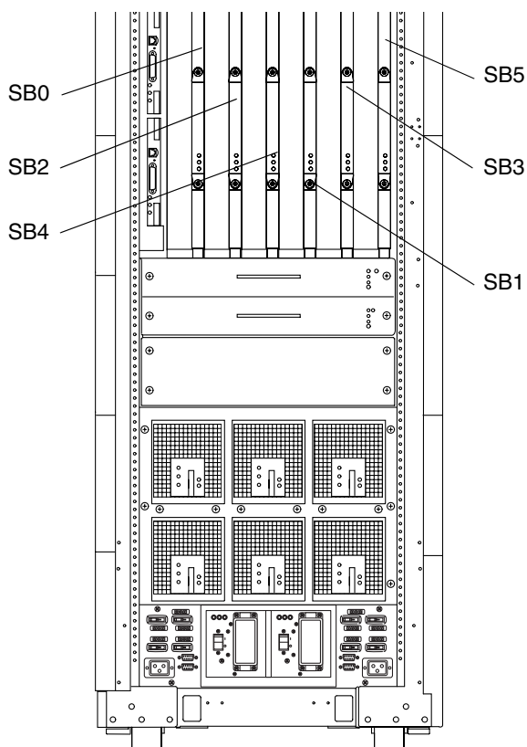
図 8-2 CPU/メモリーボードのスロット割り当て — Sun Fire E6900 システム (正面図)
