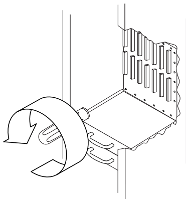
図 11-6 システムセンタープレーンを固定しているねじの取り外し — Sun Fire E6900 システム
