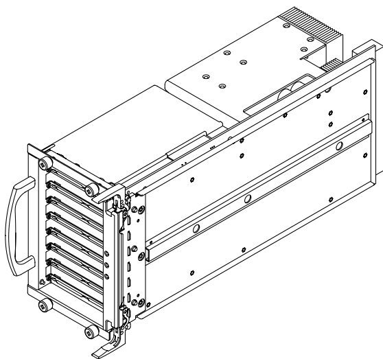
図 A-5 PCI/PCI+/PCI-X I/O アセンブリ
