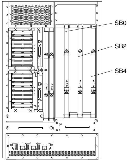
図 8-3 CPU/メモリーボードのスロット割り当て — Sun Fire E4900 システム (背面図)
