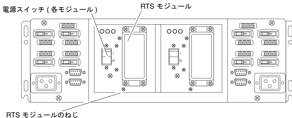
図 4-13 RTU アセンブリ
