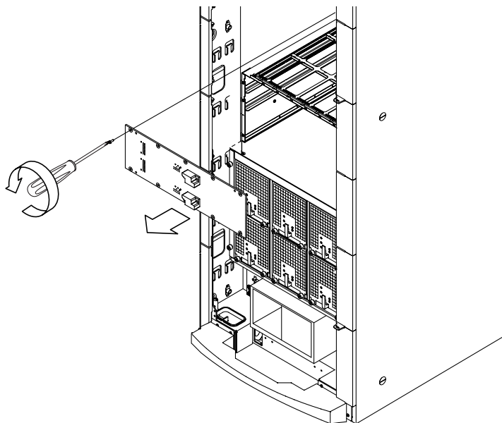
図 11-10 ファンセンタープレーンを固定しているねじの取り外し
