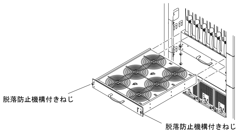
図 6-3 正面ファントレイの取り外しまたは取り付け — Sun Fire E6900 システム
