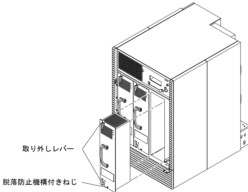
図 4-5 電源装置の取り外しまたは取り付け — Sun Fire E4900 システム
