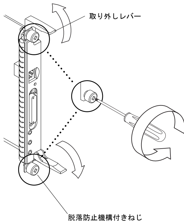
図 7-5 脱落防止機構付きねじおよび取り外しレバーの緩め方
