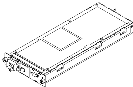
図 4-6 AC 入力ボックス — Sun Fire E6900 システム
