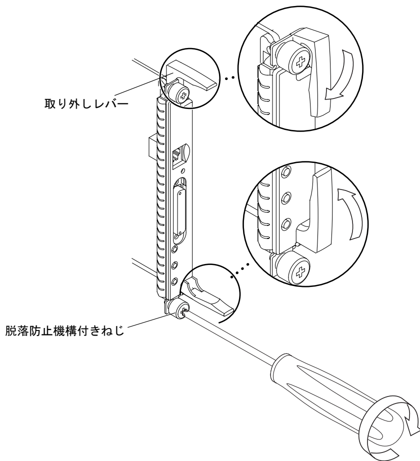
図 7-7 脱落防止機構付きねじの締め方および取り外しレバーのロック方法
