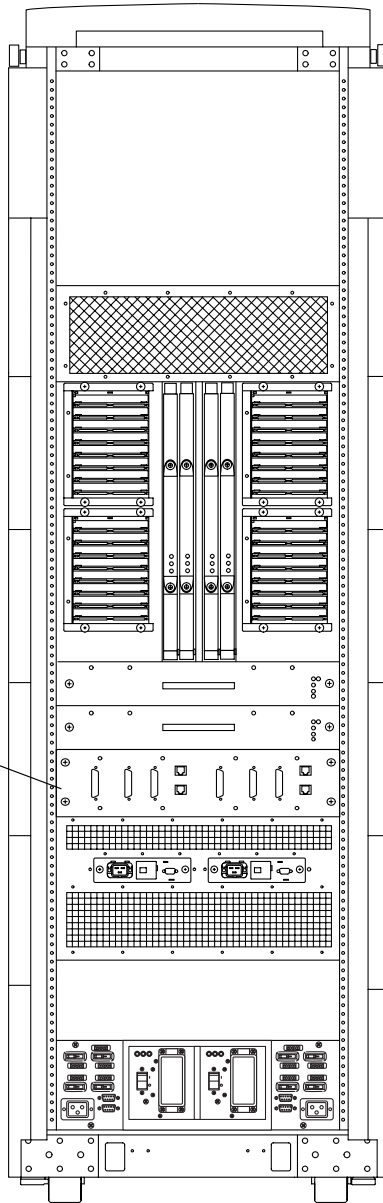
図 B-1 Sun Fire E6900 システムのシリアル番号の場所 (背面図)
