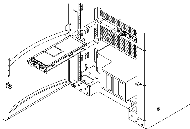
図 4-10 AC 入力ボックスの取り外し — Sun Fire E6900 システム
