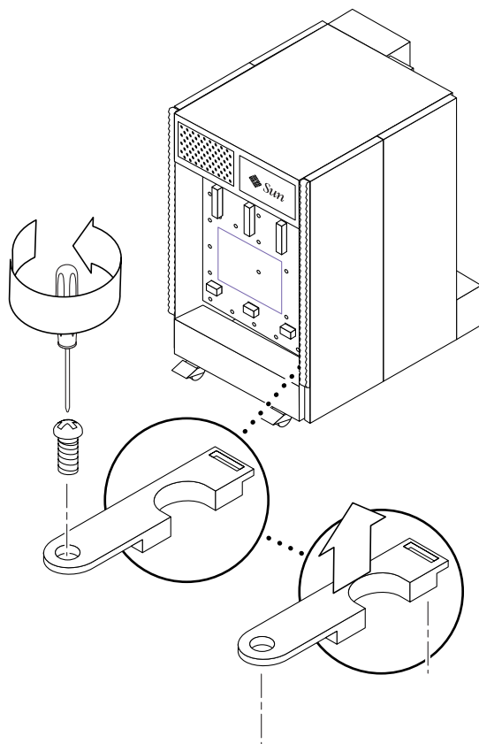
図 11-18 ケーブルガイドの取り外し — Sun Fire E4900 システム
