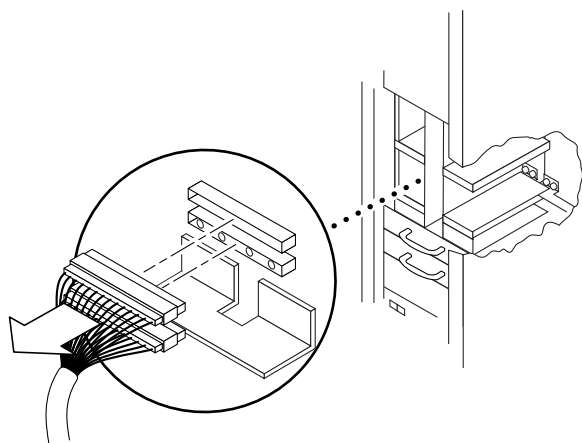
図 11-5 システムセンタープレーンからの 2 本のケーブルの取り外し — Sun Fire E6900 システム
