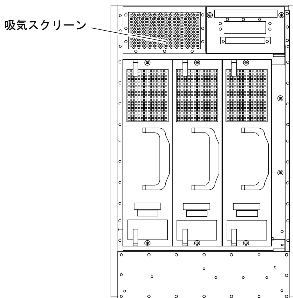
図 12-2 Sun Fire E4900 システムの吸気スクリーンの場所 (正面図)
