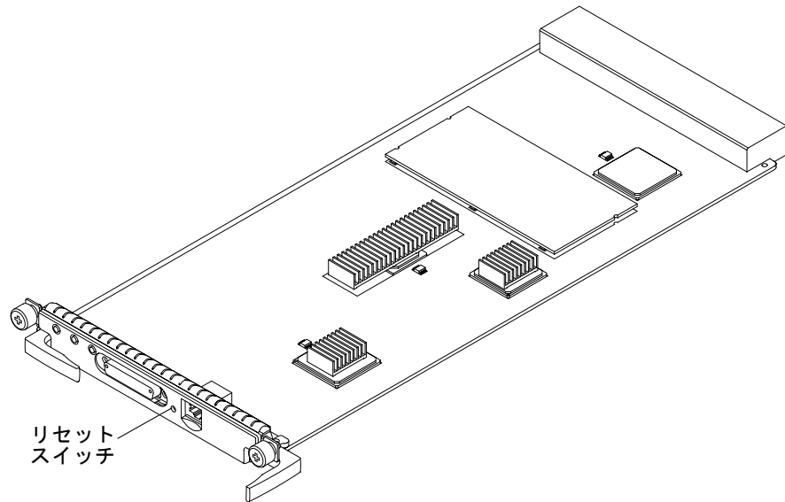
図 7-4 システムコントローラボードのリセットスイッチ
