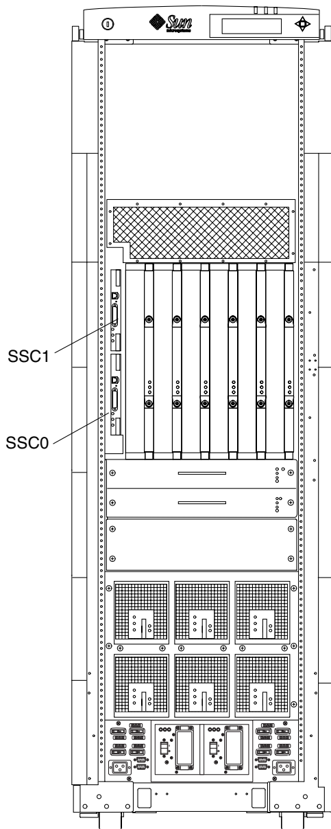
図 7-2 Sun Fire E6900 システムのシステムコントローラボードのロット割り当て (正面図)
