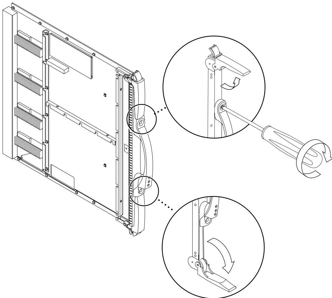
図 10-4 取り外しレバーのロック解除
