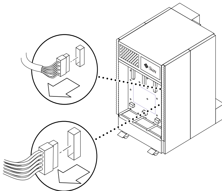
図 11-16 センタープレーンのコネクタからのケーブルの取り外し — Sun Fire E4900 システム
