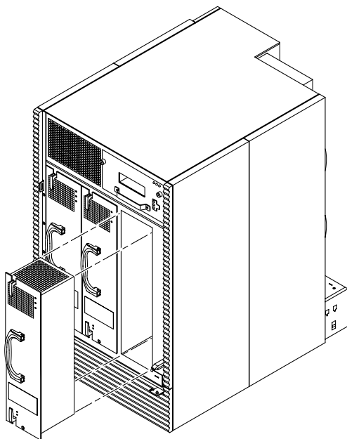
図 11-15 Sun Fire E4900 システムの正面からの電源装置の取り外し
