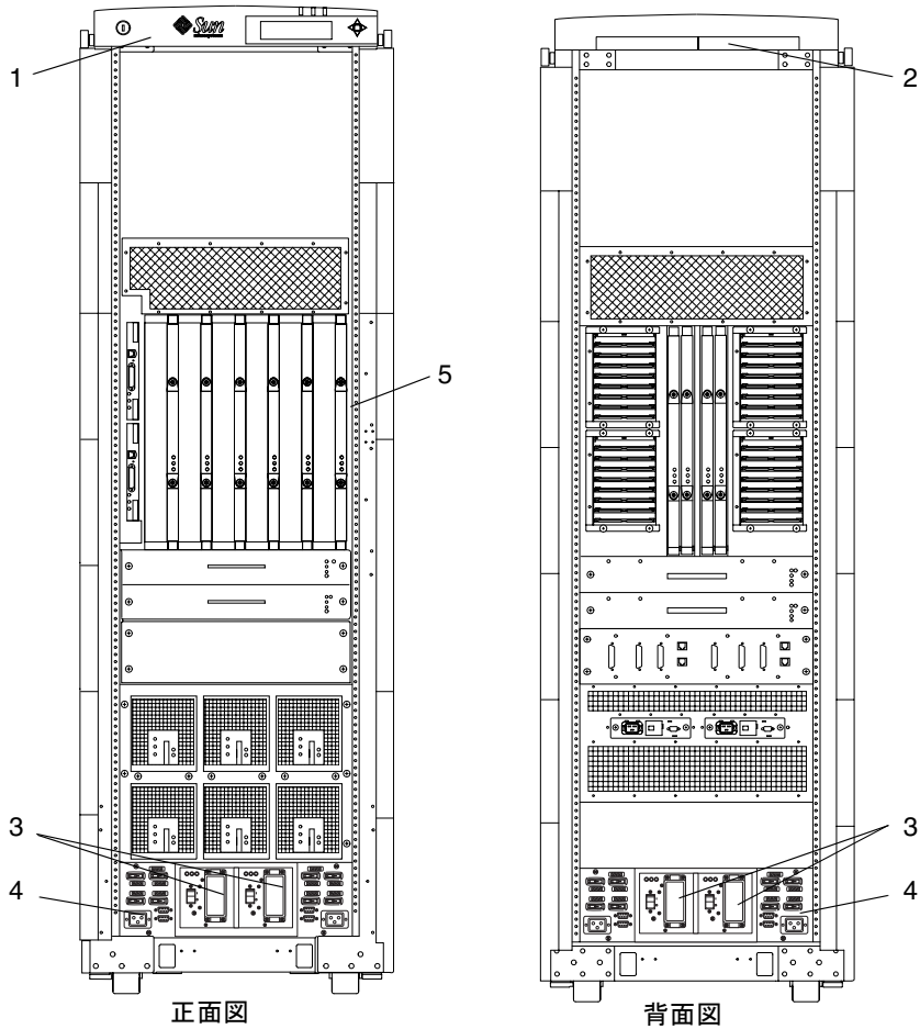
図 C-2 Sun Fire E6900 システムキャビネット
