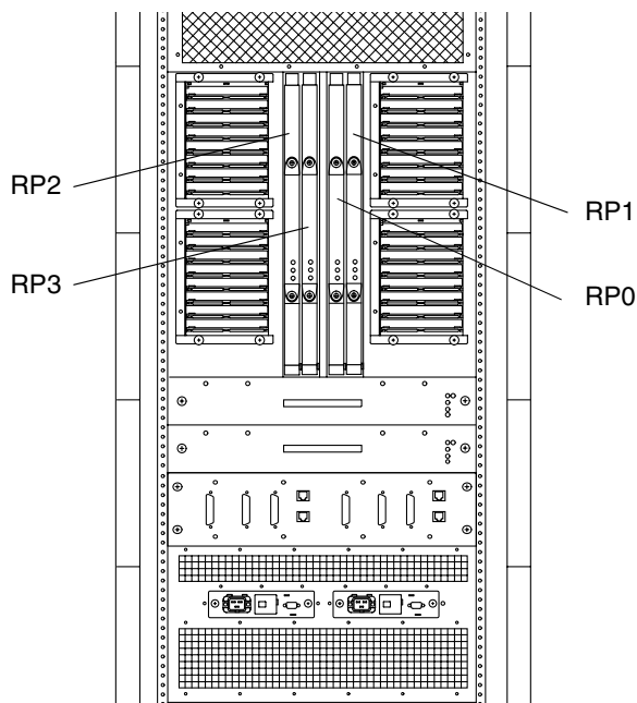
図 10-1 Sun Fire E6900 システムのリピータボードのスロット割り当て (背面図)
