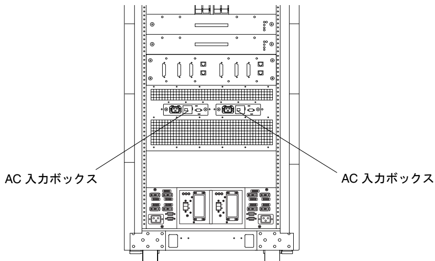
図 2-2 AC 入力ボックス — Sun Fire E6900 システム (背面図)
