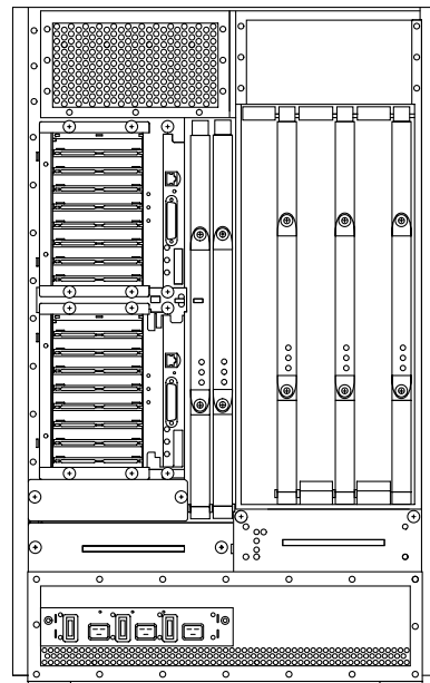
背面図
