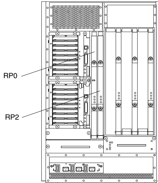
図 10-2 Sun Fire E4900 システムのリピータボードのスロット割り当て (背面図)
