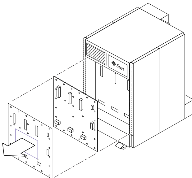
図 11-20 センタープレーンおよび絶縁体の取り外し — Sun Fire E4900 システム
