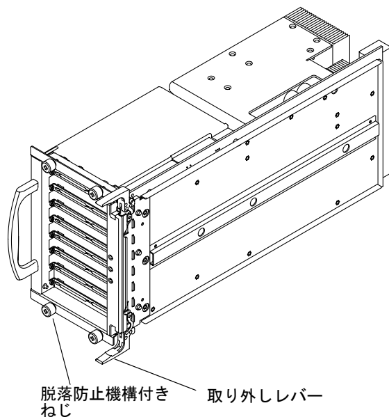
図 9-3 I/O アセンブリ
