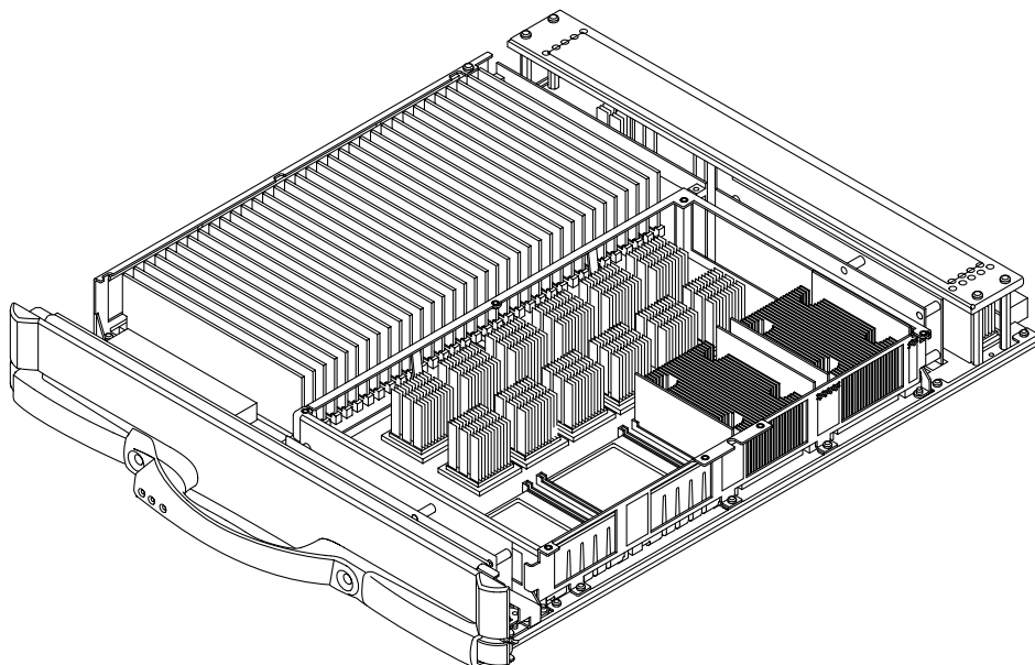
図 A-4 カバーを取り外した CPU/メモリーボード
