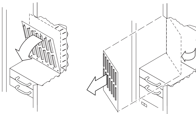
図 11-8 システムセンタープレーンの取り外し — Sun Fire E6900 システム
