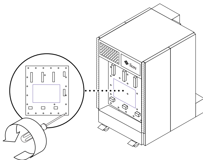
図 11-19 センタープレーンをシステムに固定しているねじの取り外し — Sun Fire E4900 システム
