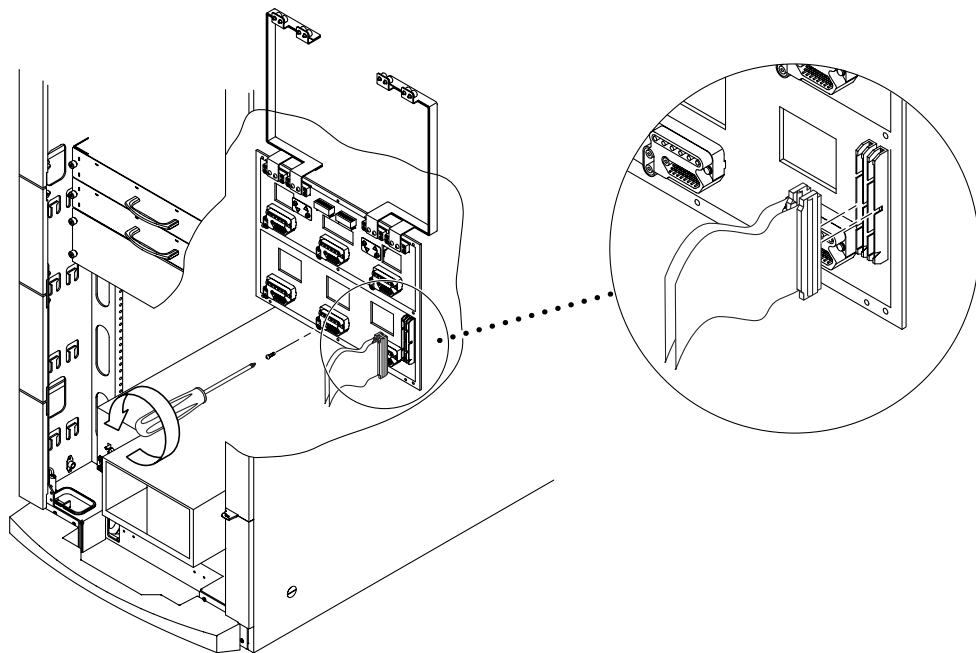
図 11-11 センタープレーンケーブル — Sun Fire E6900 システム
