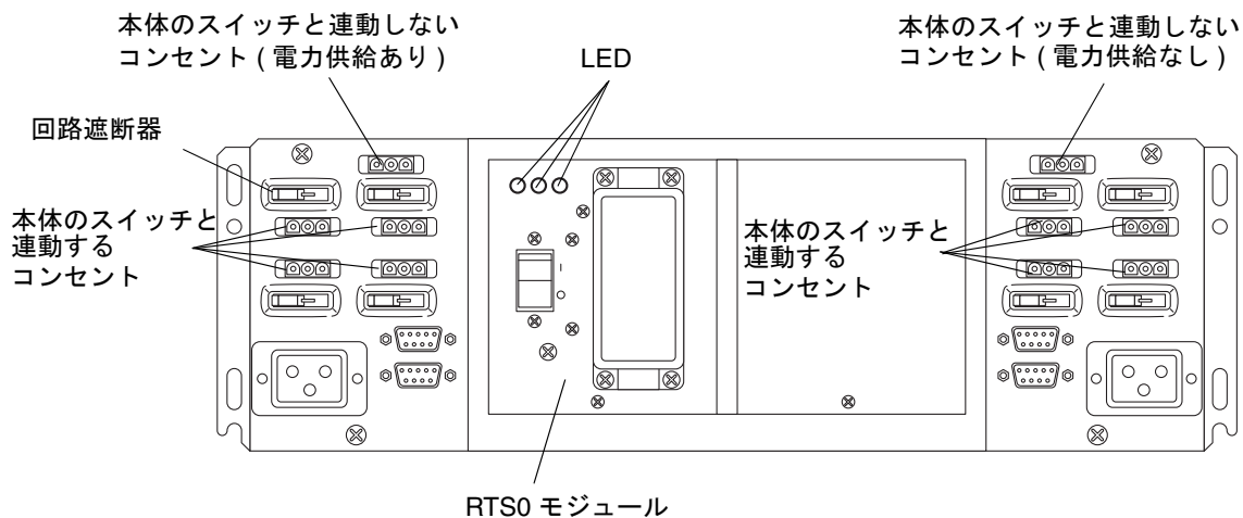
図 4-11 RTU および RTS モジュール
