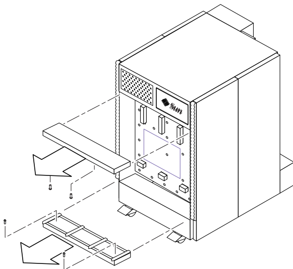
図 11-17 上部および下部の電源装置補助材の取り外し — Sun Fire E4900 システム
