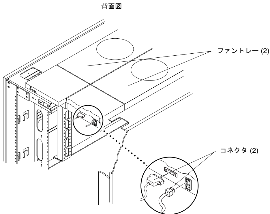
図 6-5 キャビネットのファントレーの電源スイッチおよびコネクタ
