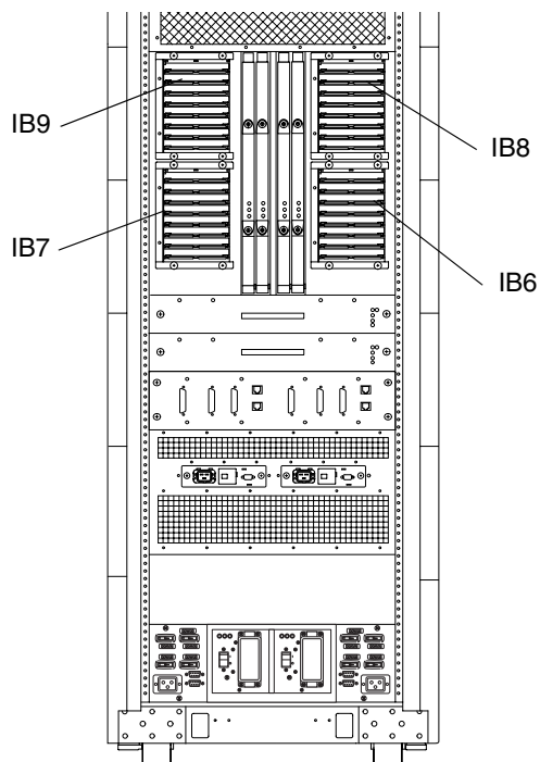
図 9-1 Sun Fire E6900 システムの I/O アセンブリ (背面図)
