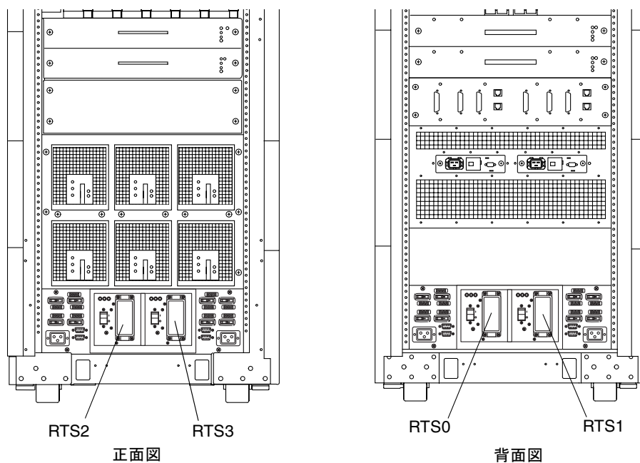
図 4-12 RTS モジュール — Sun Fire E6900 システム
