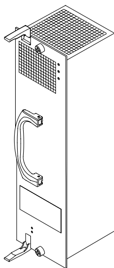
図 A-8 Sun Fire E4900 システムの電源装置
