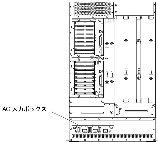
図 2-3 AC 入力ボックス — Sun Fire E4900 システム (背面図)
