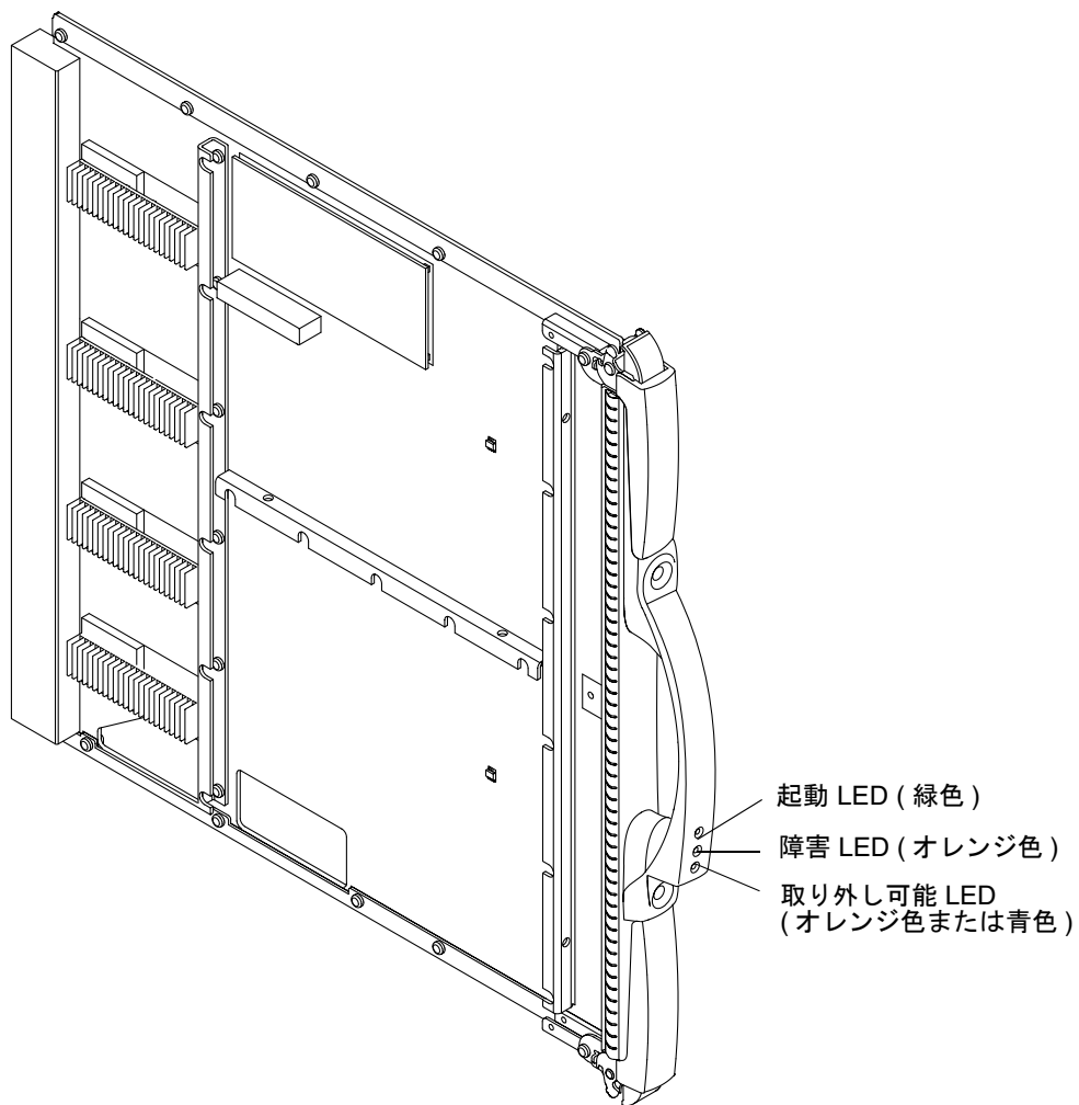
図 10-3 リピータボードの LED
