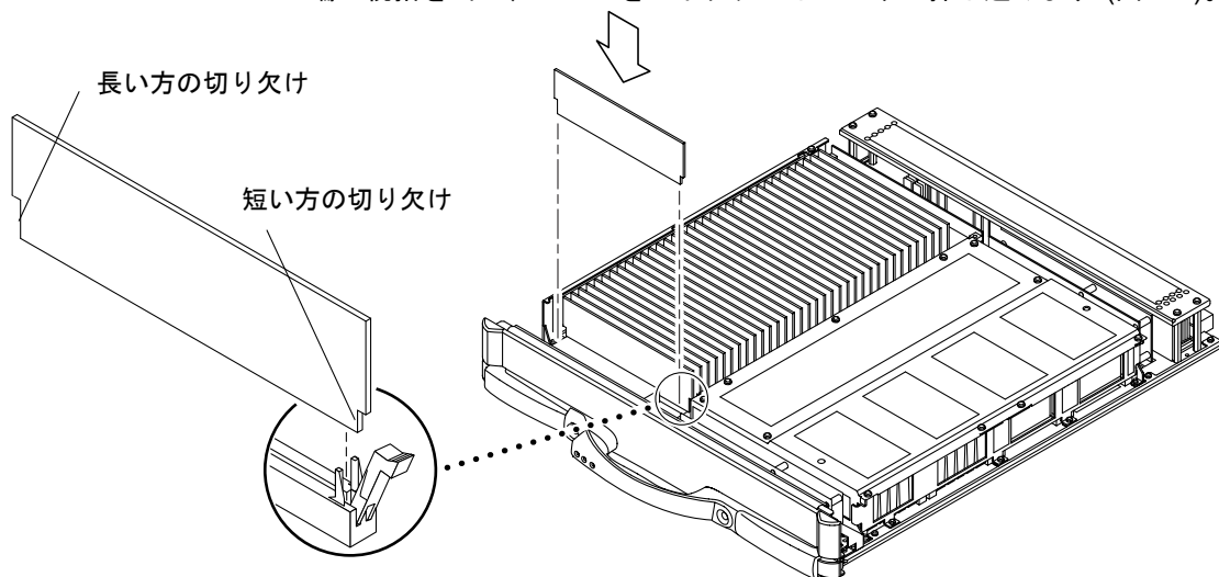
図 8-8 DIMM の取り付け
