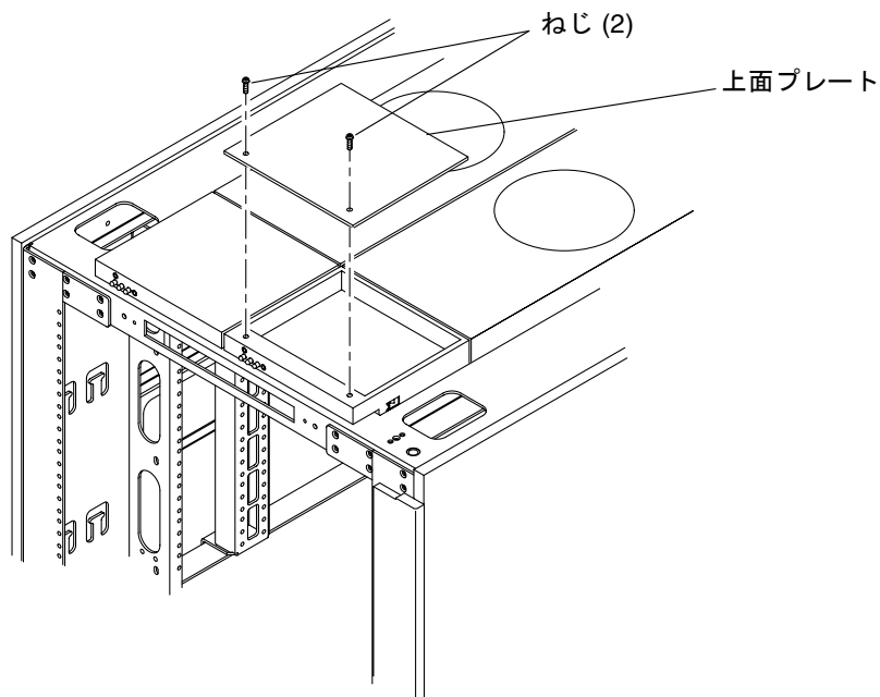
図 6-6 キャビネットのファントレーの上面プレート
