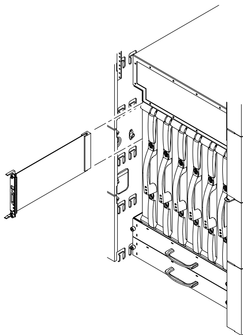
図 7-6 システムコントローラボードの取り外しおよび取り付け — Sun Fire E6900 システム
