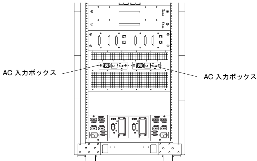
図 4-8 AC 入力ボックス — Sun Fire E6900 システム (背面図)
