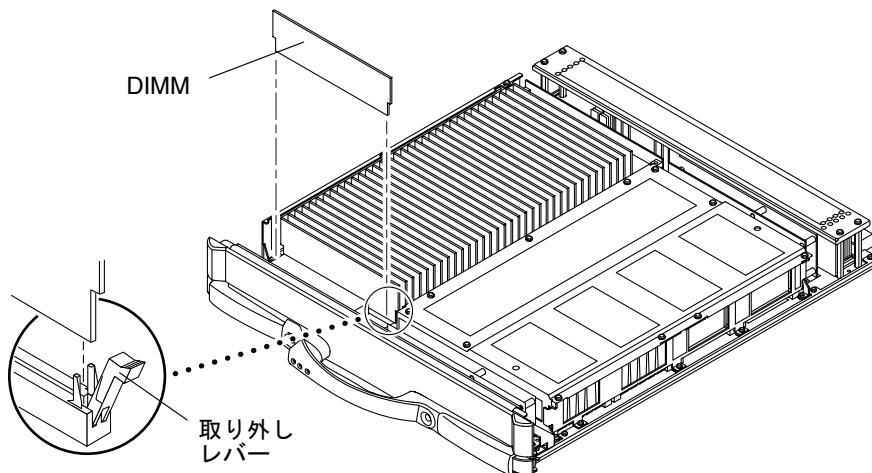
図 8-7 DIMM の取り外し
