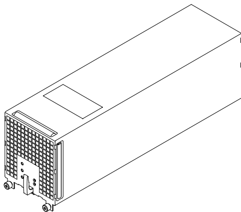
図 C-9 Sun Fire E6900 システムの電源装置
