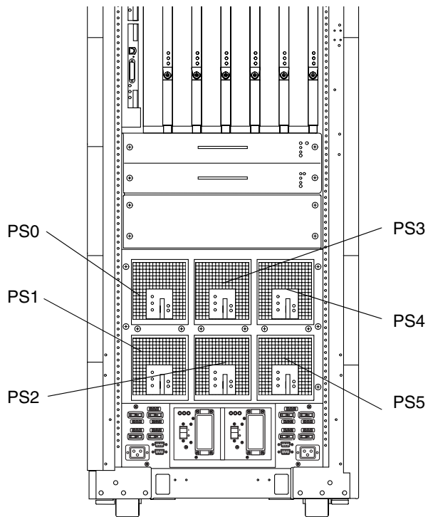
図 4-1 電源装置の場所 — Sun Fire E6900 システム (正面図)
