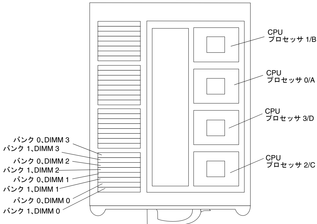
図 8-6 DIMM のスロット番号
