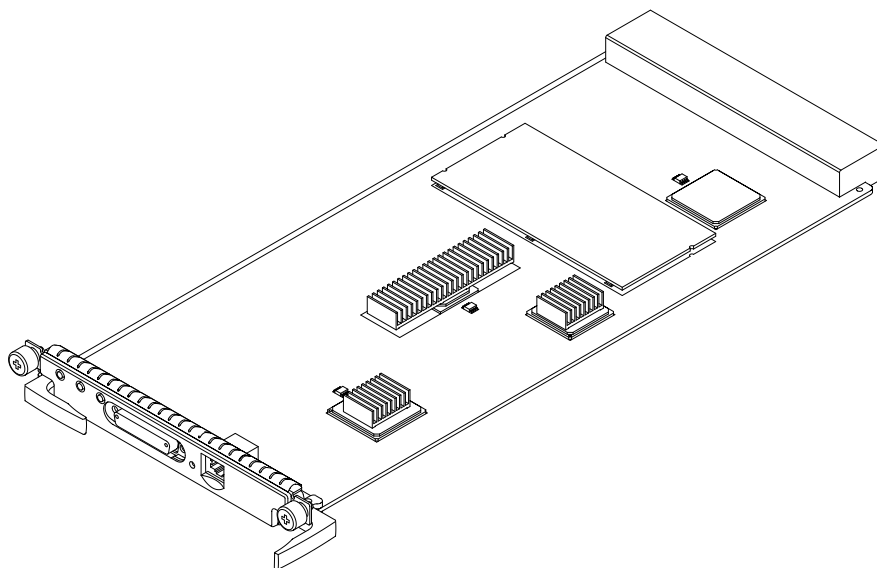
図 A-9 システムコントローラボード — Sun Fire E6900/E4900 システム
