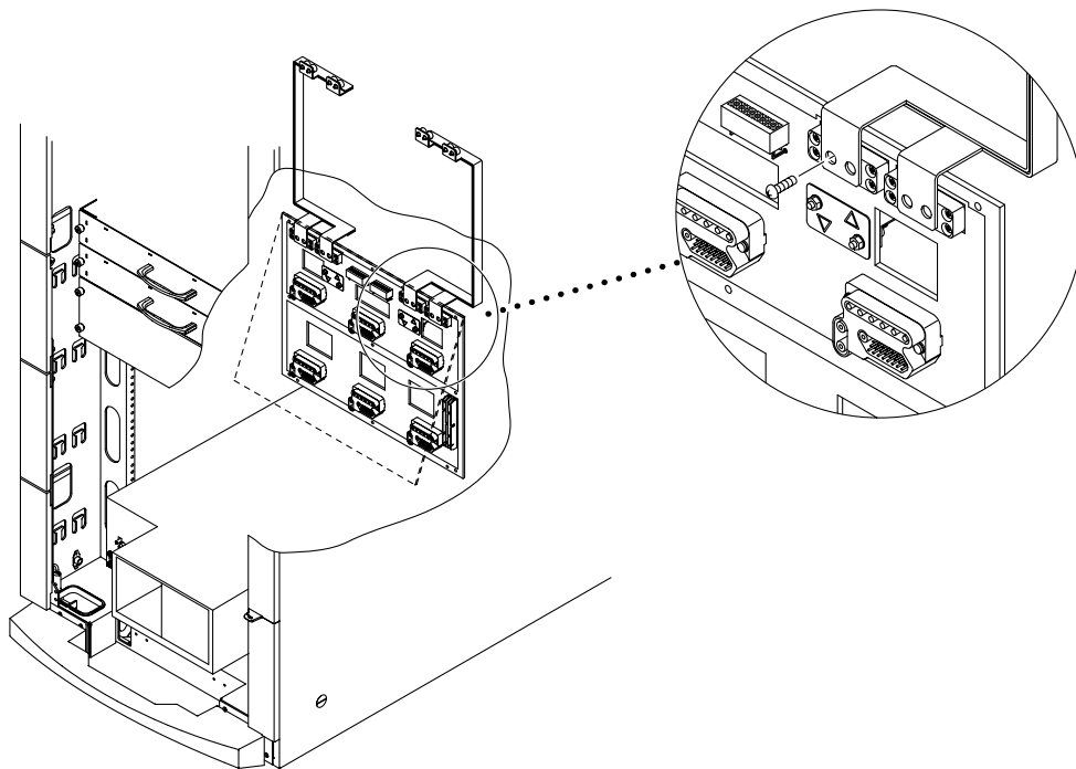
図 11-12 電源センタープレーンバスバーを固定しているねじの取り外し
