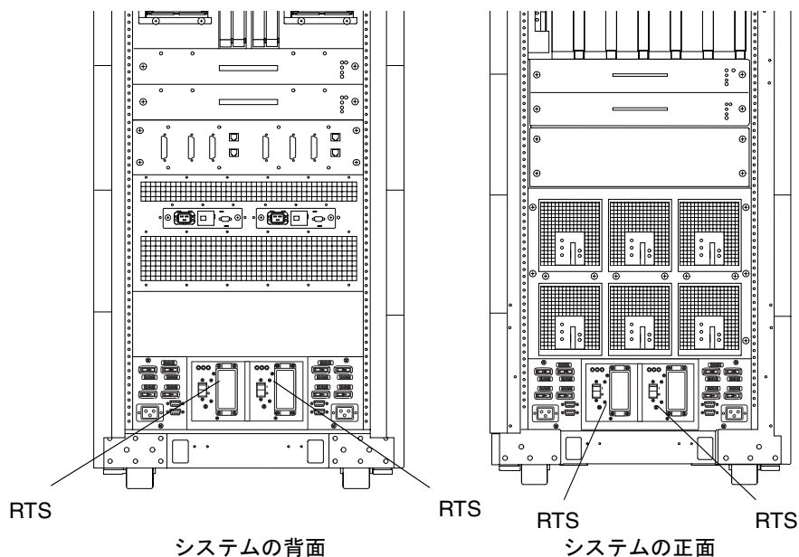
図 2-4 冗長転送スイッチ (RTS) — Sun Fire E6900 システム
