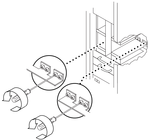
図 11-4 バスバーの脱落防止機構付きねじの緩め方 — Sun Fire E6900 システム
