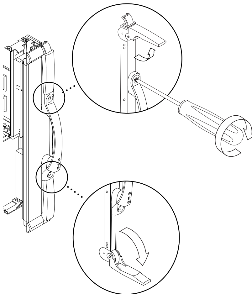
図 8-4 取り外しレバーのロック解除
