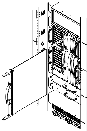
図 10-5 リピータボードの取り外しおよび取り付け — Sun Fire E6900 システム
