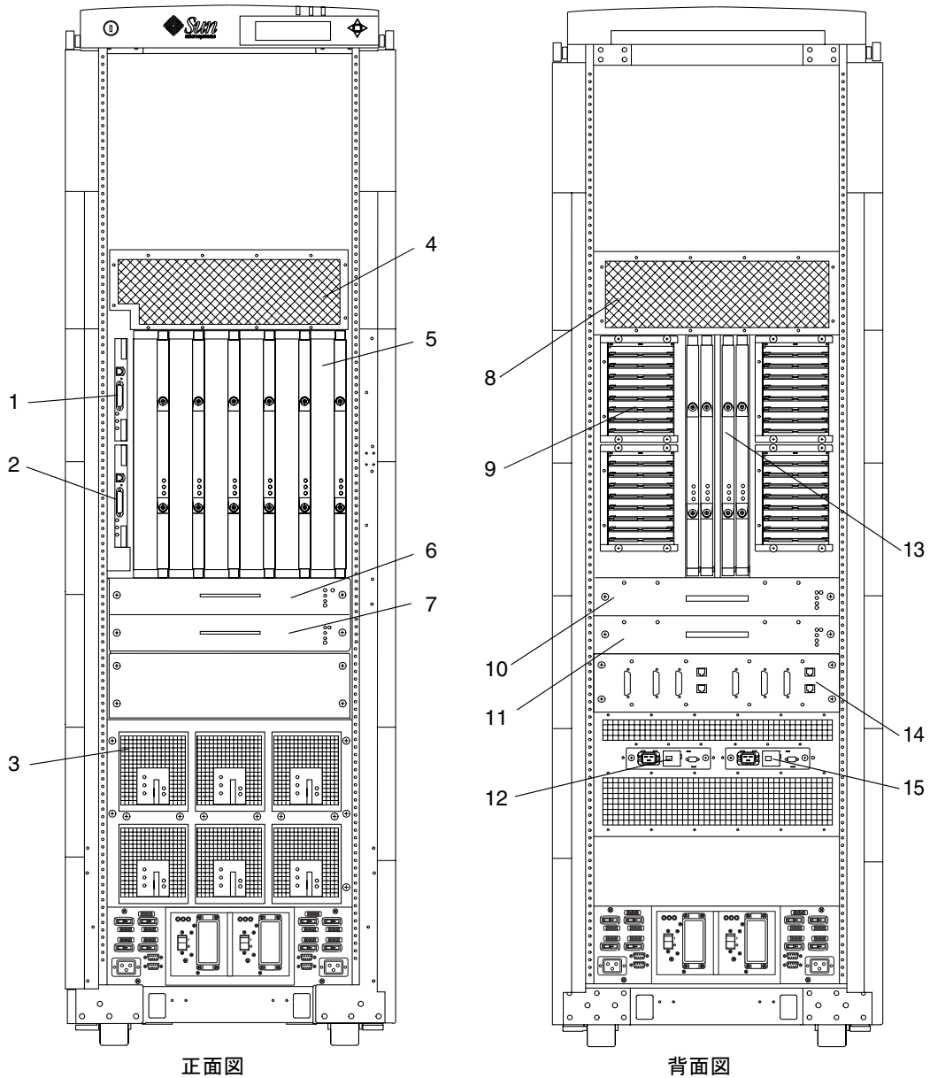
図 C-1 Sun Fire E6900 システム (正面図および背面図)
