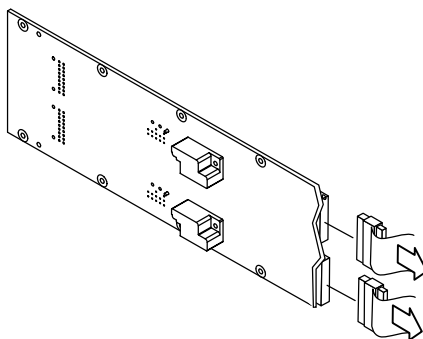
図 11-9 ファントレイセンタープレートケーブルの取り外し
