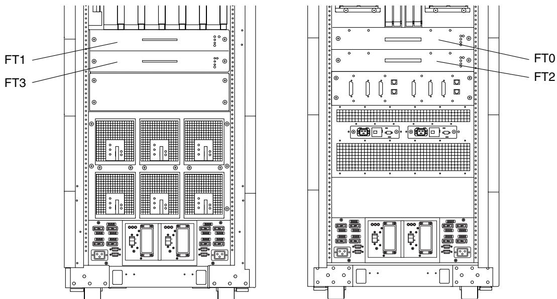
図 6-1 正面および背面のファントレー — Sun Fire E6900 システム
