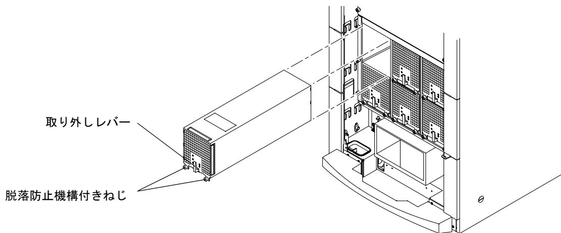
図 4-4 電源装置の取り外しまたは取り付け — Sun Fire E6900 システム
