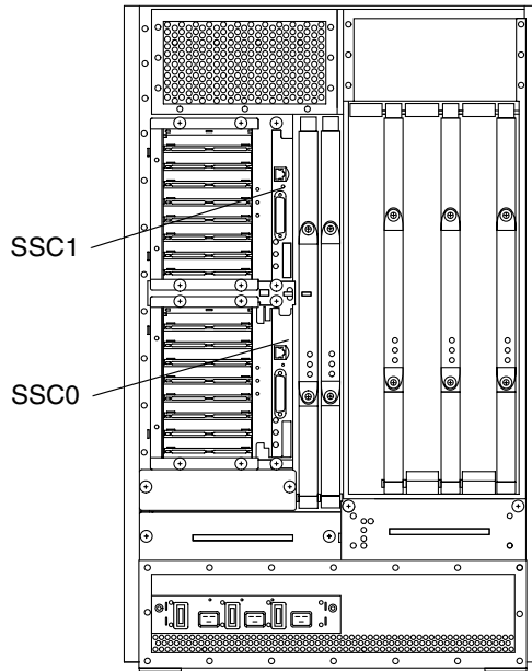
図 7-3 Sun Fire E4900 システムのシステムコントローラボードのスロット割り当て (背面図)
