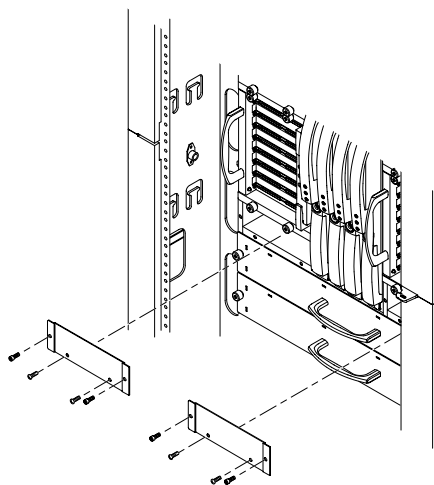
図 11-3 バスバーアクセスパネルの取り外し
