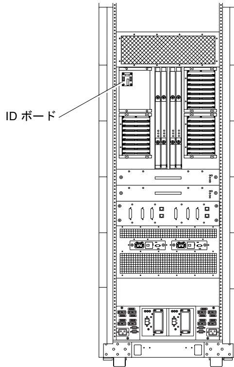
図 11-22 センタープレーンからの ID ボードの取り外し — Sun Fire E6900 システム
