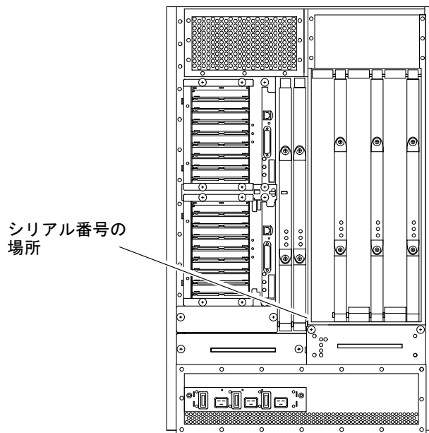
図 B-2 Sun Fire E4900 システムのシリアル番号の場所 (背面図)
