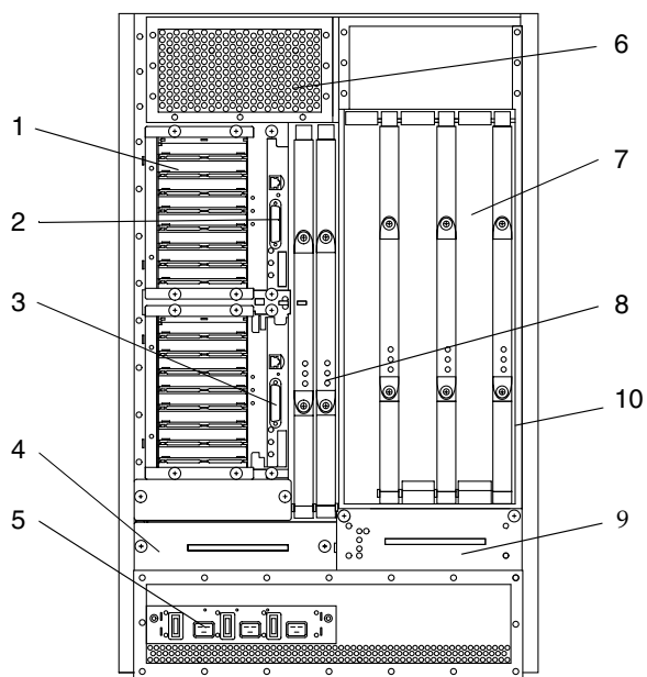
図 C-3 Sun Fire E4900 システム (背面図)
