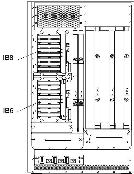
図 9-2 Sun Fire E4900 システムの I/O アセンブリ (背面図)
