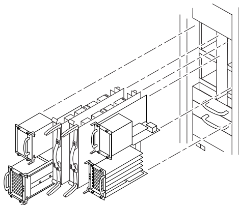
図 11-2 Sun Fire E6900 システムの正面からのすべてのコンポーネントの取り外し
