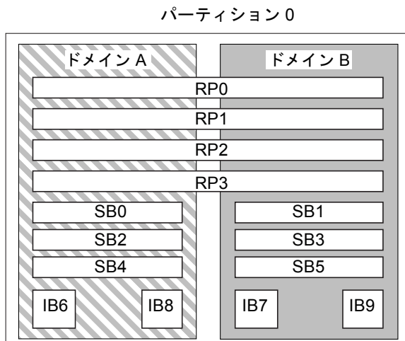
図 1-1 シングルパーティションモードの Sun Fire E6900 および 6800 システム
