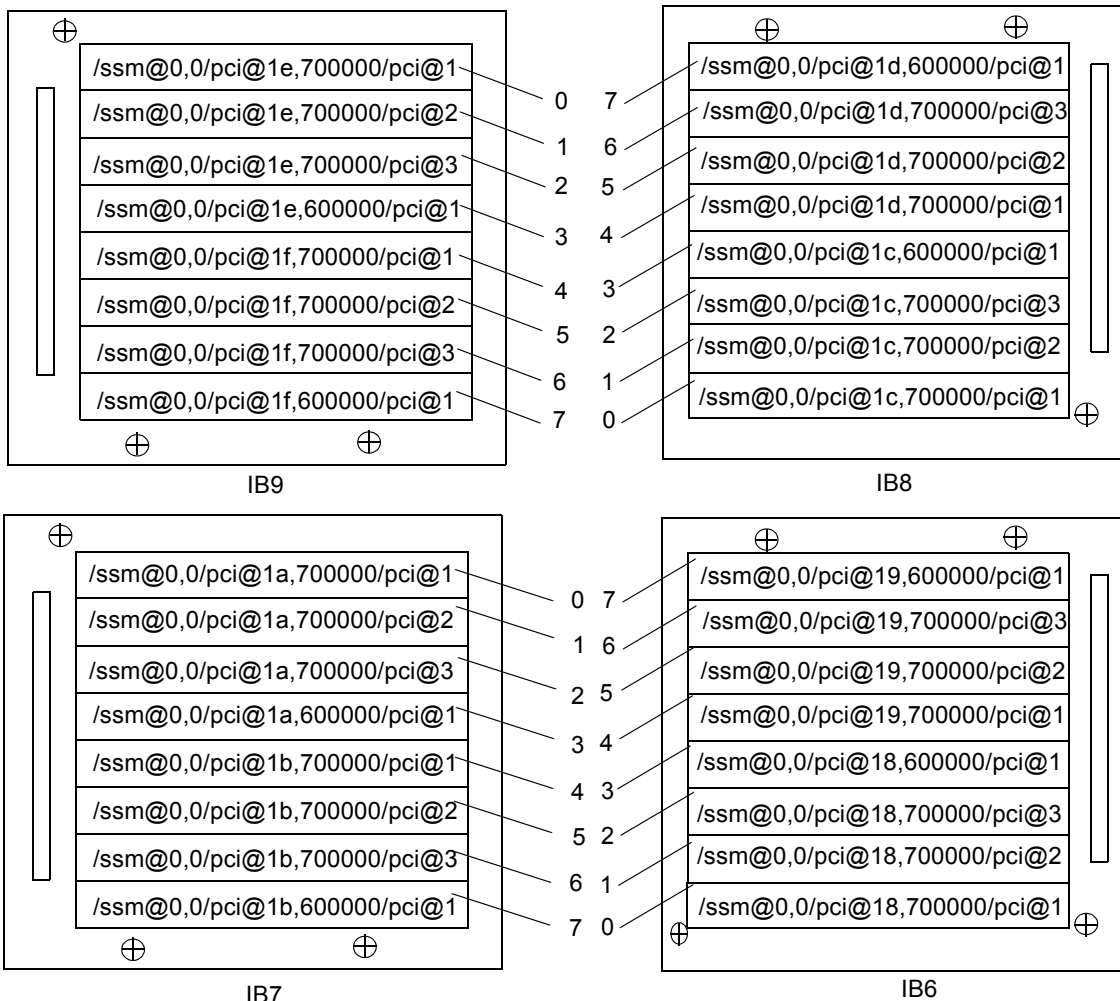
図 A-1 Sun Fire E6900 および 6800 システムの IB6～IB9 に対応する PCI 物理slotの番号
