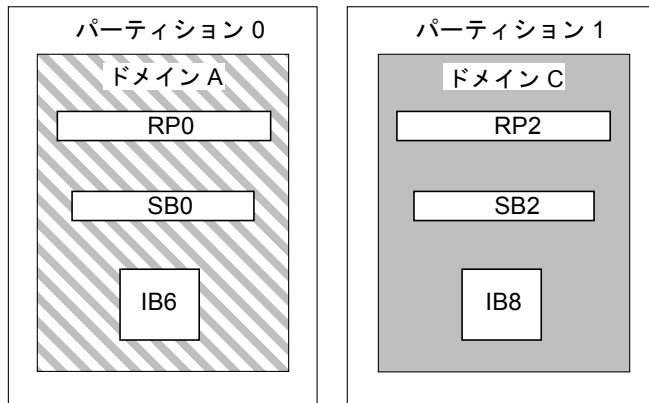
図 1-6 デュアルパーティションモードの Sun Fire 3800 システム
