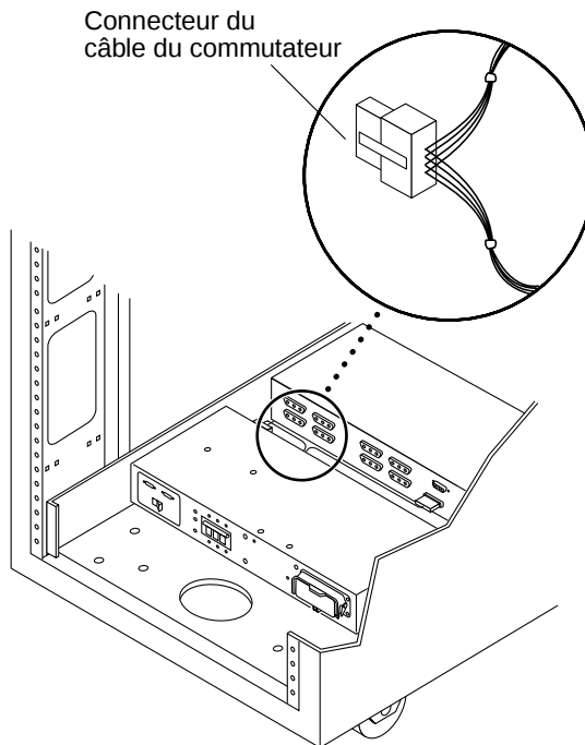
FIGURE 9-3 Connecteur du câble du commutateur
