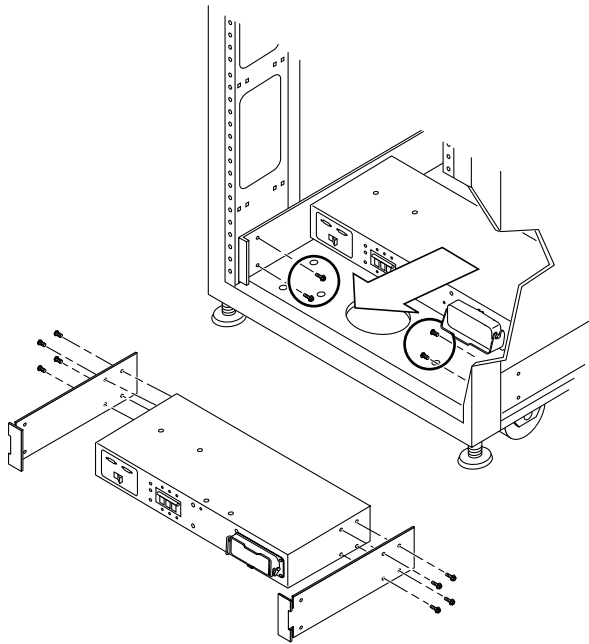
FIGURE 9-1 Retrait du séquenceur d'alimentation
