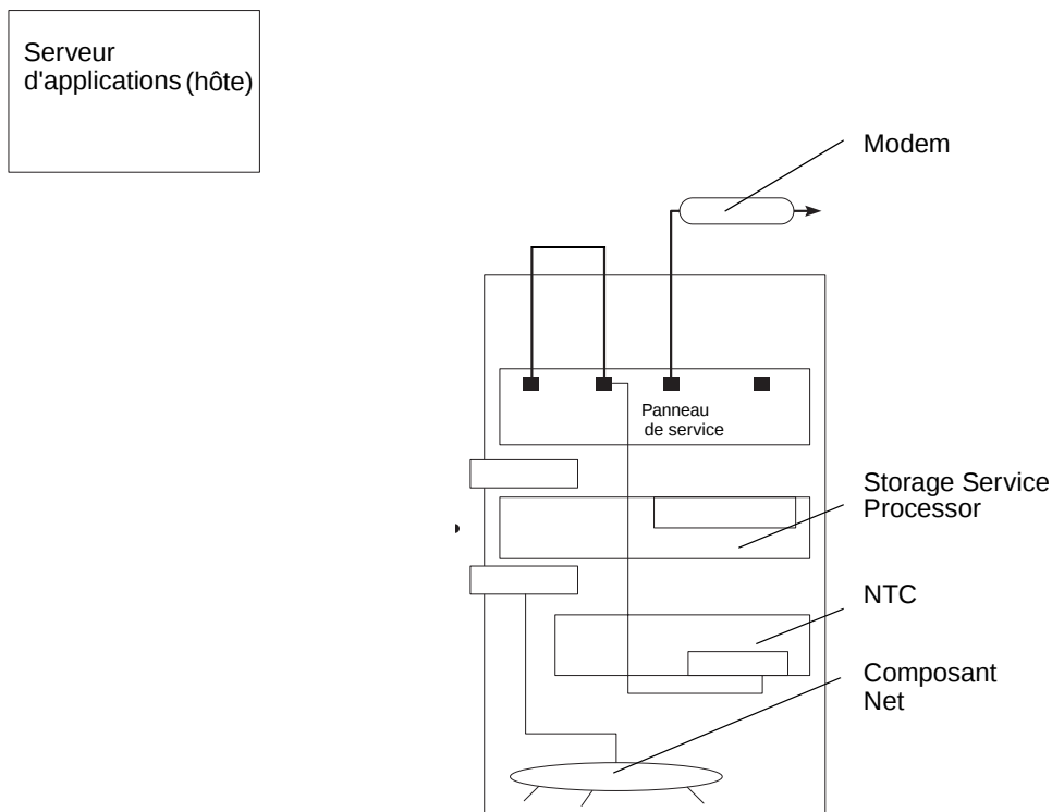
FIGURE 4-2 Maintenance à distance d'une unité sans hôte
