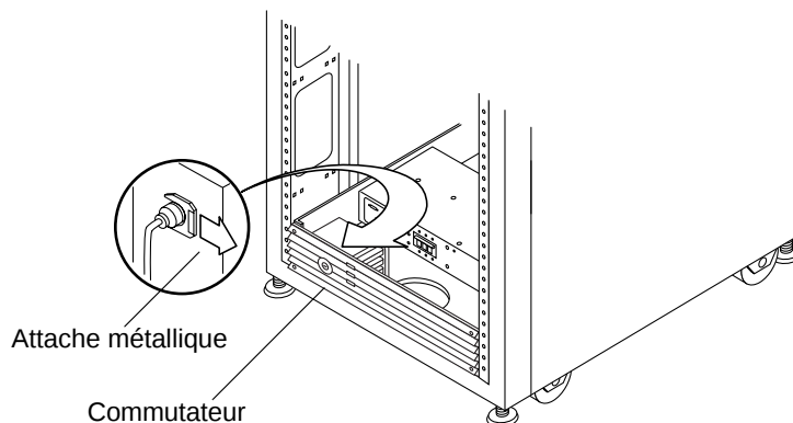
FIGURE 9-4 Retrait et réinstallation d'un commutateur
