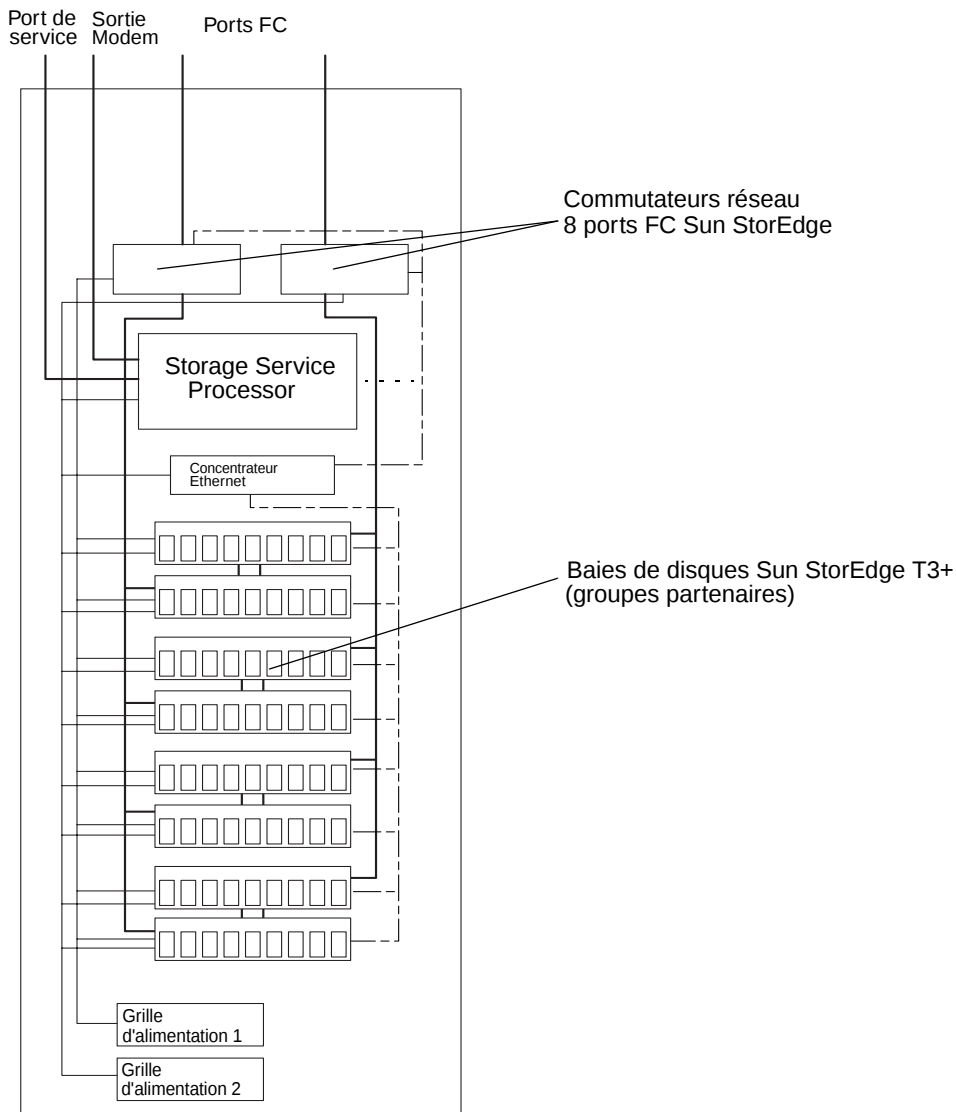
FIGURE 1-1 Système Sun StorEdge 3910
