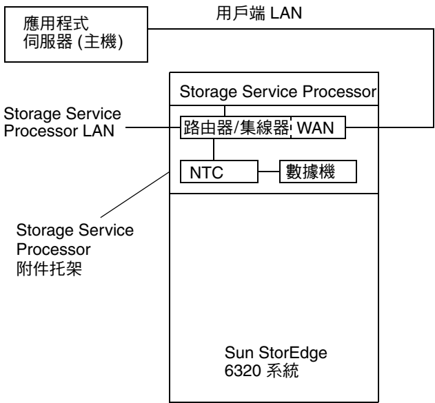
圖 1-6 無遠端服務的獨立 Sun StorEdge 6320 系統
