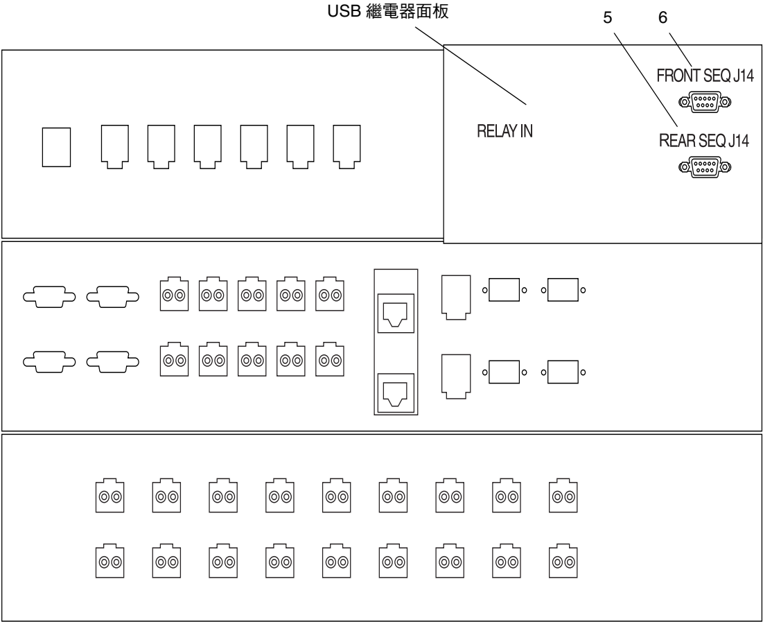
圖 4-13 Storage Service Processor 服務面板接頭背面圖
