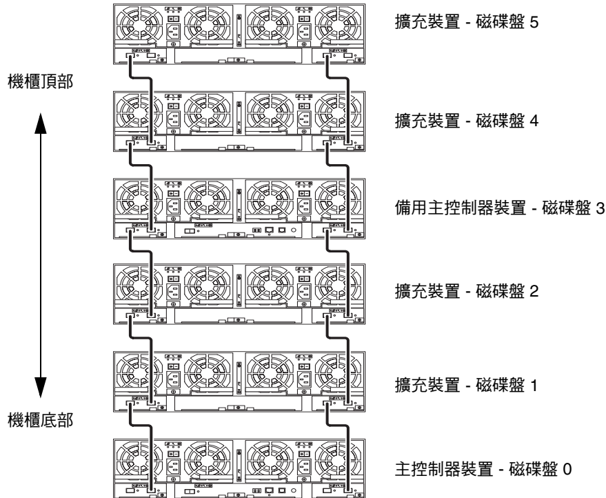
圖 4-16 2×6 HA 組態與相應的磁碟盤編號
