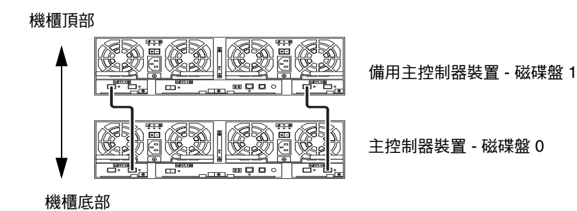
圖 4-14 2×2 HA 組態與相應的磁碟盤編號
