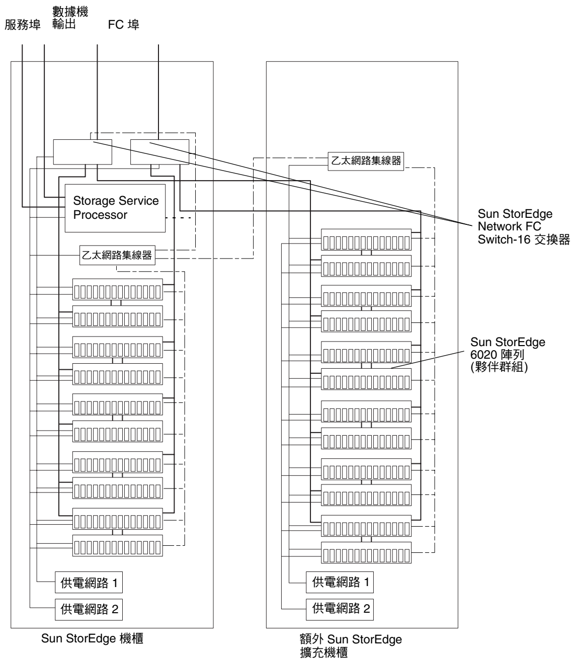
圖 1-3 Sun StorEdge 6320 系統
