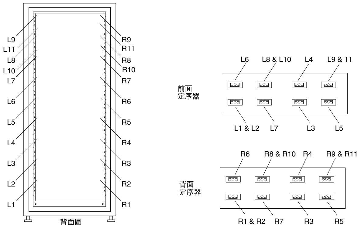
圖 4-6 電源線佈線
