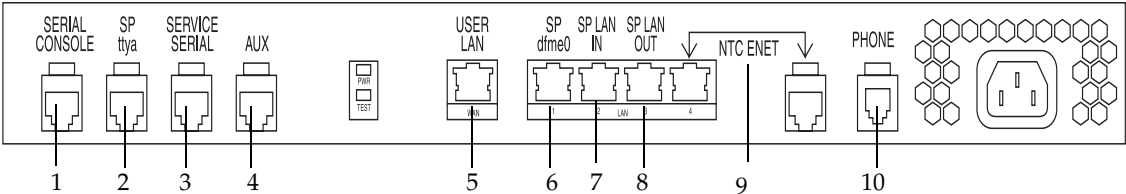
圖 4-17 Storage Service Processor 附件托架連線
