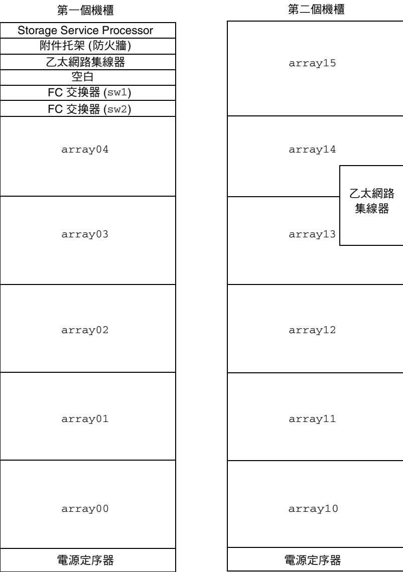
圖 1-5 Sun StorEdge 6320 系統背面圖
