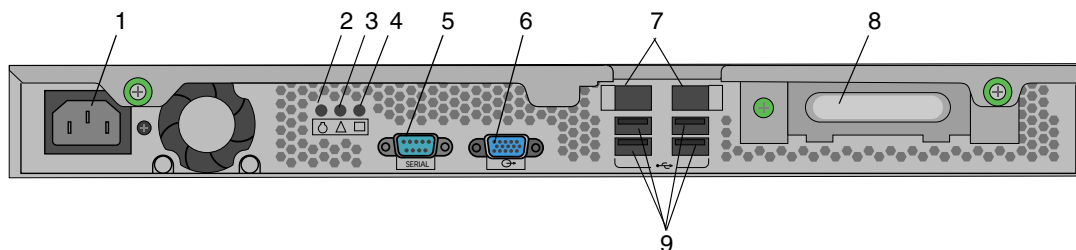
图 1-14 背面板
