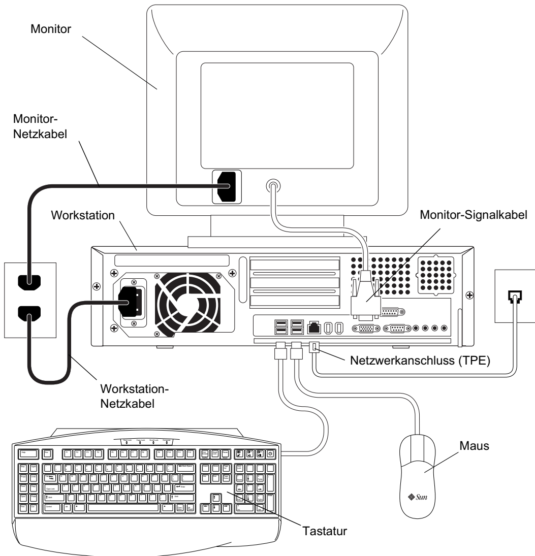
ABBILDUNG 4-2 Abtrennen externer Geräte von der Workstation
