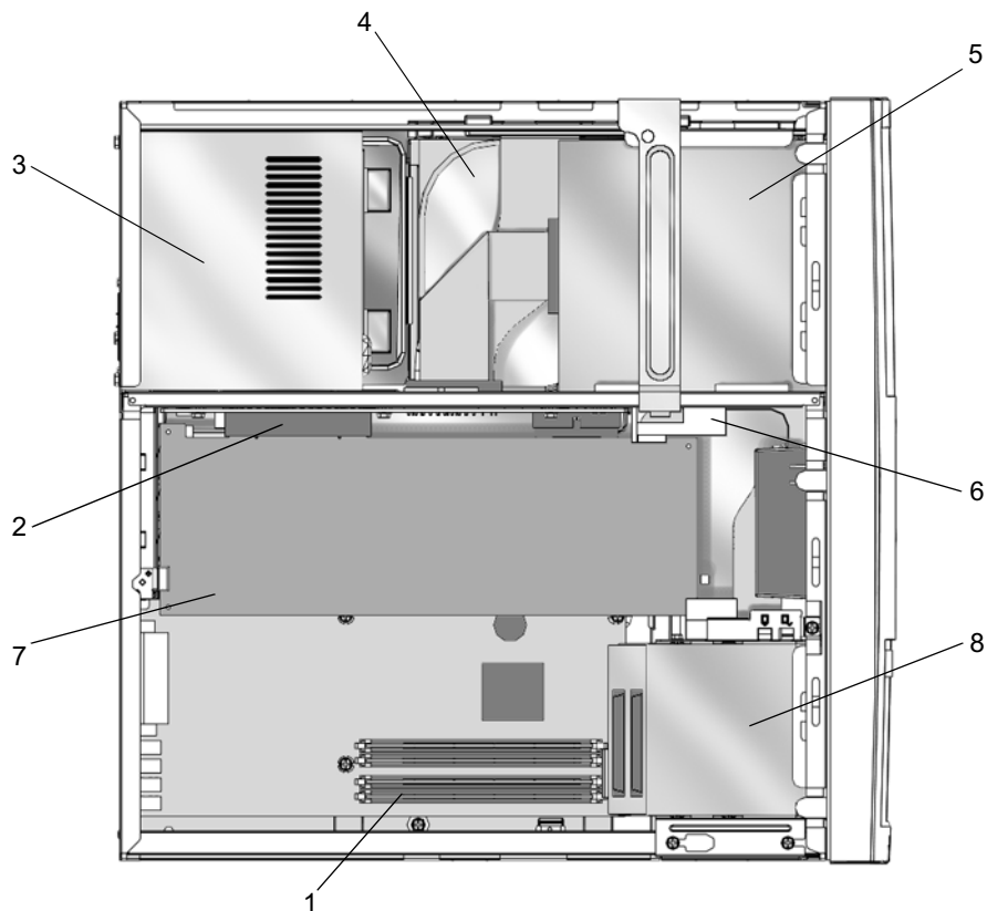
ABBILDUNG 4-5 Interner Aufbau der Workstation (Ansicht von oben mit abgenommener Abdeckung)
