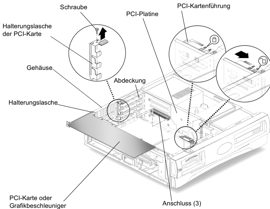
ABBILDUNG 4-8 Installieren einer PCI-Karte oder eines Grafikbeschleunigers
