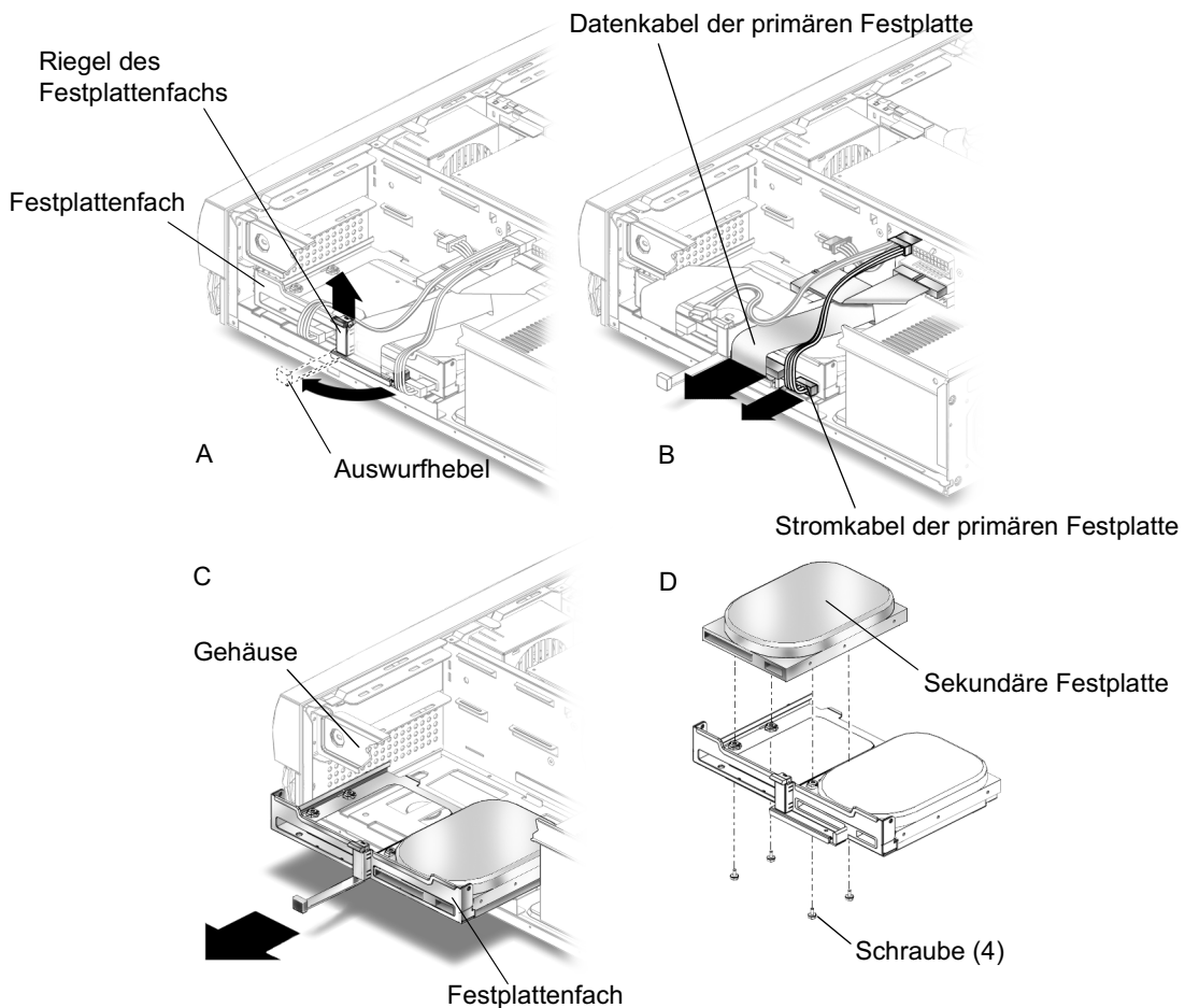
ABBILDUNG 4-11 Installieren einer sekundären Festplatte
