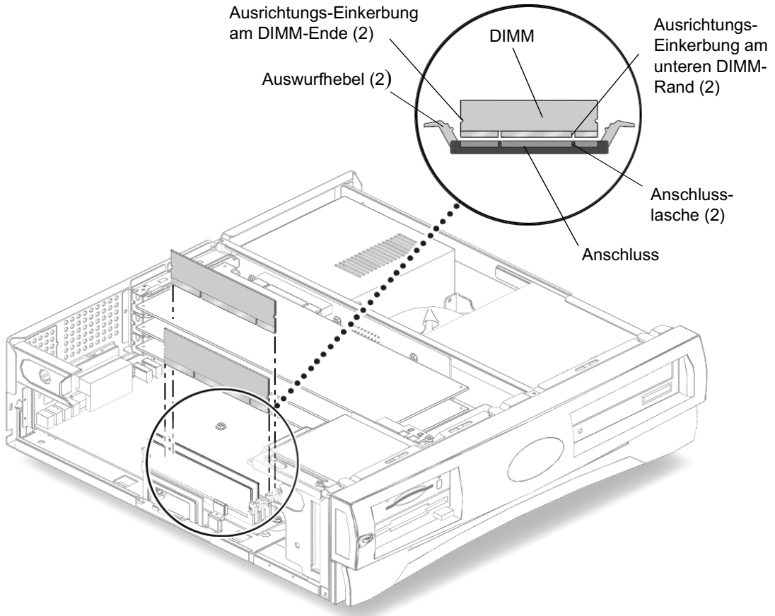
ABBILDUNG 4-7 Installieren der DIMMs
