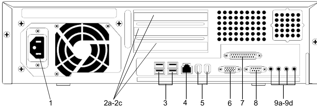
ABBILDUNG 1-4 Übersicht über die Rückseite
