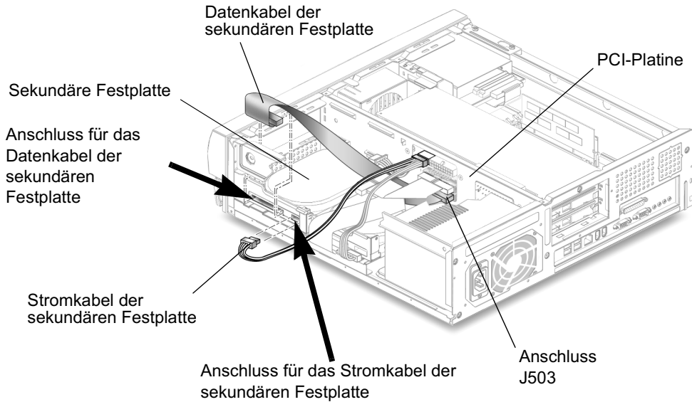
ABBILDUNG 4-12 Wiederanschließen der Kabel der sekundären Festplatte
