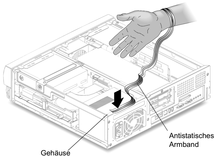
ABBILDUNG 4-4 Anlegen des antistatischen Armbands
