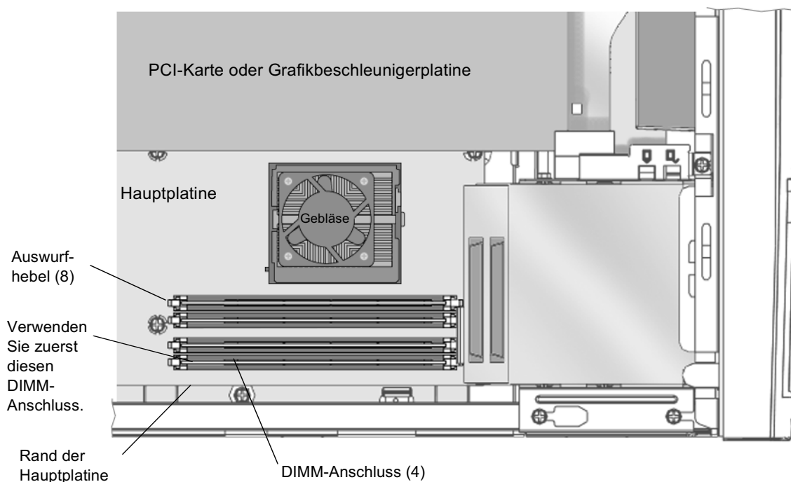
ABBILDUNG 4-6 DIMM-Installationsreihenfolge (Ansicht von oben auf die Workstation mit abgenommener Abdeckung)
