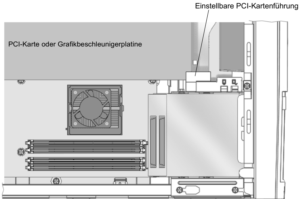
ABBILDUNG 4-9 PCI-Kartenführung
