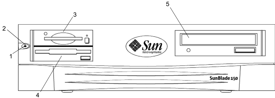
ABBILDUNG 1-3 Übersicht über die Vorderseite
