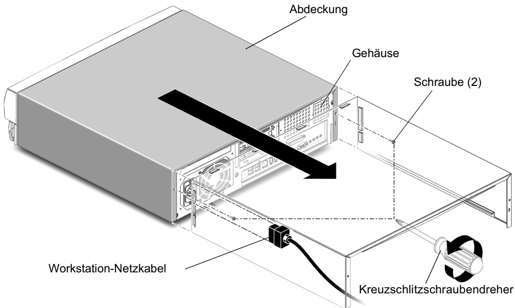
ABBILDUNG 4-3 Abnehmen der Workstation-Abdeckung
