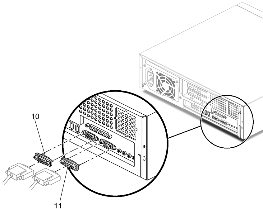
ABBILDUNG 1-5 Videoanschlussverlängerung und Verlängerung für den seriellen Anschluss
