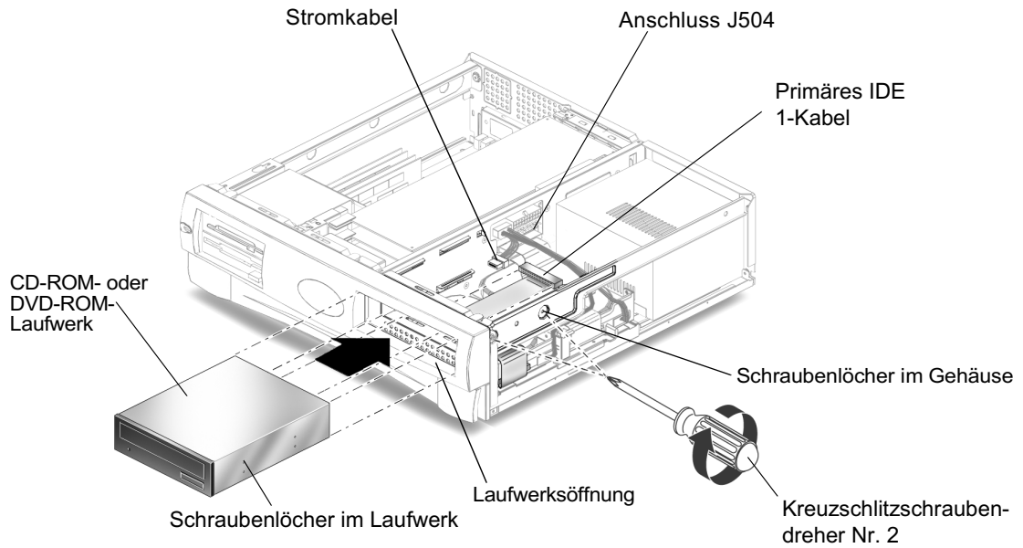
ABBILDUNG 4-10 Installieren eines CD-ROM- oder DVD-ROM-Laufwerks
