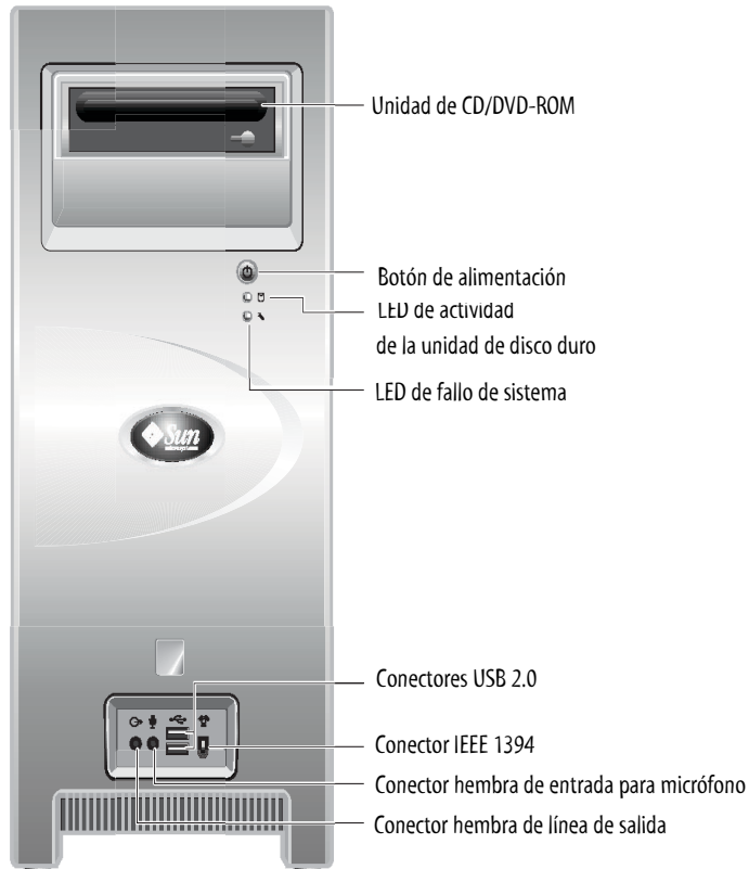
FIGURA 1-2 Panel anterior
