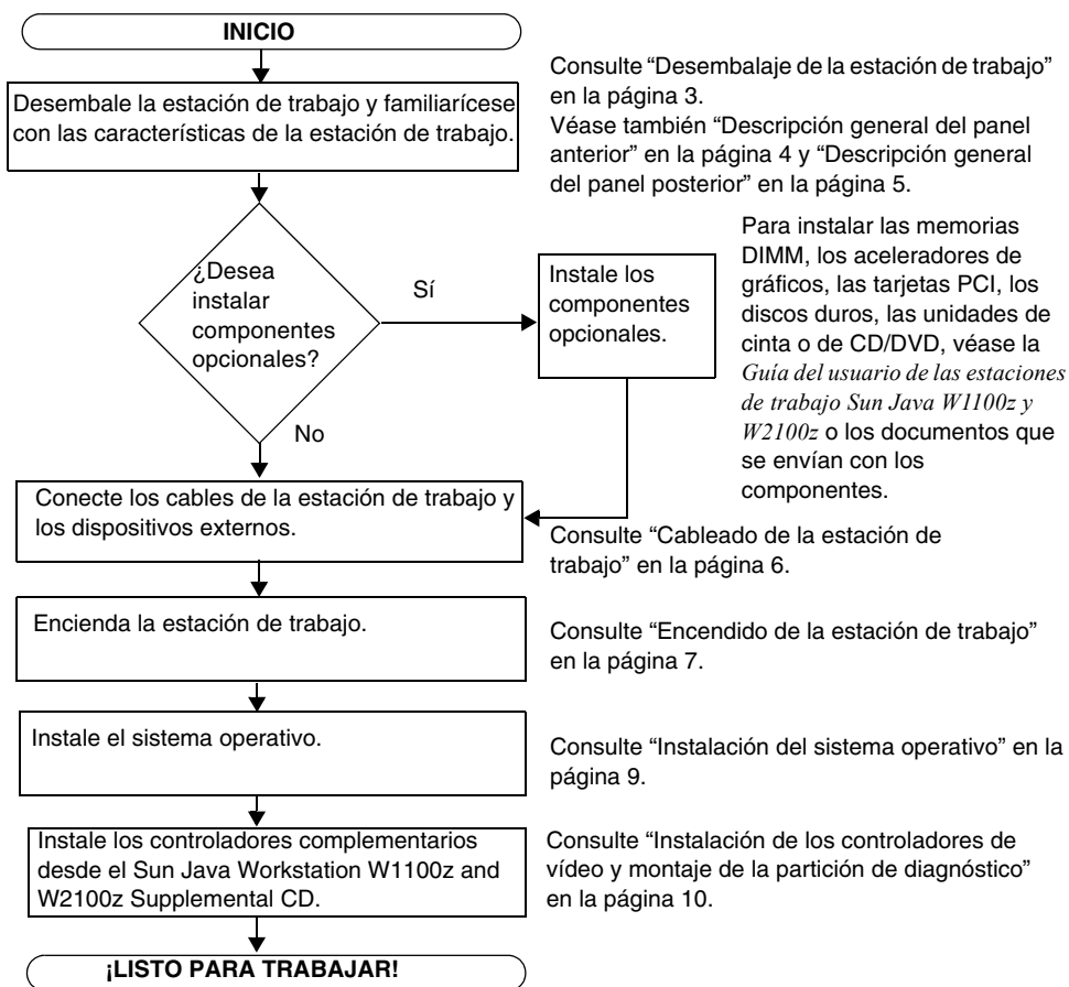
FIGURA 1-1 Proceso para la instalación de las estaciones de trabajo Sun Java W1100z y W2100z
