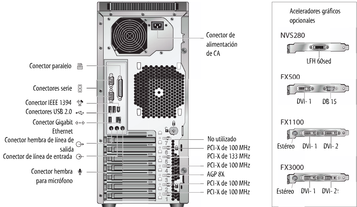
FIGURA 1-3 Panel posterior
