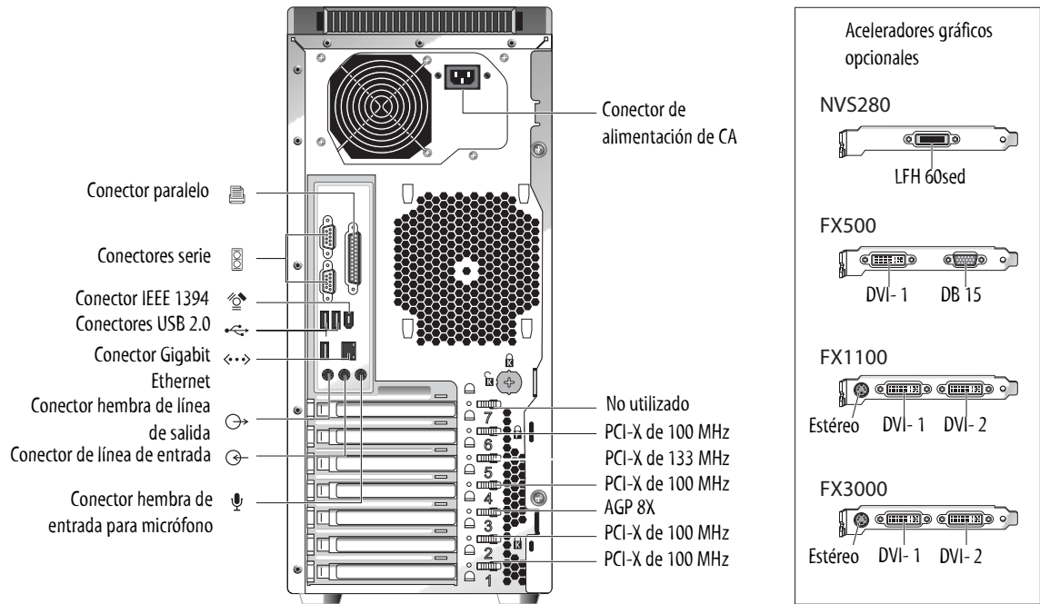
FIGURA 1-2 Panel posterior
