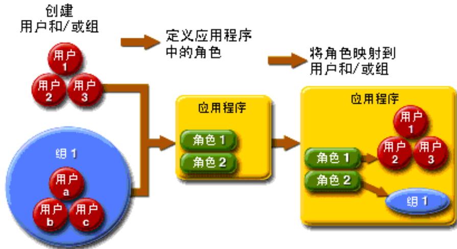
图 9-1 角色映射
