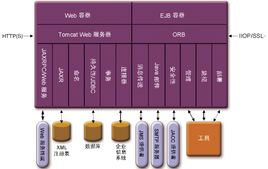
图 1-1 Application Server 体系结构
