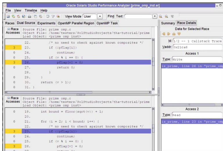
图 2-2 prime_omp.c 中检测到的数据争用的源代码
