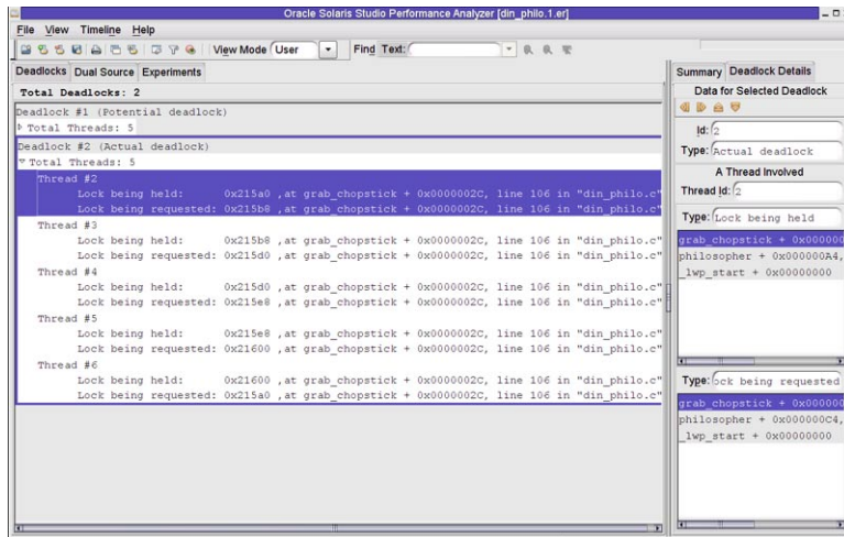
图 3-2 din_philo.c 中检测到的死锁
