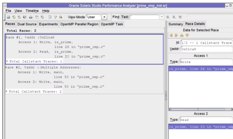
图 2-1 prime_omp.c 中检测到的数据争用
