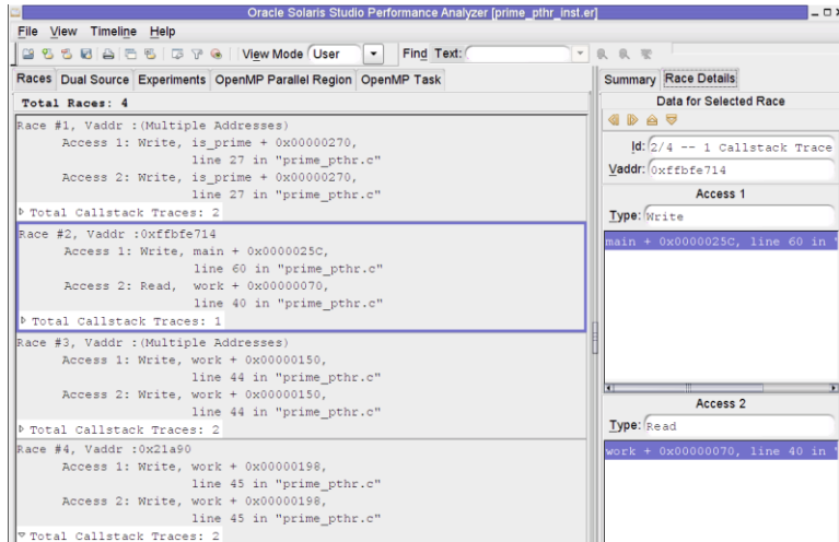
图2-3 prime_pthr.c 中检测到的数据争用
