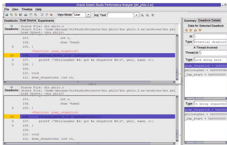
图 3-3 din_philo.c 中的潜在死锁
