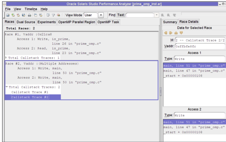
图 2-5 "Races" (争用) 标签 (包含 prime_omp.c 的调用栈跟踪)
