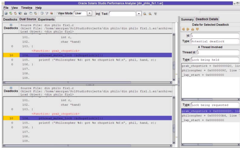
图 3-6 误报的潜在死锁的源代码
