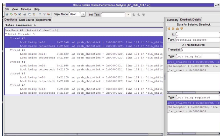
图 3-5 误报的潜在死锁
