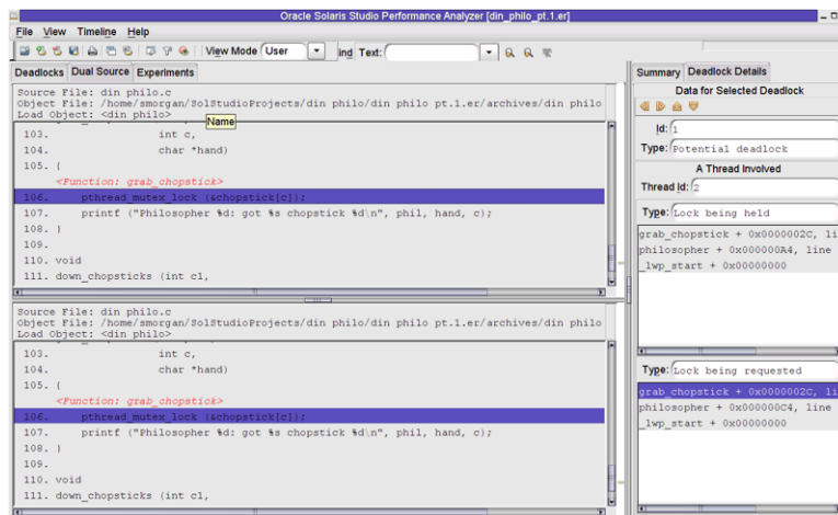
图 3-4 din_philo.c 中的潜在死锁
