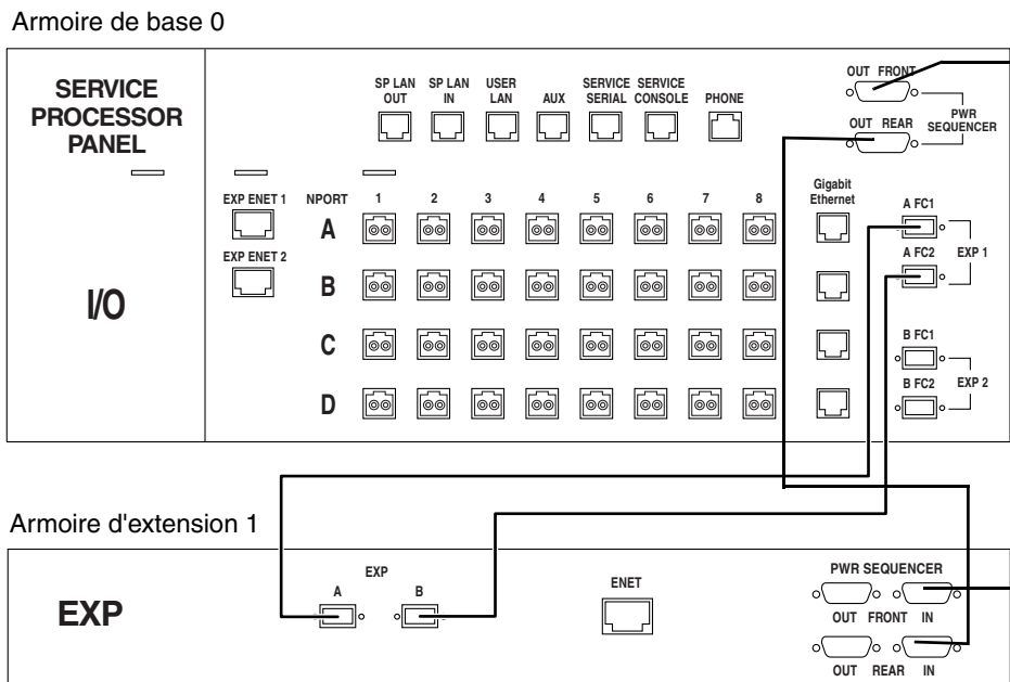
FIGURE 5 Câblage du séquenceur d'alimentation et câblage Ethernet entre un nouveau panneau de service de l'armoire de base 0 et l'armoire d'extension 1
