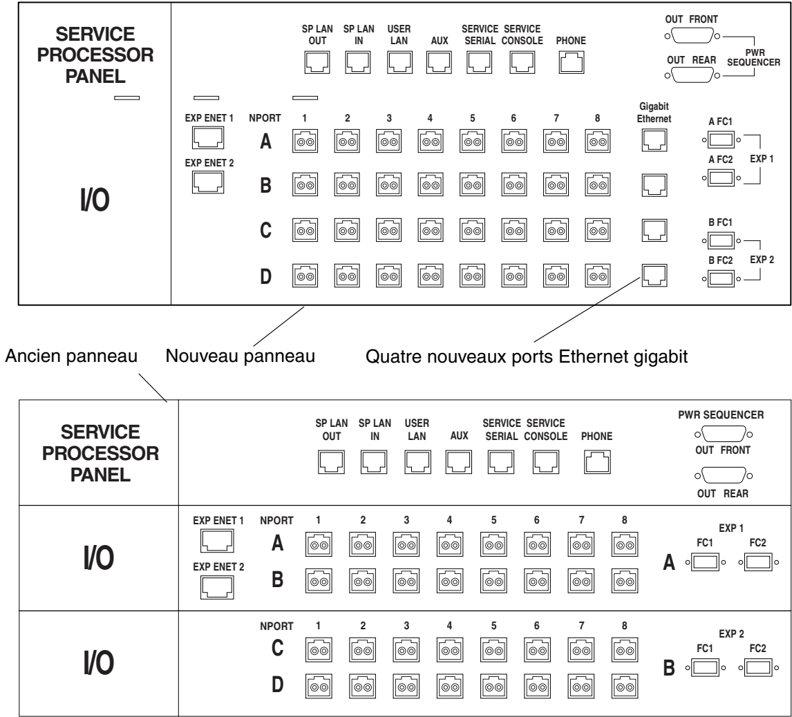
FIGURE 1 Ancien et nouveaux panneaux de service
