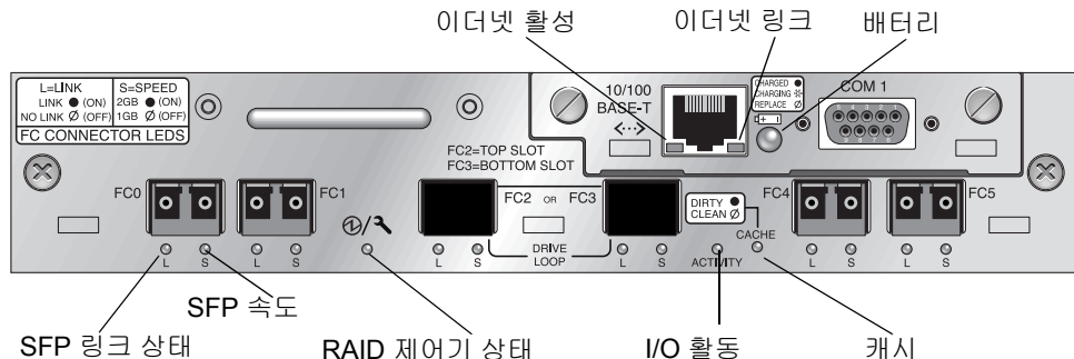
그림 7-3 Sun StorEdge 3510 FC 어레이 I/O 제어기 모듈 및 배터리 모듈 LED
