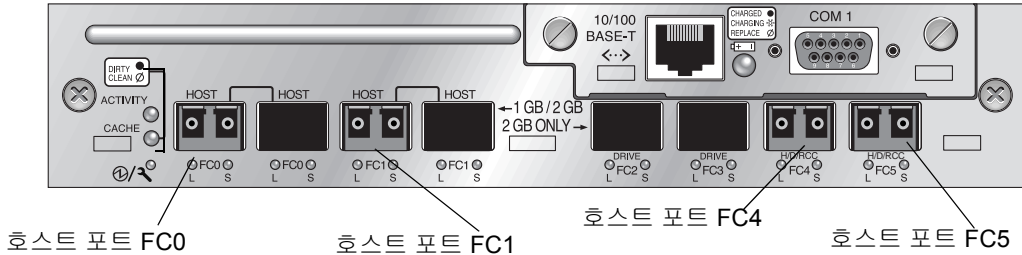
그림 4-14 Sun StorEdge 3511 FC 어레이 기본 단일 제어기의 SFP 배치
