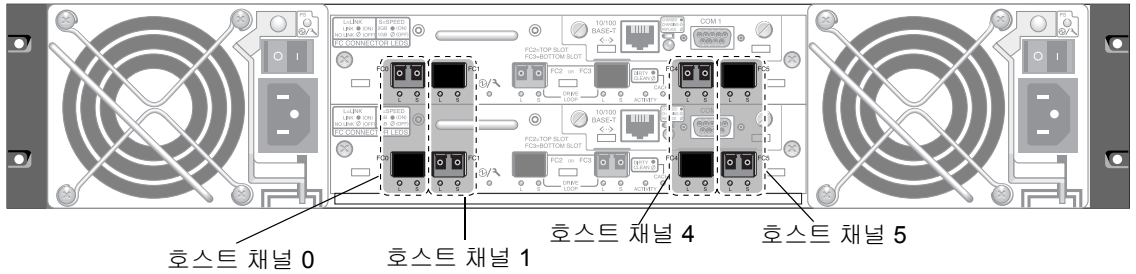
그림 4-9 이중 제어기 Sun StorEdge 3510 FC 어레이의 호스트 채널
