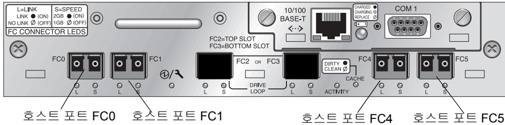
그림 4-13 Sun StorEdge 3510 FC 어레이 기본 단일 제어기의 SFP 배치
