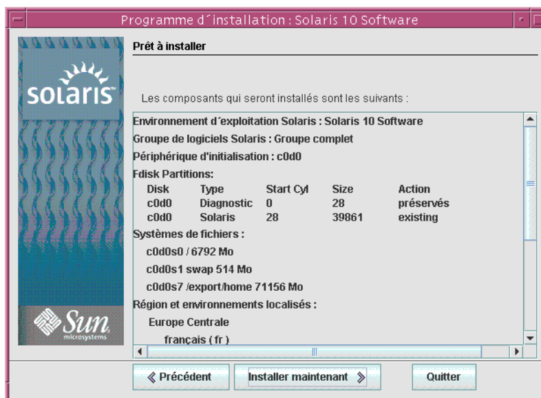
FIGURE 2-12 Écran Prêt pour l'installation de Solaris
