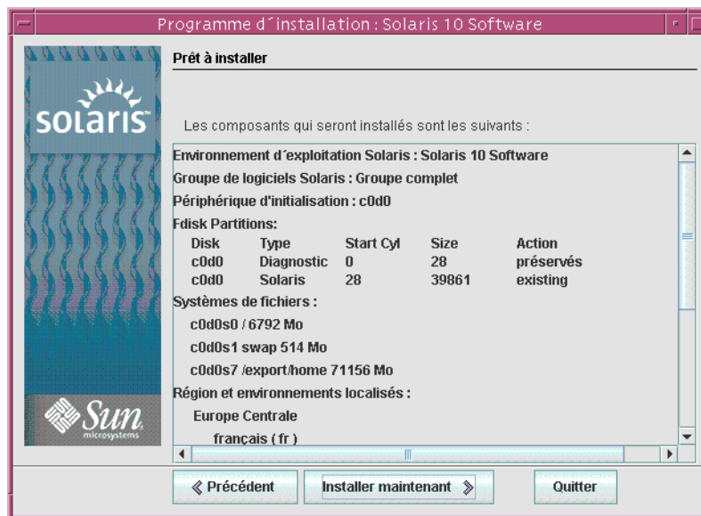
FIGURE 2-8 Écran Prêt pour l'installation de Solaris
