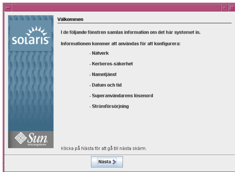
FIGUR 2-9 Välkomstskärm för Solaris GUI installationsprogram
