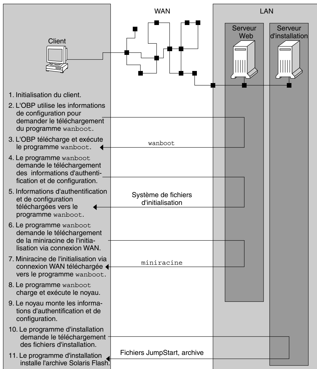
FIGURE 11-1 Déroulement des événements lors d'une installation et initialisation via connexion WAN
