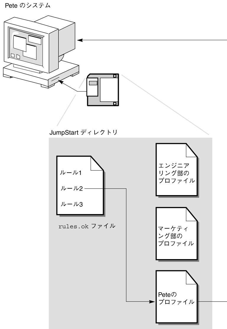
図 2-1 カスタム JumpStart インストールの流れ: ネットワークに接続されていない場合の例
