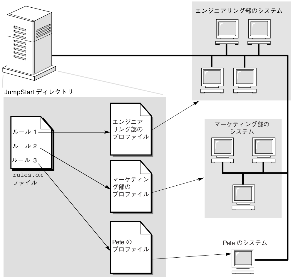
図 2-2 カスタム JumpStart インストールの流れ: ネットワークに接続されている場合の例
