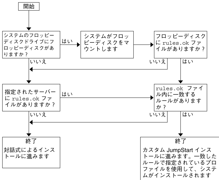
図 2-3 カスタム JumpStart インストール実行時の流れ
