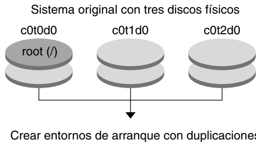
FIGURA 10-1 Desconexión y modernización de uno de los lados de un volumen RAID-1 (duplicación)
