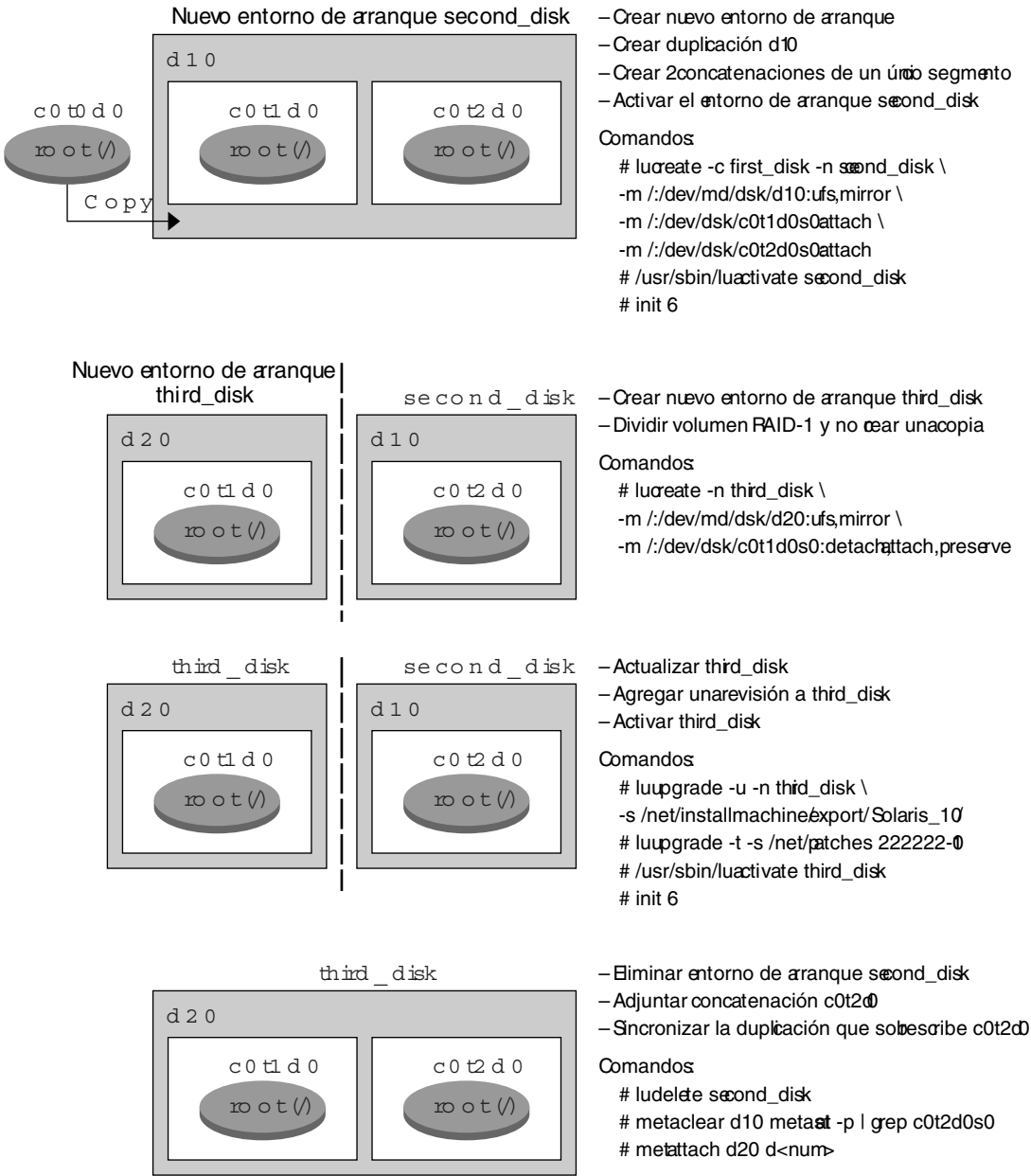
FIGURA 10-2 Desconexión y modernización de uno de los lados de un volumen RAID-1 (duplicación) (continuación)
