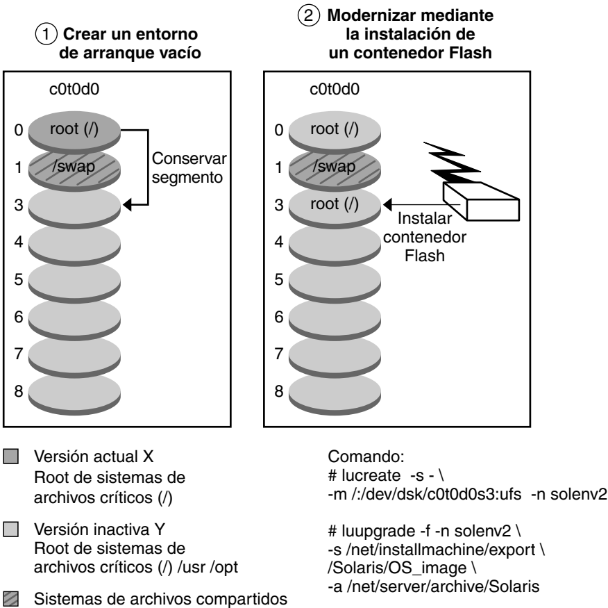
FIGURA 2–8 Instalación de un contenedor de Solaris Flash en un único disco
