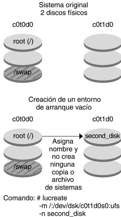
FIGURA 10-3 Creación de un entorno de arranque vacío
