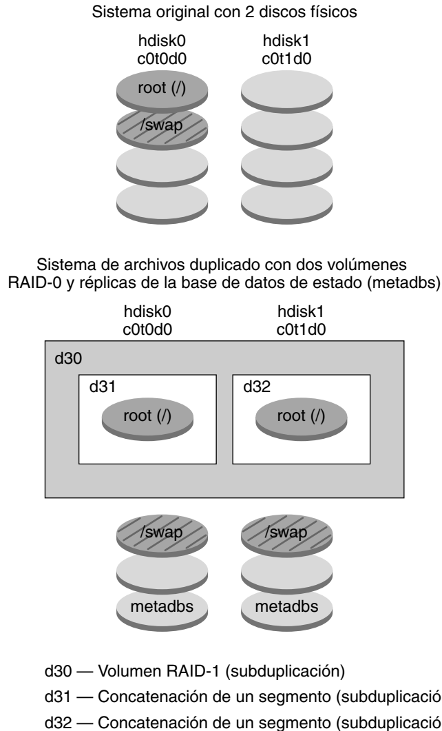
FIGURA 8-2 Disposición de discos en volúmenes RAID-1
