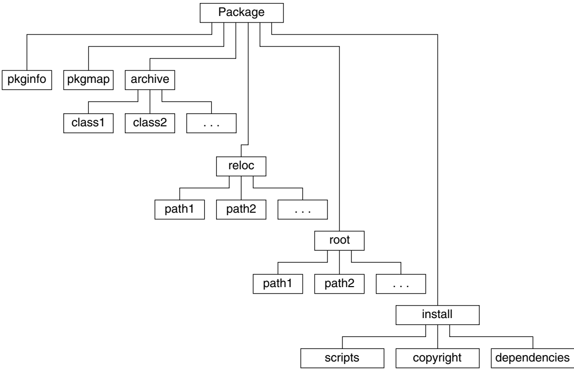
FIGURA 6-2 Estructura de directorios de paquetes de archivos de almacenamiento
