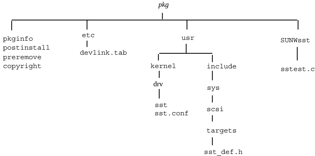
FIGURA 5-1 Estructura jerárquica de directorios de paquetes
