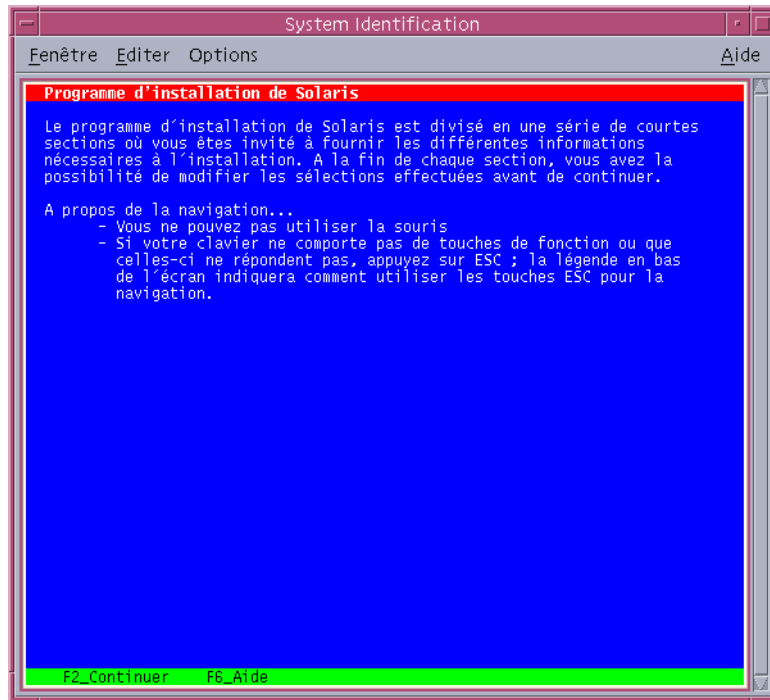
FIGURE 2-6 Écran d'accueil du programme d'installation en mode texte de Solaris
