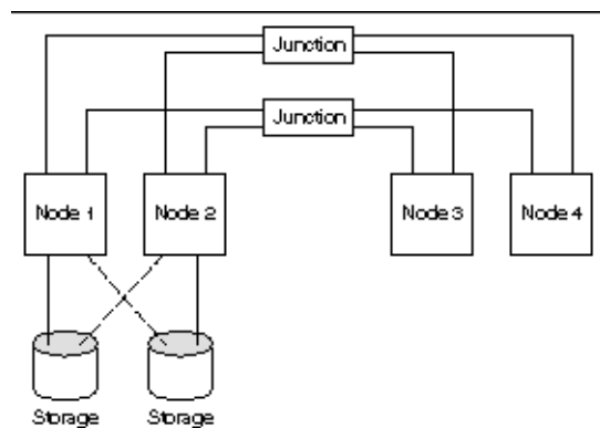
그림 2-3 SPARC: 쌍+N 토폴로지
