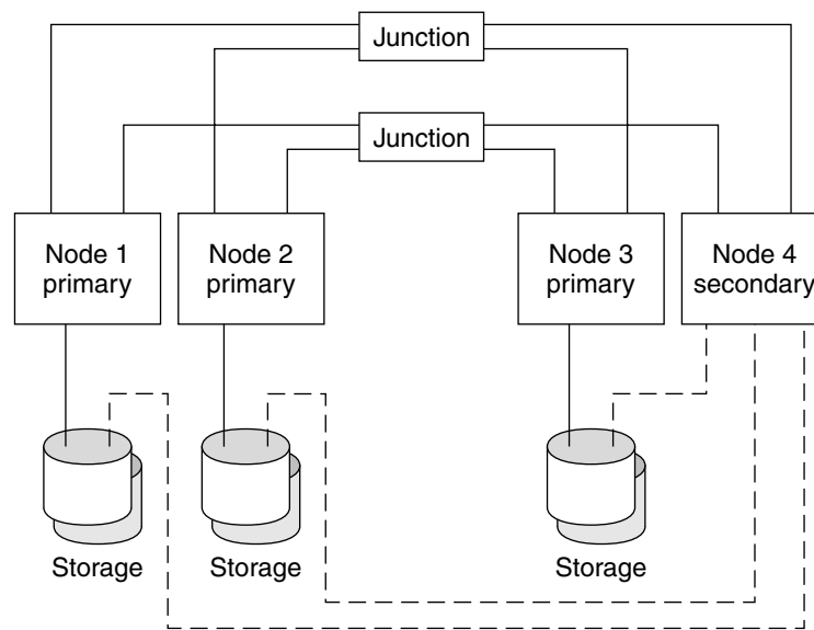
그림 2-4 SPARC: N+1 토폴로지
