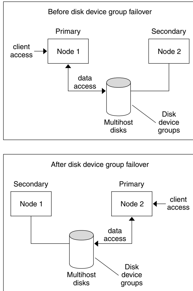
그림 3-1 디스크 장치 그룹 페일오버
