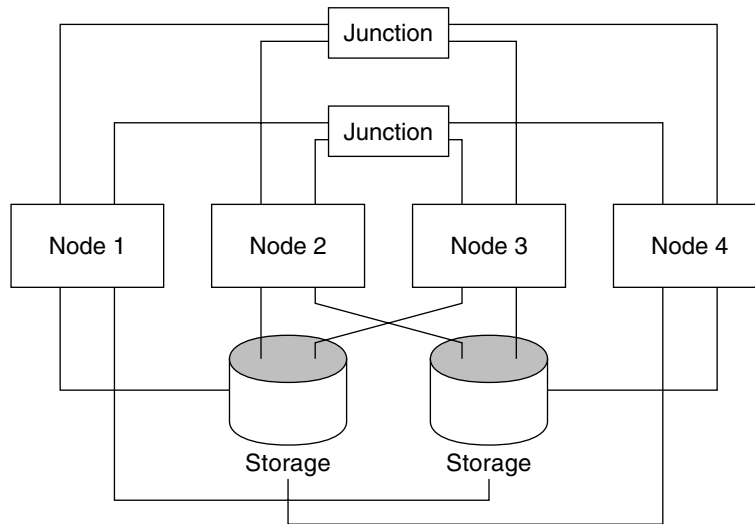
그림 2-5 SPARC: N*N 토폴로지
