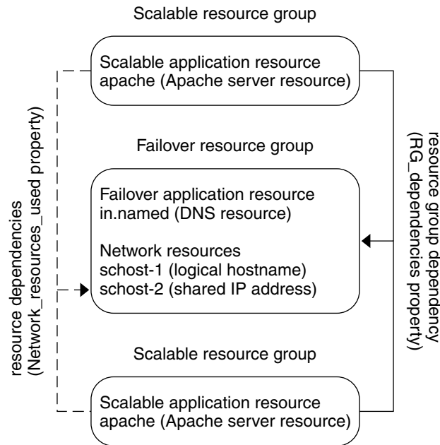
그림 3-6 SPARC: 페일오버 및 확장 가능 자원 그룹의 예
