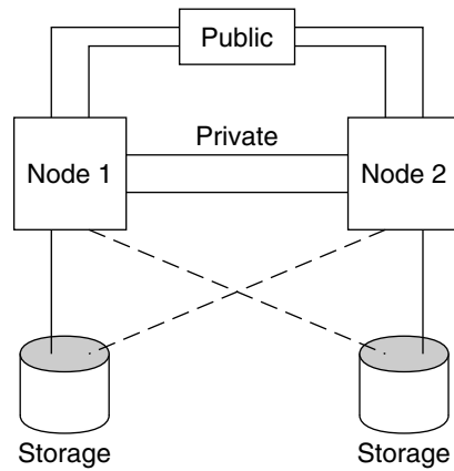
그림 2-6 x86: 클러스터 쌍 토폴로지
