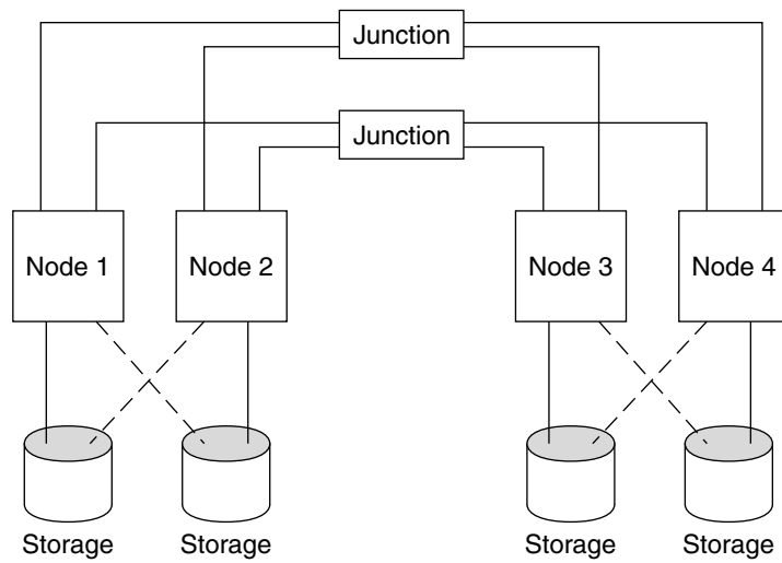
그림 2-2 SPARC: 클러스터 쌍 토폴로지
