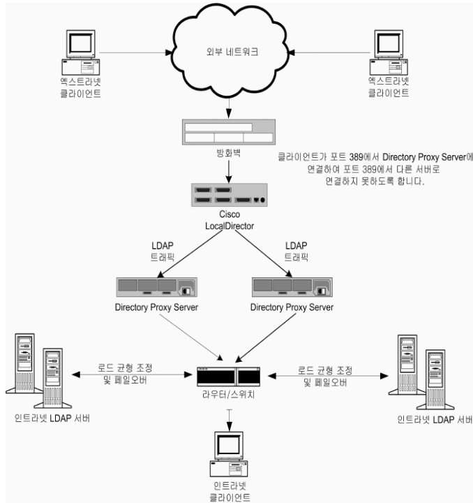
그림 2-4 단일 방화벽이 있는 Directory Proxy Server 설정
