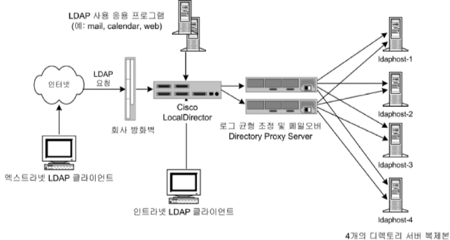
그림 2-1 내부 고가용성 구성
