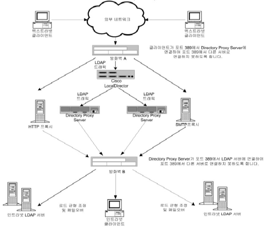
그림 2-5 두 방화벽이 있는 Directory Proxy Server 설정
