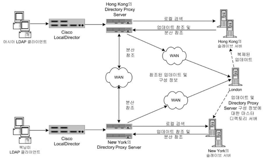
그림 2-2 분산 LDAP 디렉토리 인프라
