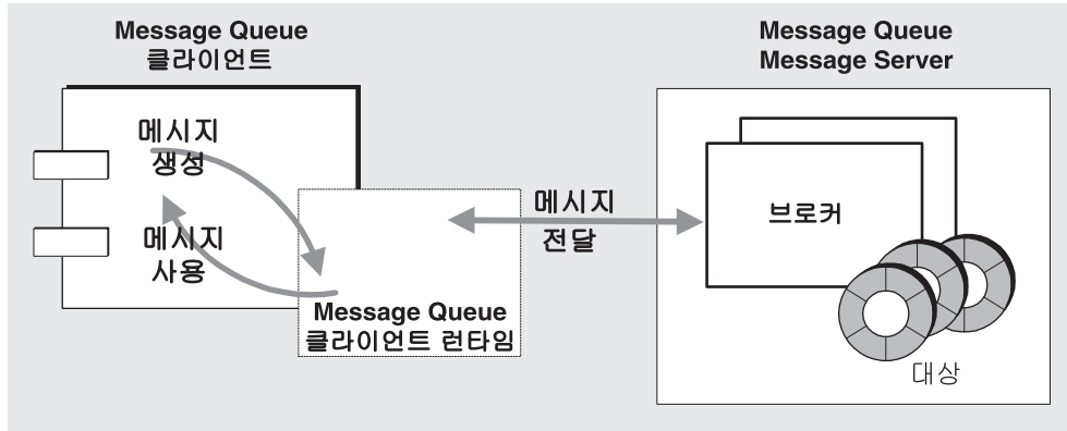
그림 11-5 메시지 작업
