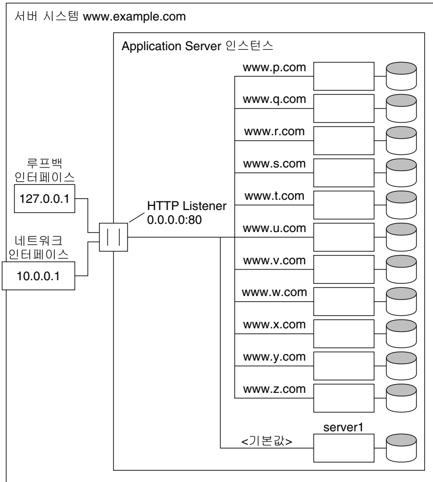
그림 15-5 다중 호스팅
