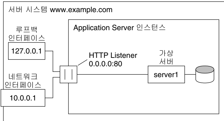
그림 15-1 기본 구성
