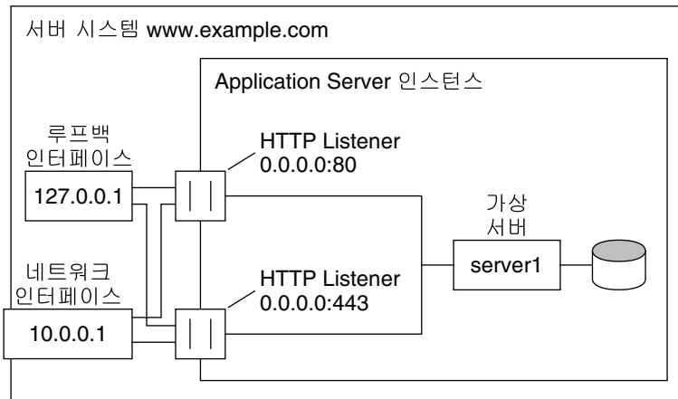
그림 15-2 보안 서버
