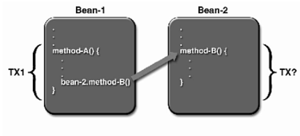
그림 9-1 트랜잭션 속성
