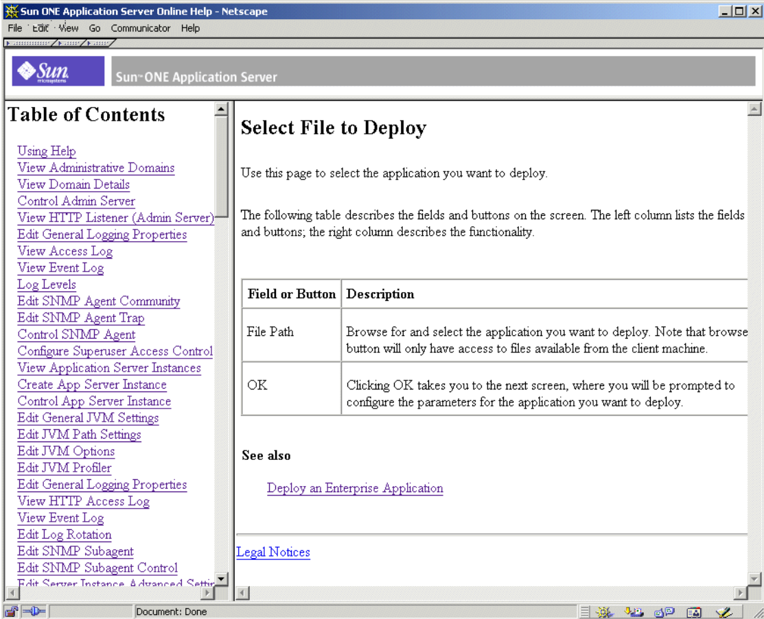
그림 1-5 온라인 도움말
