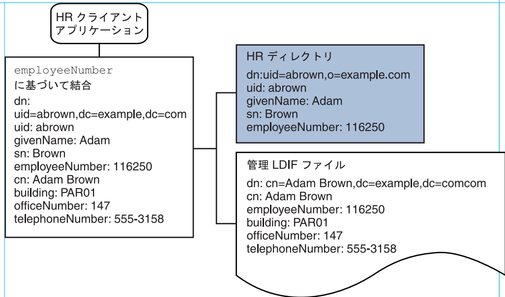
図 23-4 LDAPディレクトリとLDIFファイルのデータの集約
