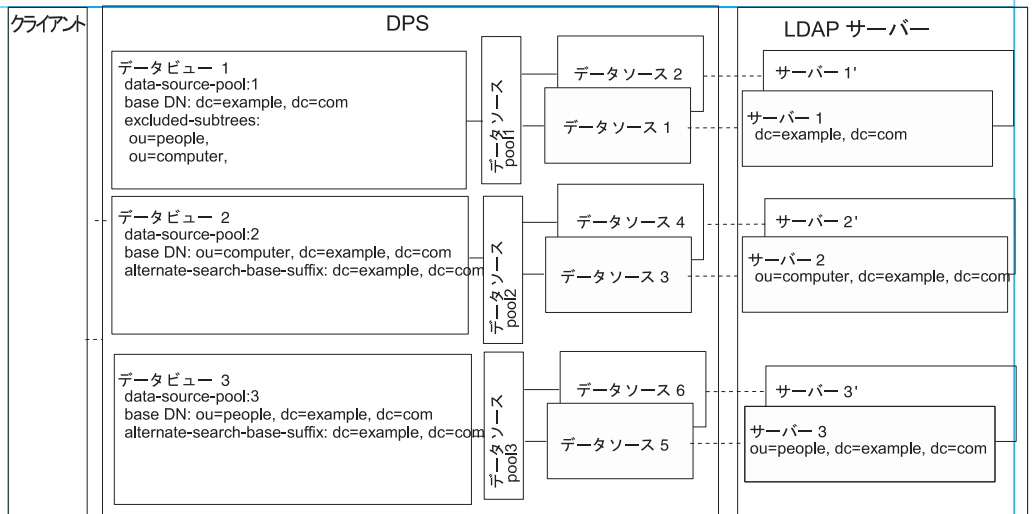
図 19-3 上位サブツリーと下位サブツリーが異なるデータソースに保存される場合に要求を経路指定する配備の例
