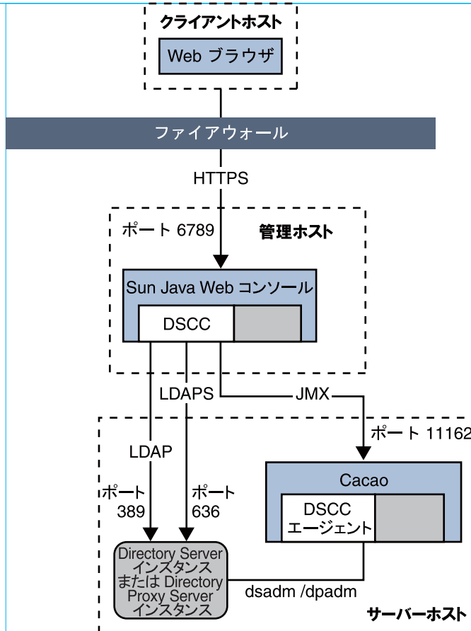
図 1-2 ネイティブパッケージ配布のインストール後の、別々のシステム上の管理ホストとサーバーホスト
