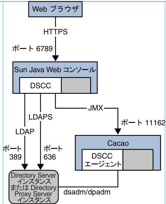
図1-1 ネイティブパッケージ配布のインストール後のポートとプロトコル
