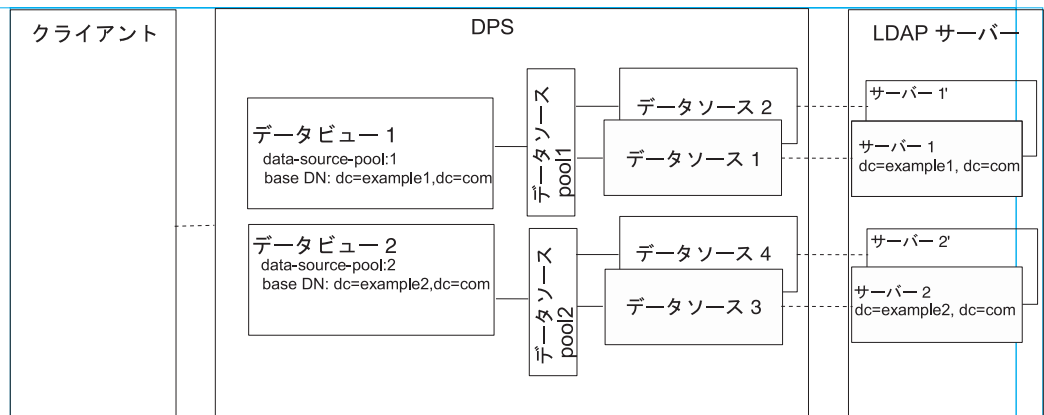
図 19-2 異なるサブツリーが異なるデータソースに保存されている場合に単一のアクセスポイントを提供する配備の例
