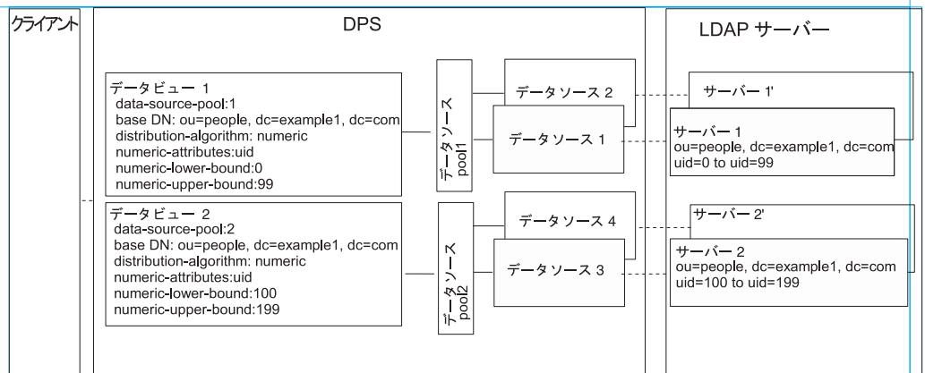
図 22-1 サブツリーの異なる部分が異なるデータソースに保存されている場合に単一のアクセスポイントを提供する配備の例
