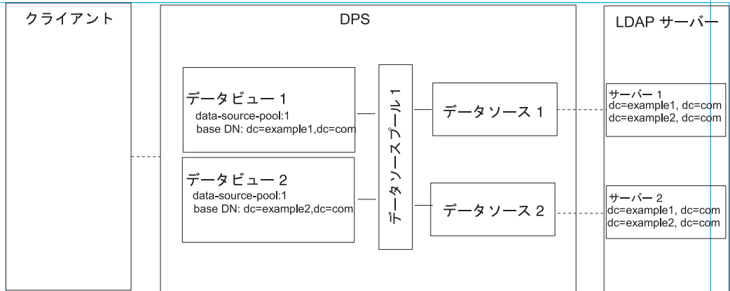
図 19-1 サブツリーの一覧が複数のデータ同等のデータソースに保存されると要求を経路指定する配備の例
