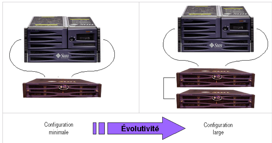
FIGURE 5 Architecture optimisée pour un serveur de bases de données
