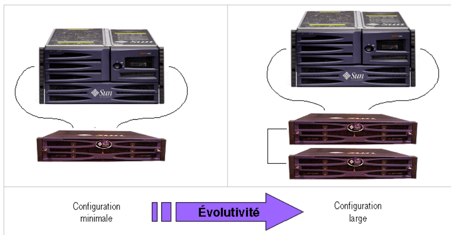
FIGURE 4 Architecture optimisée pour un serveur de messagerie
