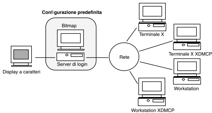
FIGURA 1-1 Possibile configurazione del server di login
