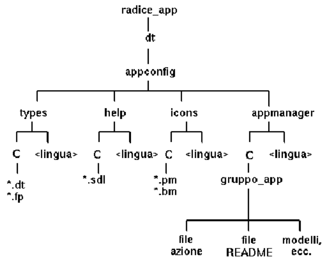
FIGURA 5-4 Pacchetto di registrazione nella directory radice di un'applicazione
