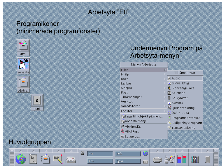
FIGUR 1-1 CDE-skrivbordet
