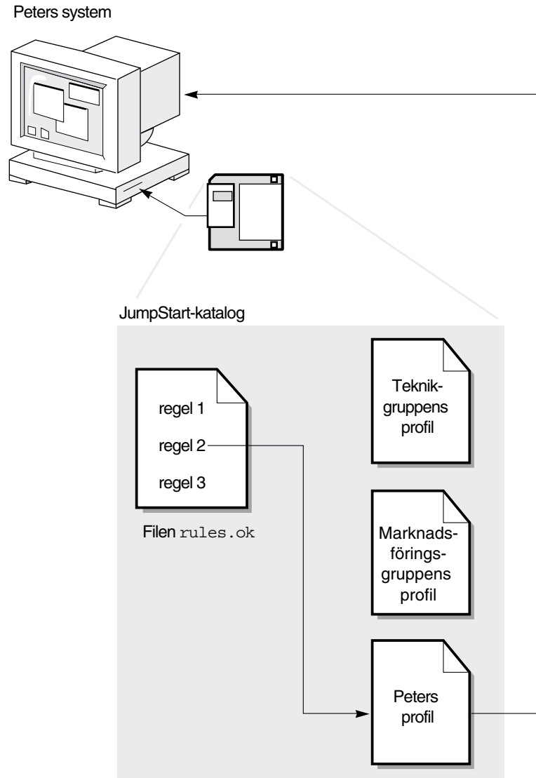
FIGUR 22-1 Så här fungerar en anpassad JumpStart-installation: exempel för ej nätverksanslutna system
