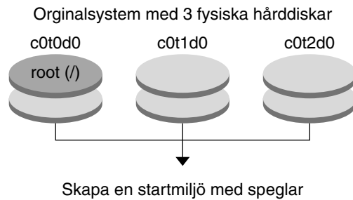
FIGUR 35-1 Koppla bort och uppgradera ena sidan av en RAID-1-volym (spegel) (fortsättning)
