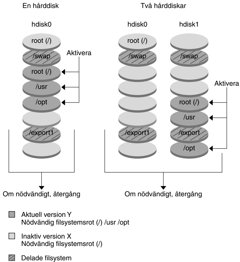
FIGUR 30–8 Aktivera en inaktiv startmiljö
