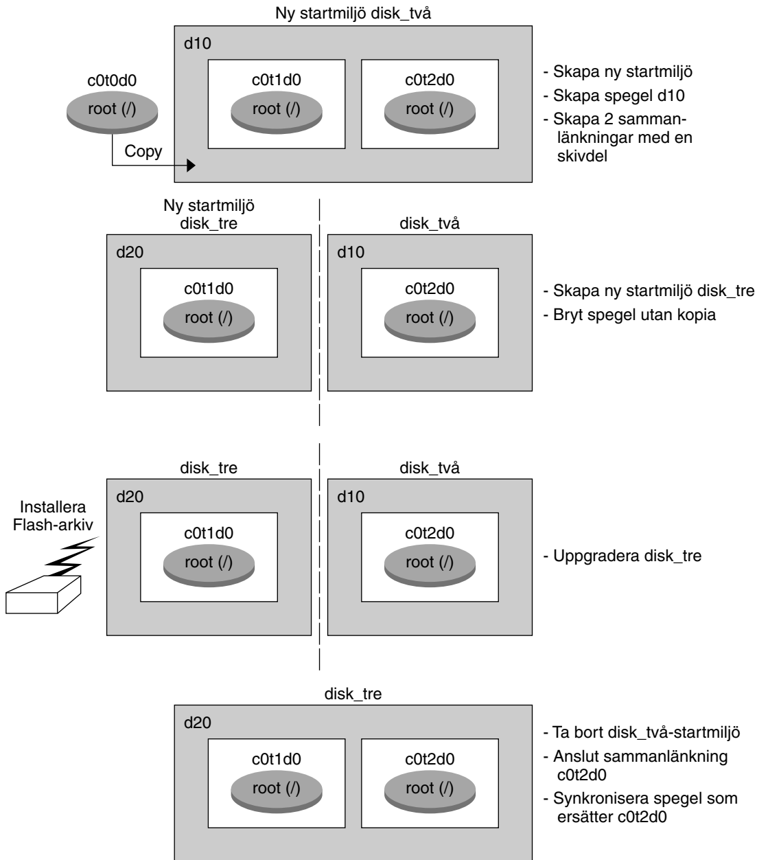
FIGUR 35-2 Koppla bort och uppgradera ena sidan av en RAID-1-volym (spegel) (fortsättning)
