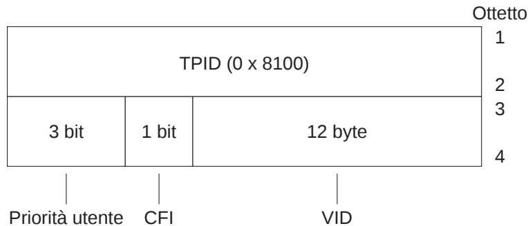
FIGURA 3-1 Formato Ethernet Tag Header
