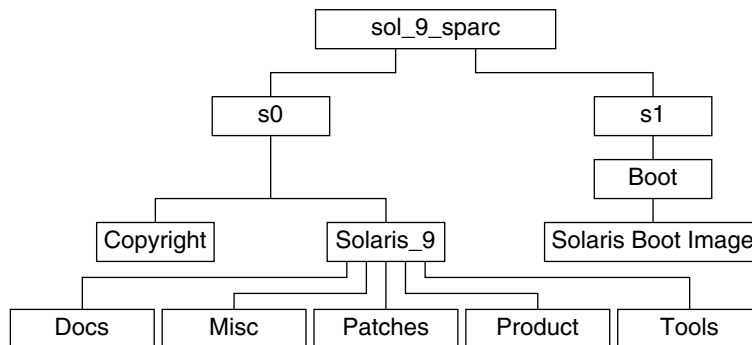
FIGUR B-3 SPARC: Solaris programvaru-cd 1 (av 2), SPARC-version
