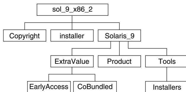
FIGUR B-9 Solaris programvaru-cd 2 (av 2), x86-version
