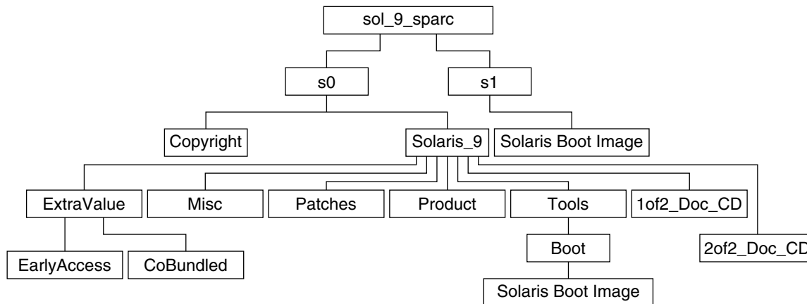
FIGUR B-1 Solaris-dvd (SPARC-version)
