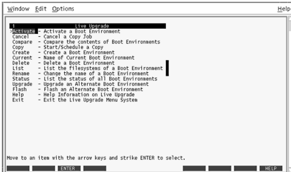
FIGUR 35-3 Huvudmenyn för Solaris Live Upgrade
