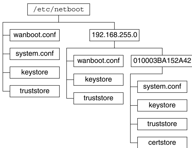
FIGUR 39-2 Exempel på katalogen /etc/netboot
