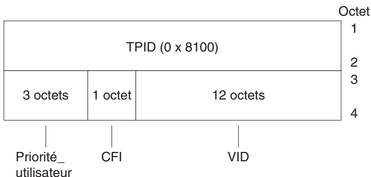
FIGURE 3-1 Format de l'en-tête de la trame Ethernet
