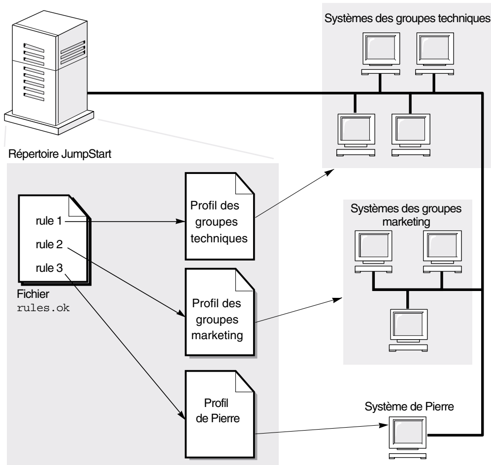
FIGURE 25-2 Fonctionnement d'une installation JumpStart personnalisée : exemple en réseau
