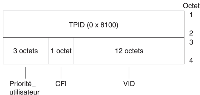
FIGURE 2-1 Format de l'en-tête de la trame Ethernet
