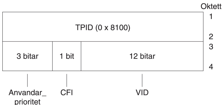
FIGUR 2-1 Ethernet-huvudmärkesformat
