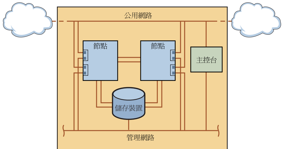
圖 1-1 叢集拓樸與纜線連接
