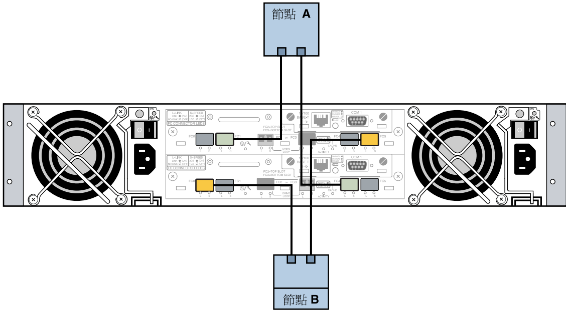
圖 1-3 Sun StorEdge 3510 FC RAID 陣列連接到兩個節點
