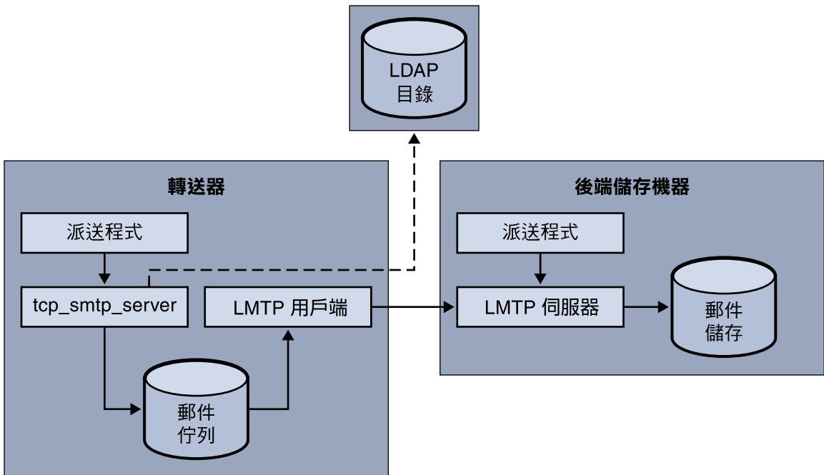
圖 15-2 帶有 LMTP 的兩層部署
