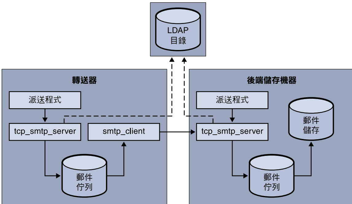
圖 15-1 不使用 LMTP 的兩層部署
