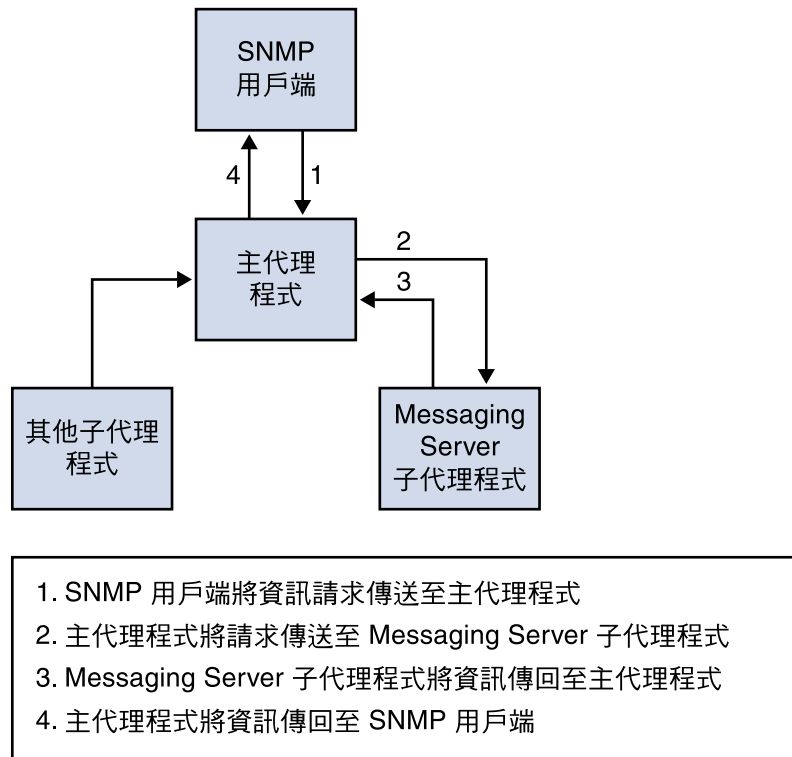
圖 A-1 SNMP 資訊流程
