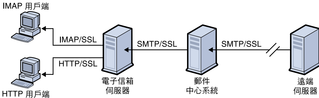
圖 19-1 與 Messaging Server 進行加密通訊
