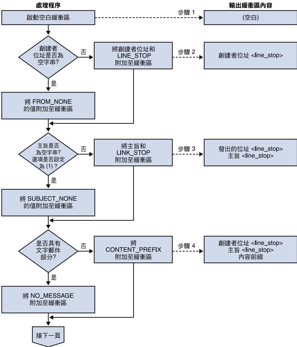
圖 D-2 SMS 通道電子郵件處理
