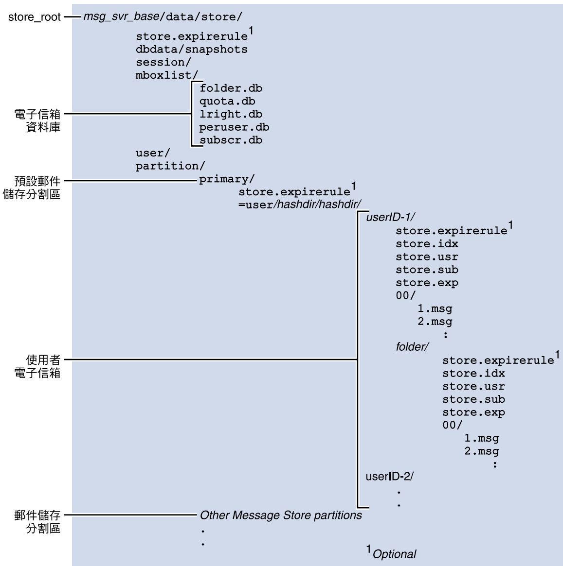
圖 18-1 郵件儲存目錄配置
