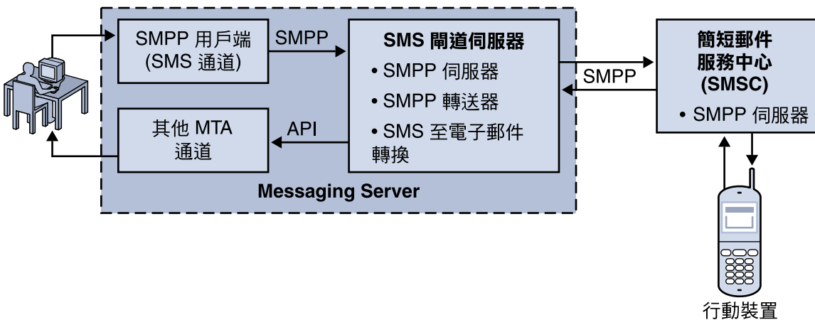
圖 D-1 單向與雙向 SMS 的邏輯流程
