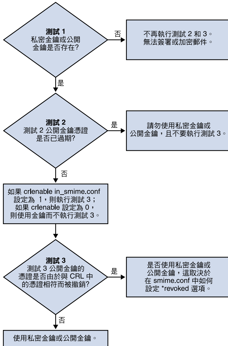
圖 20-2 驗證私密金鑰和公開金鑰
